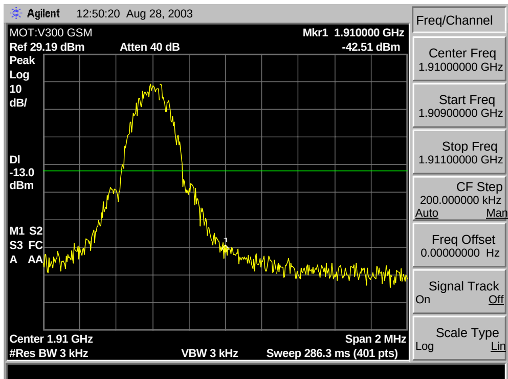
GSM 1900 C, C1 Max Block Edge
