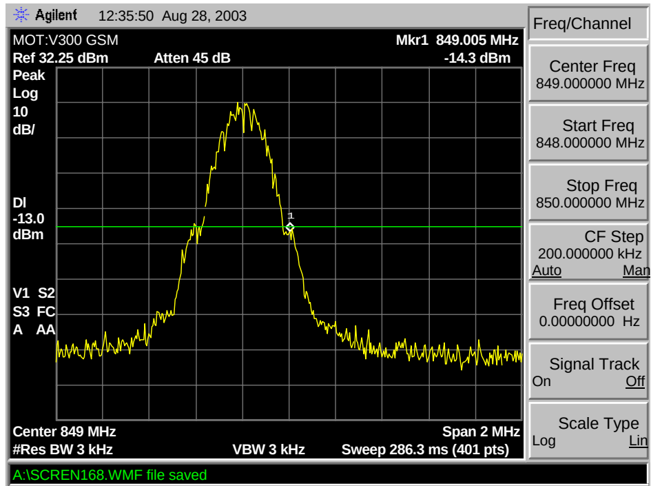
GSM 850 B* Max Block Edge
