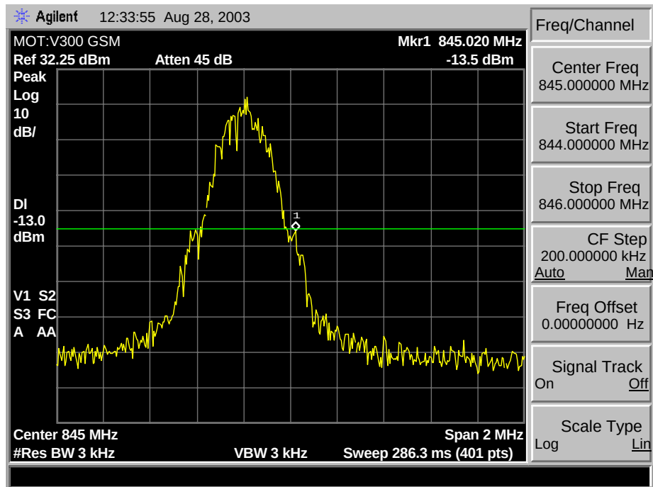
GSM 850 B Max Block Edge
