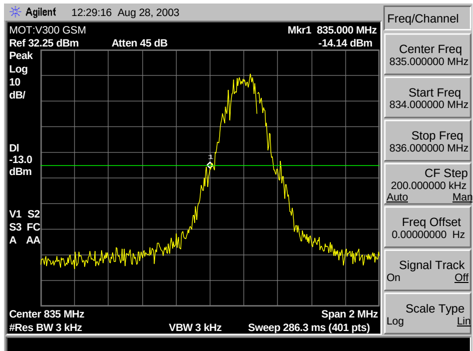
GSM 850 B Min. Block Edge
