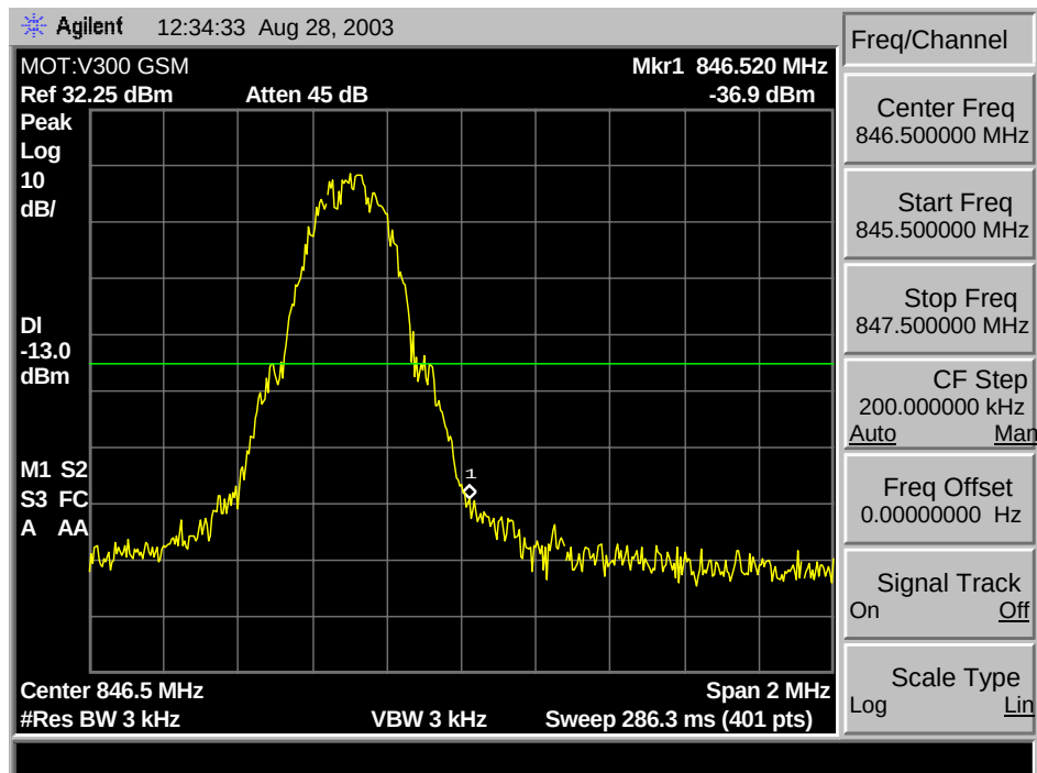
GSM 850 A*(Upper) Max Block Edge
