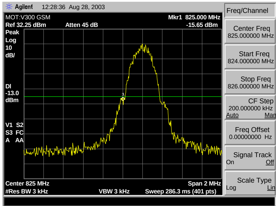
GSM 850 A Min. Block Edge
