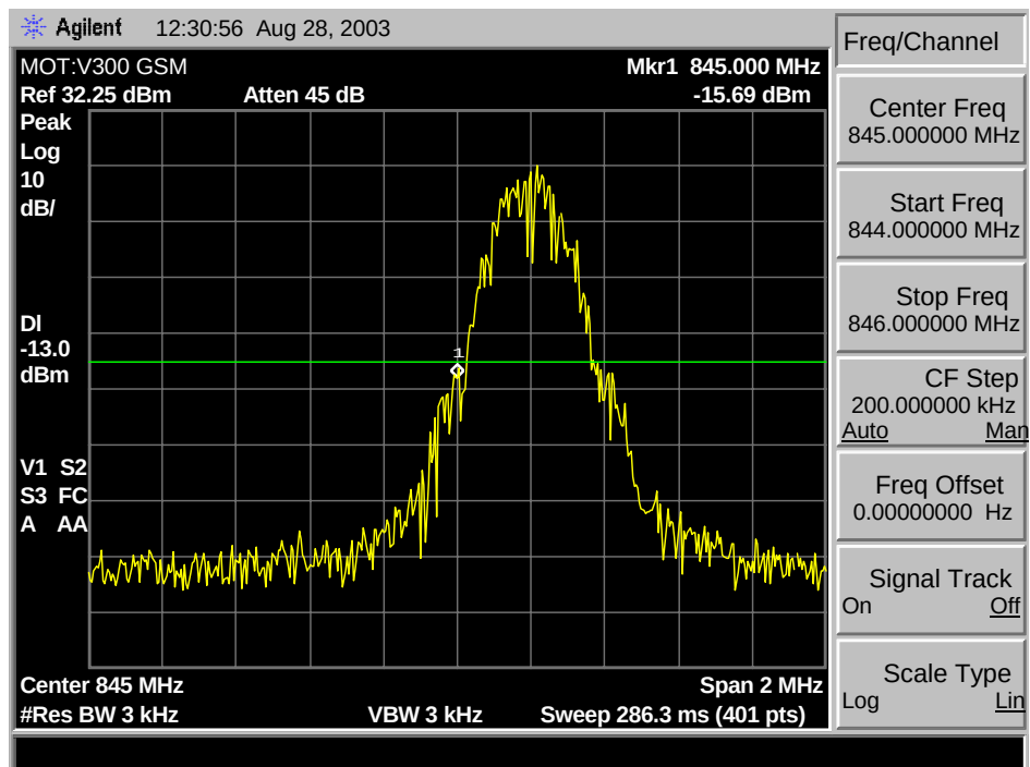
GSM 850 BLK A*(Upper) Min. Block Edge
