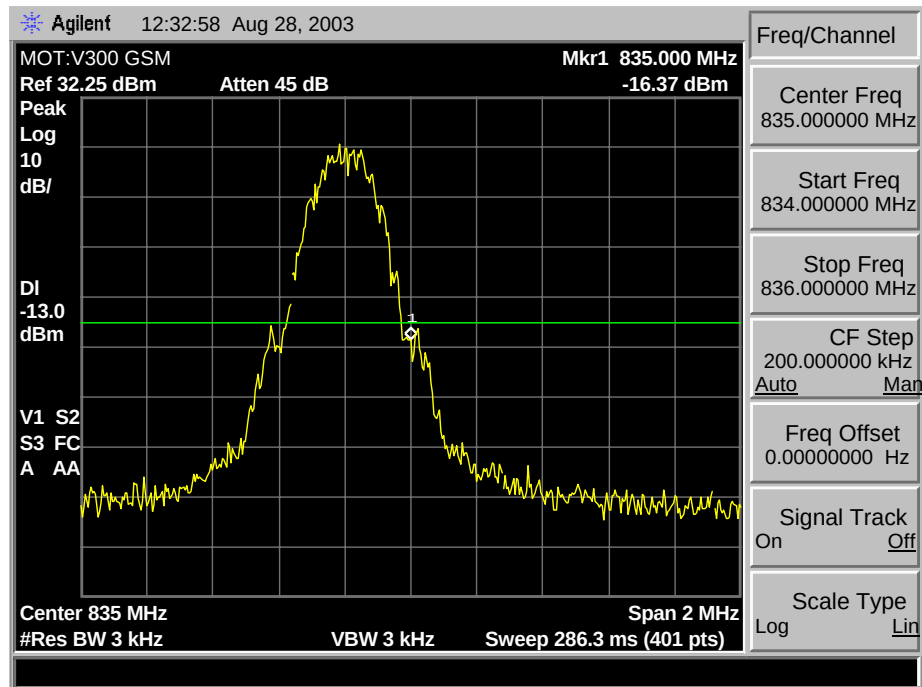
GSM 850 A Max Block Edge
