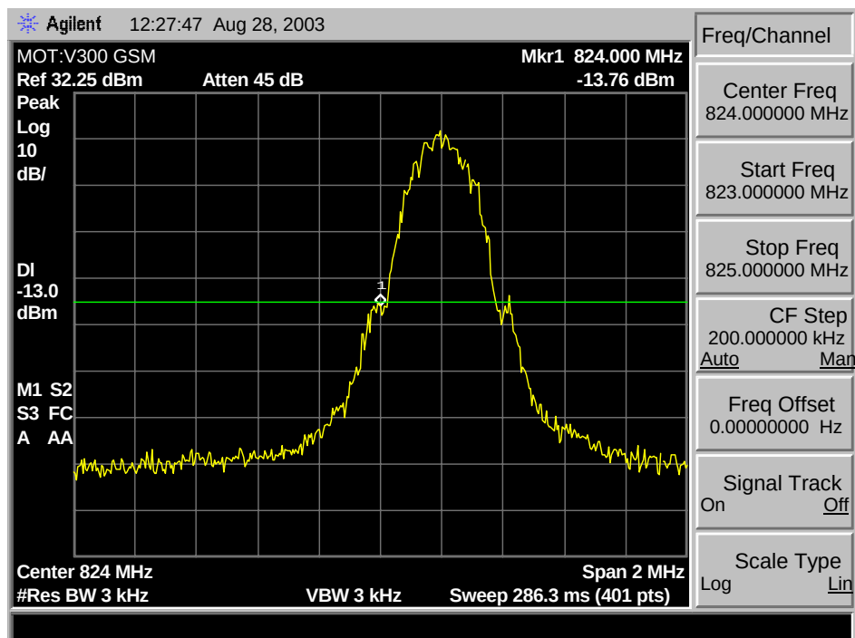
GSM 850 A*(Lower) Min. Block Edge
