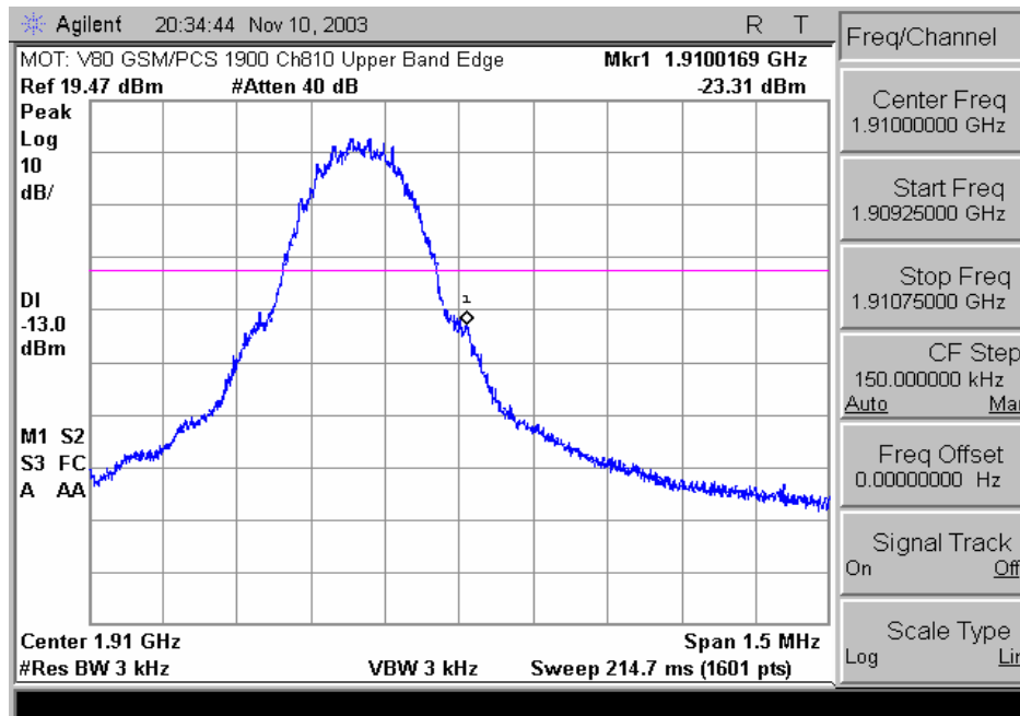
1900 GSM Upper Band Edge
