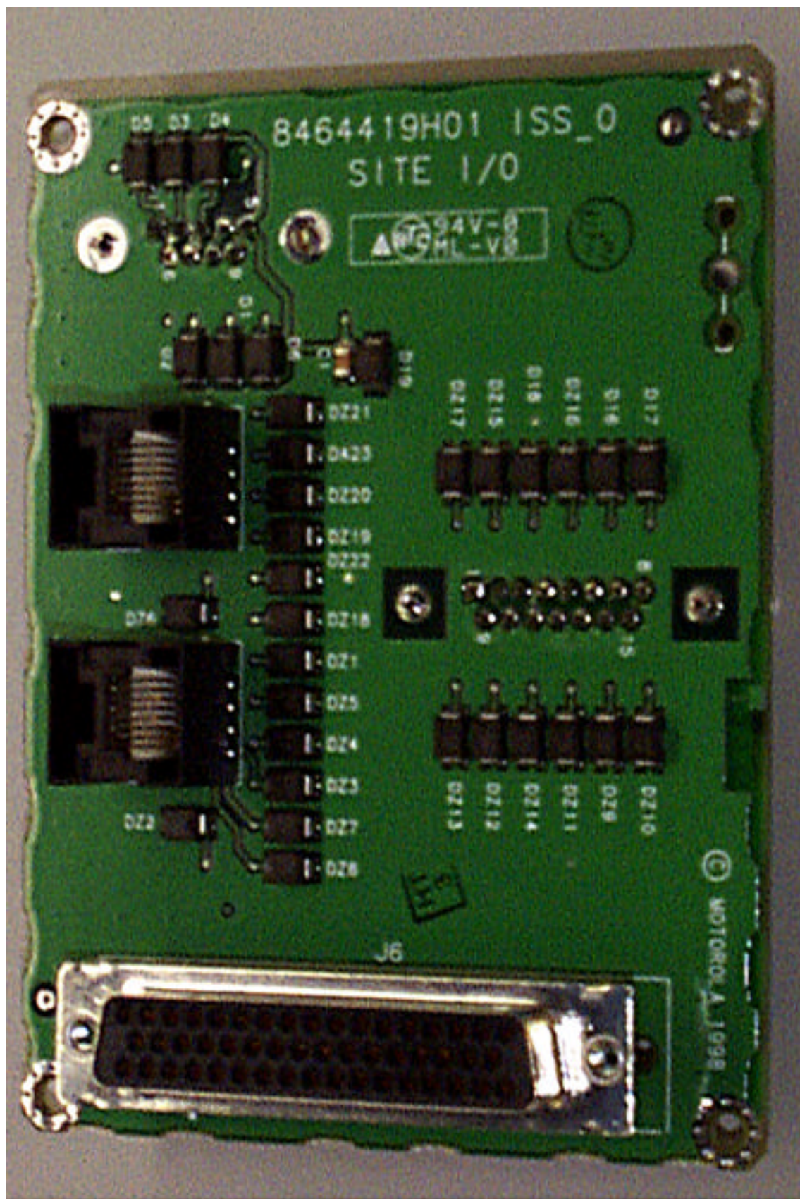
IHET5YP1 SC4812T 800 MHz Site I/O Back
