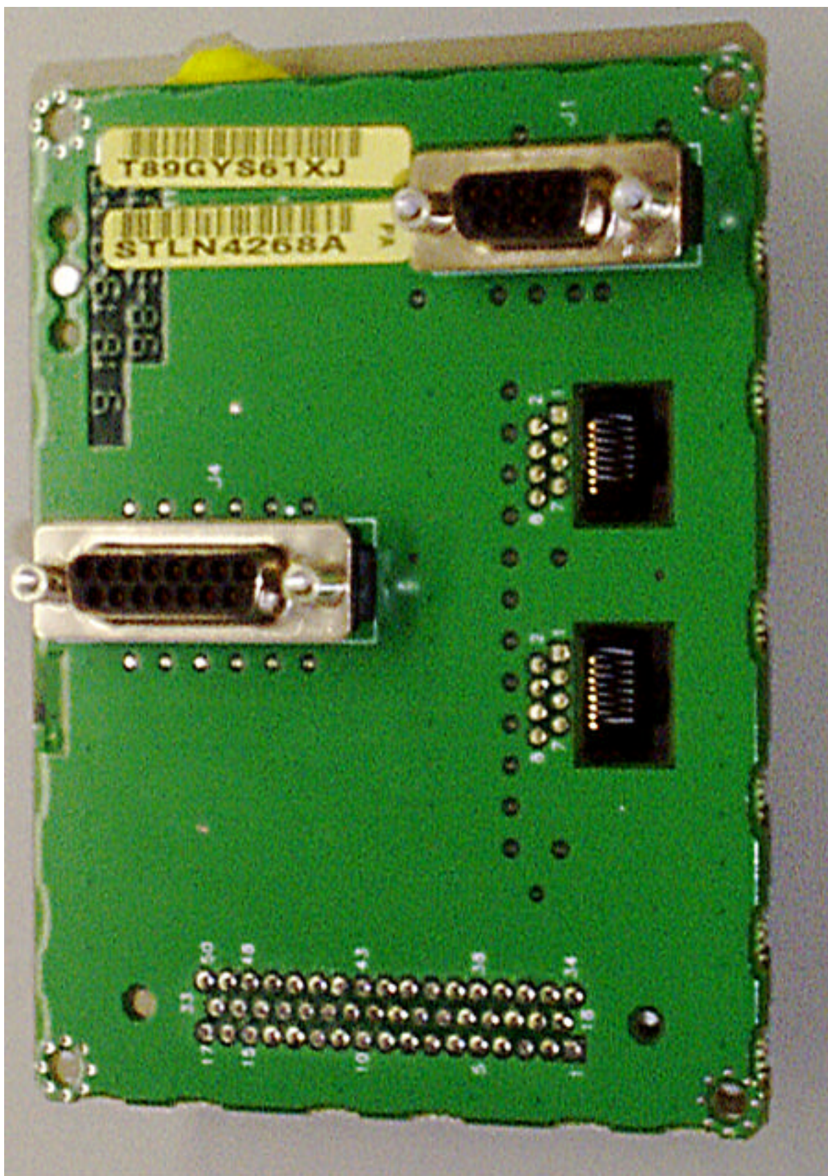
IHET5YP1 SC4812T 800 MHz Site I/O Front
