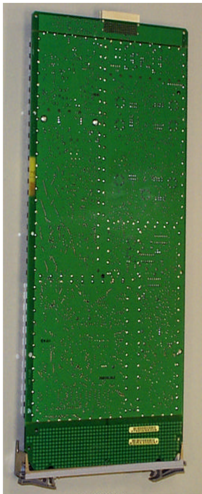
IHET5YP1 SC4812T 800 MHz LFR Back
