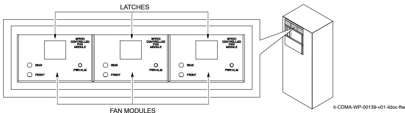
Figure 3-27: Fan Modules
