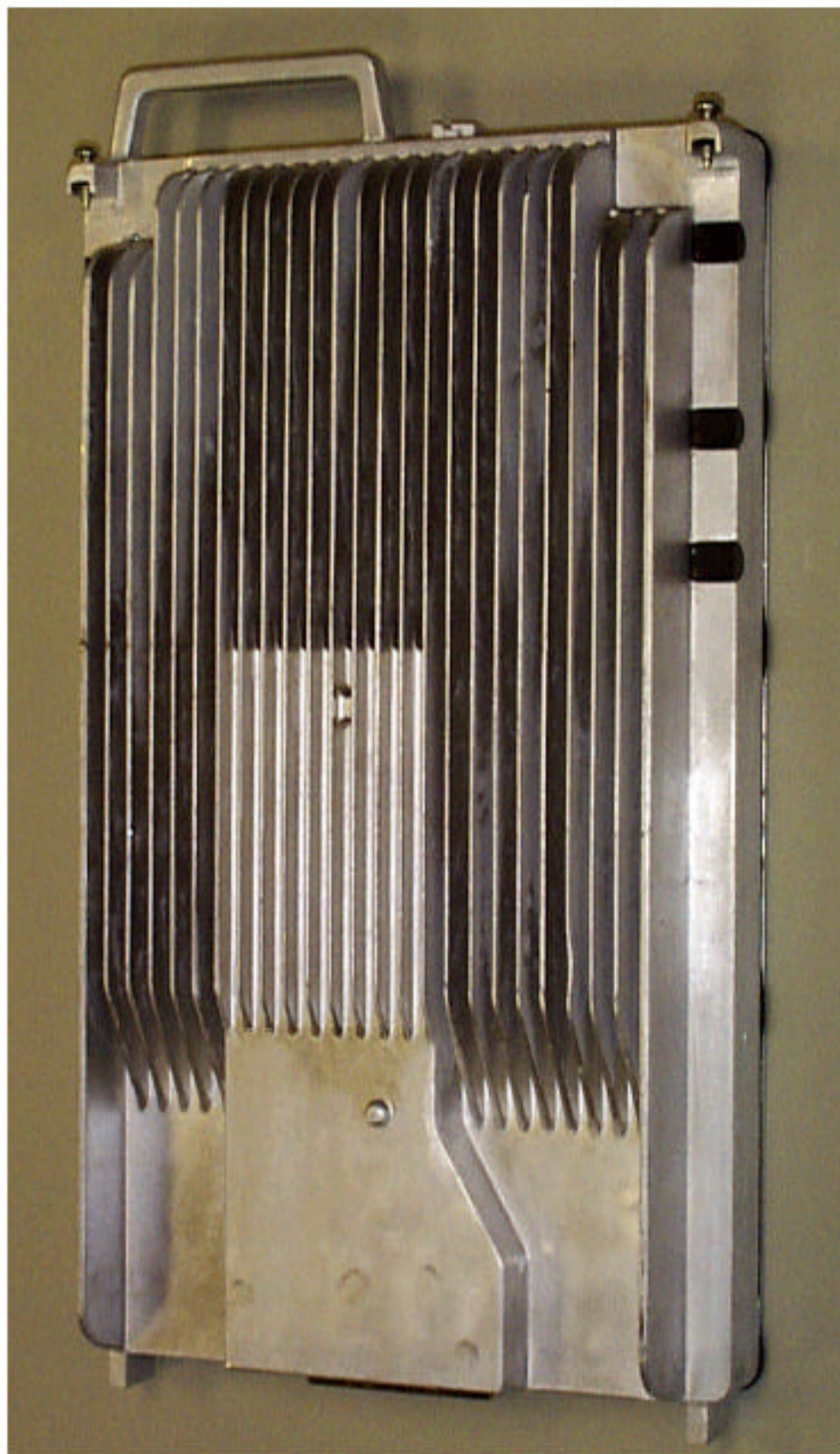
IHET6YZ1 SC4812ET 1.9 GHz LPA Front
