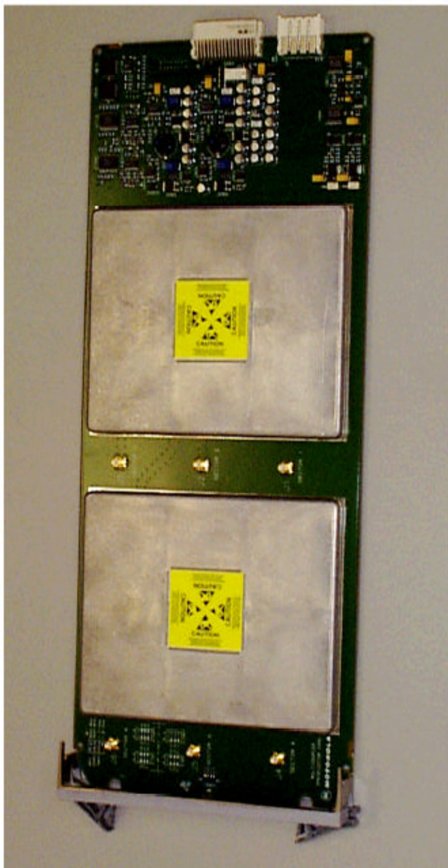
IHET6YZ1 SC4812ET 1.9 GHz MPC Front
