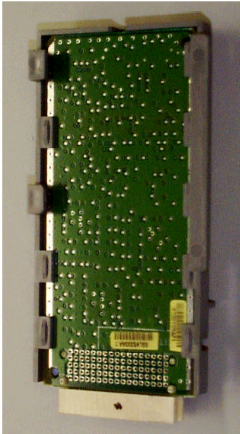
IHET6YZ1 SC4812ET 1.9 GHz CCD Back
