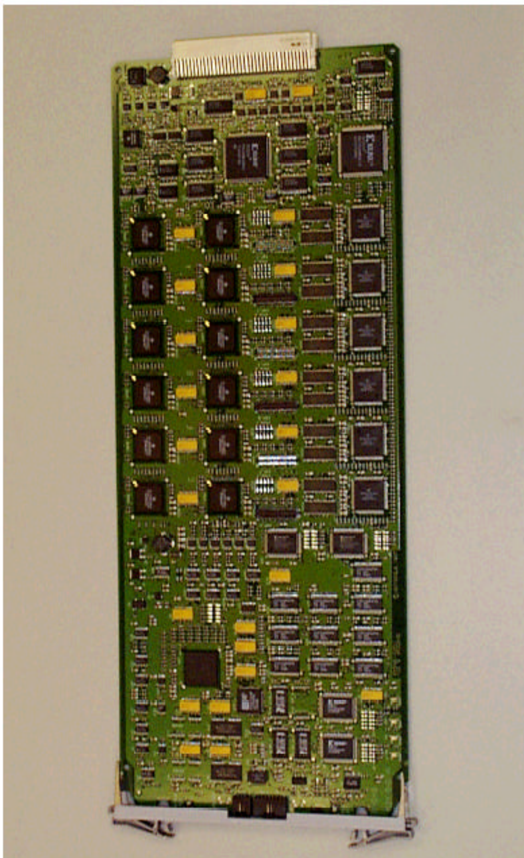
IHET6YZ1 SC4812ET 1.9 GHz MCC x 24E Front
