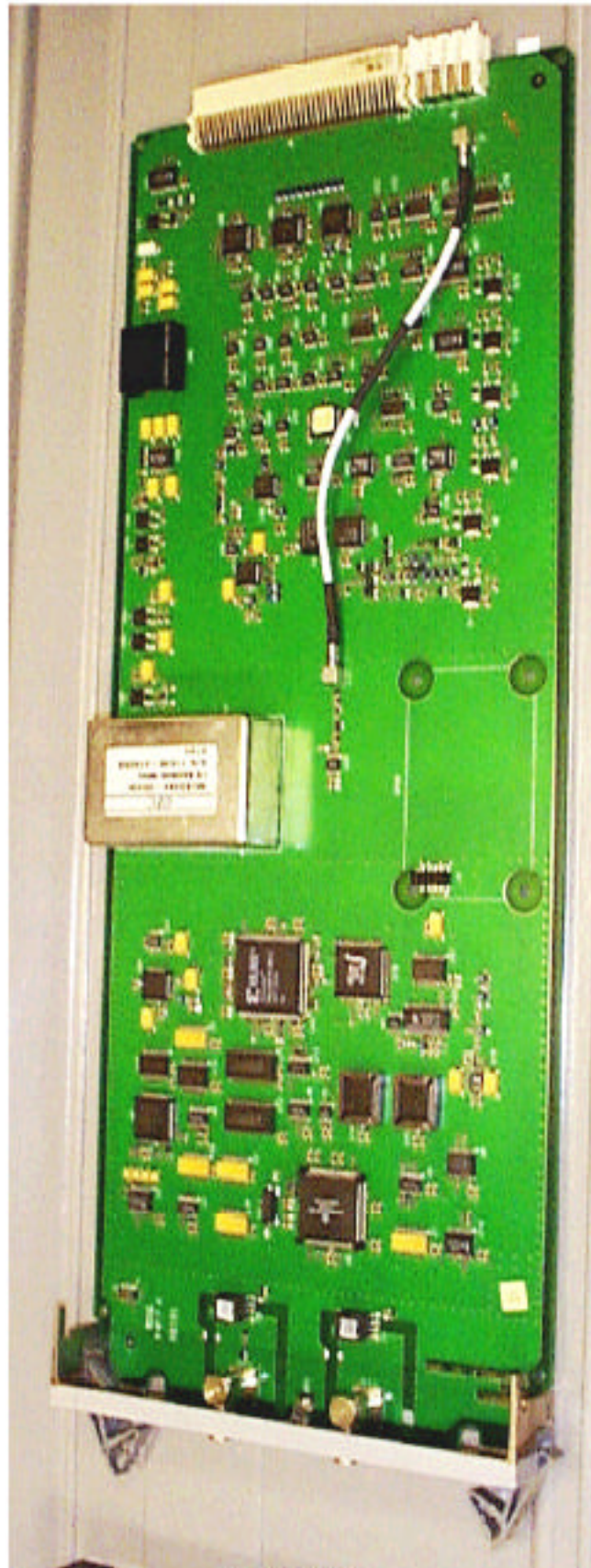
IHET6YZ1 SC4812ET 1.9 GHz CSM2 Front
