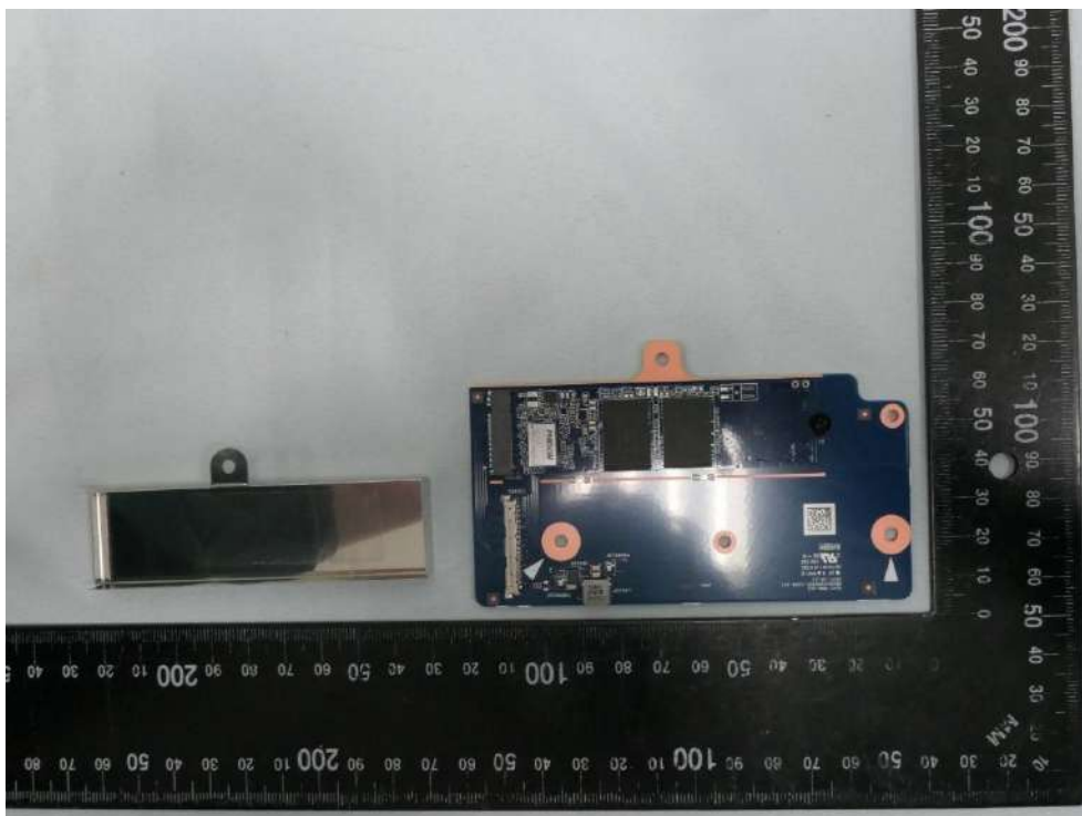
(40) EUT Photo
