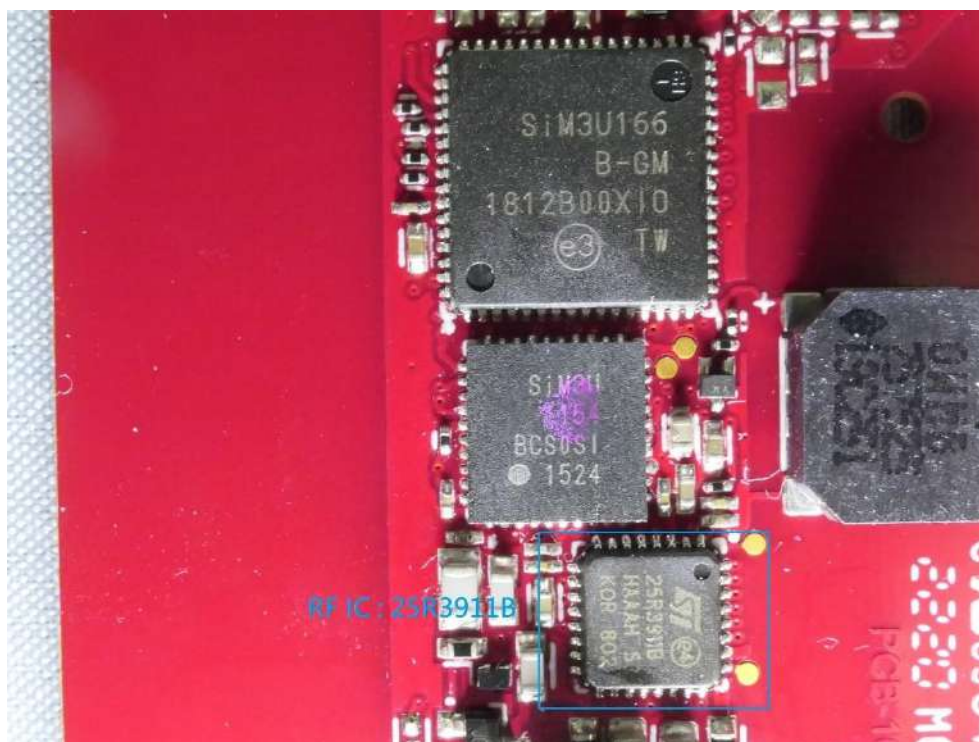
(52) EUT Photo
