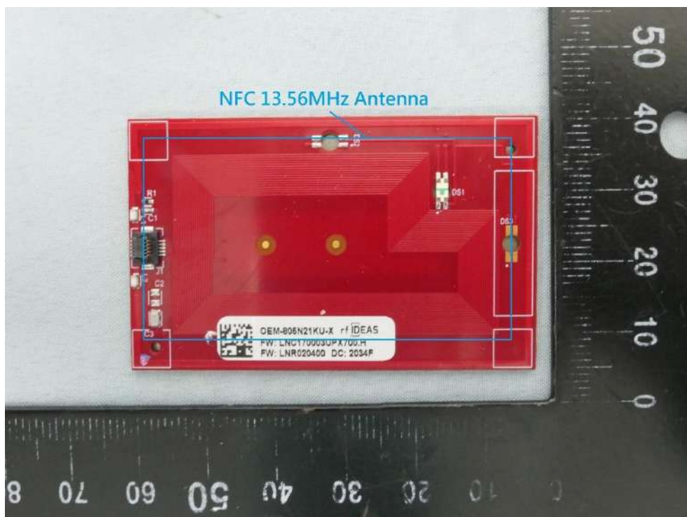
(50) EUT Photo
