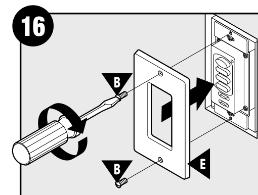
Replace the switch plate and restore power./ Coloque de nuevo la placa del interruptor y restablezca la alimentación eléctrica.
