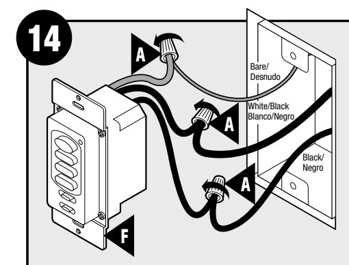
Connect wires as shown./ Conecte los alambres como se muestra.
