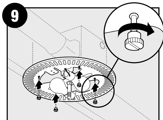
Attach thumbscrews. WARNING: To reduce the risk of electrical shock, all 4 thumbscrews MUST be properly installed./Coloque y apriete los tornillos de mano. ADVERTENCIA: Para reducir el riesgo de descargas eléctricas, los 4 tornillos de mano SE DEBEN instalar correctamente.
