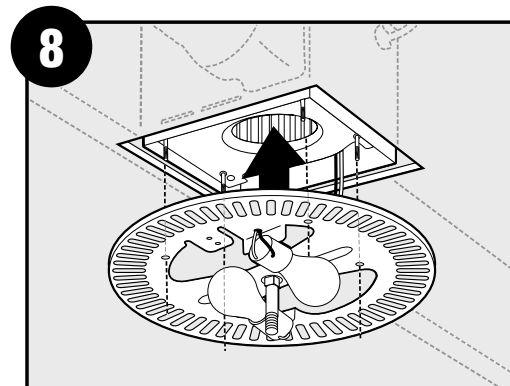
Slide light mount over posts. (Models vary – For details see bath fan owner's manual.)/Deslice el soporte de la luz por los postes. (Los modelos varían. Para obtener detalles, consulte el manual del usuario del ventilador de baño.)
