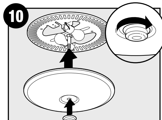
Replace the dome./Coloque de nuevo la cúpula.
