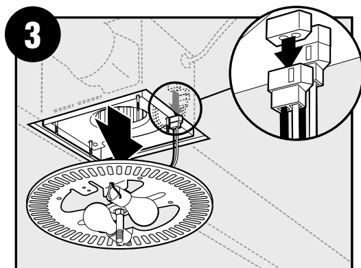
Unplug the light mount./Desenchufe el soporte de la luz.
