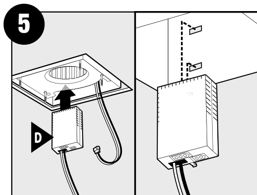
Snap the receiver into place between the motor and the housing./Encaje el receptor en su sitio entre el motor y la caja.
