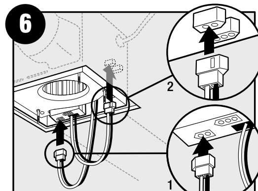
Plug motor wiring into the receiver and receiver wiring into the wiring cover plate./Enchufe los cables del motor en el receptor y los cables del receptor en la placa de cubierta de los cables.
