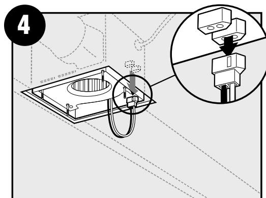
Unplug the motor from the wiring cover plate./ Desenchufe el motor de la placa de cubierta de los cables.
