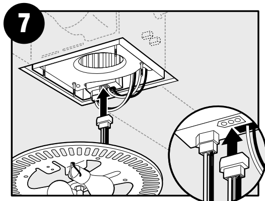
Plug the light mount into the receiver./ Enchufe el soporte de la luz en el receptor.
