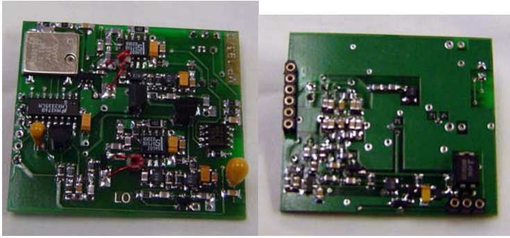
PLL VCO TXCO PCB TOP & BOTTOM
