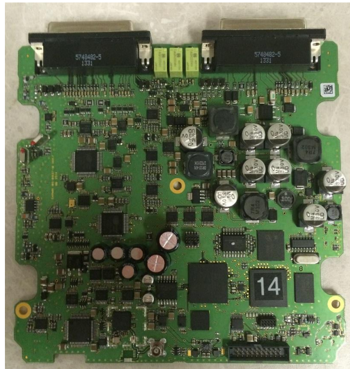
Top Side
