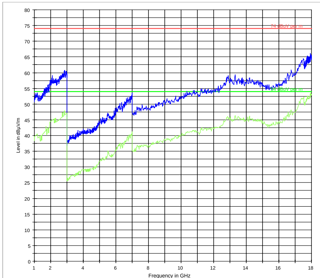
FCC 15 1-18GHz
