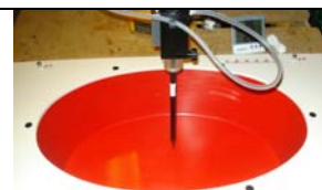
ELI Planar Phantom
