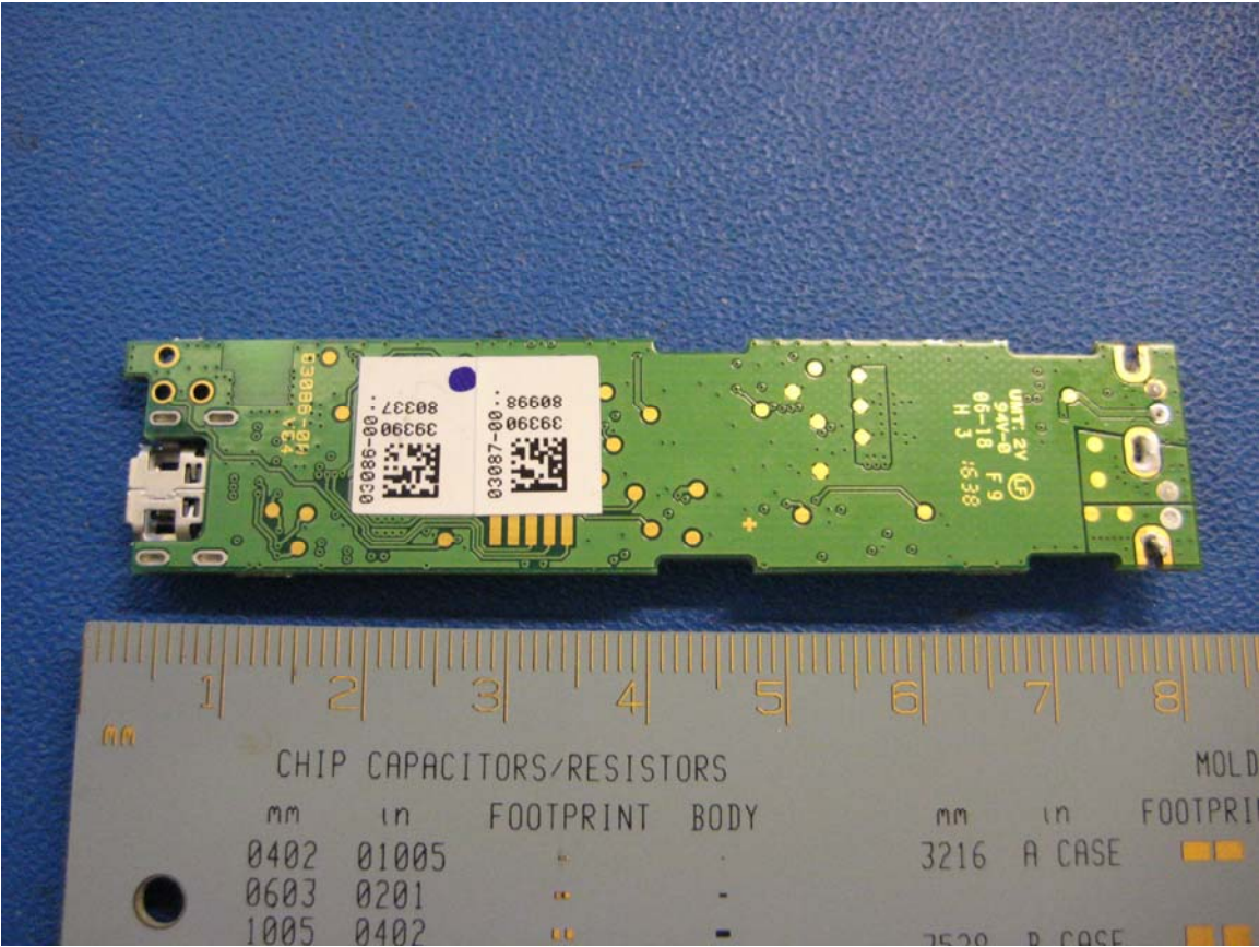
PCB Bottom
