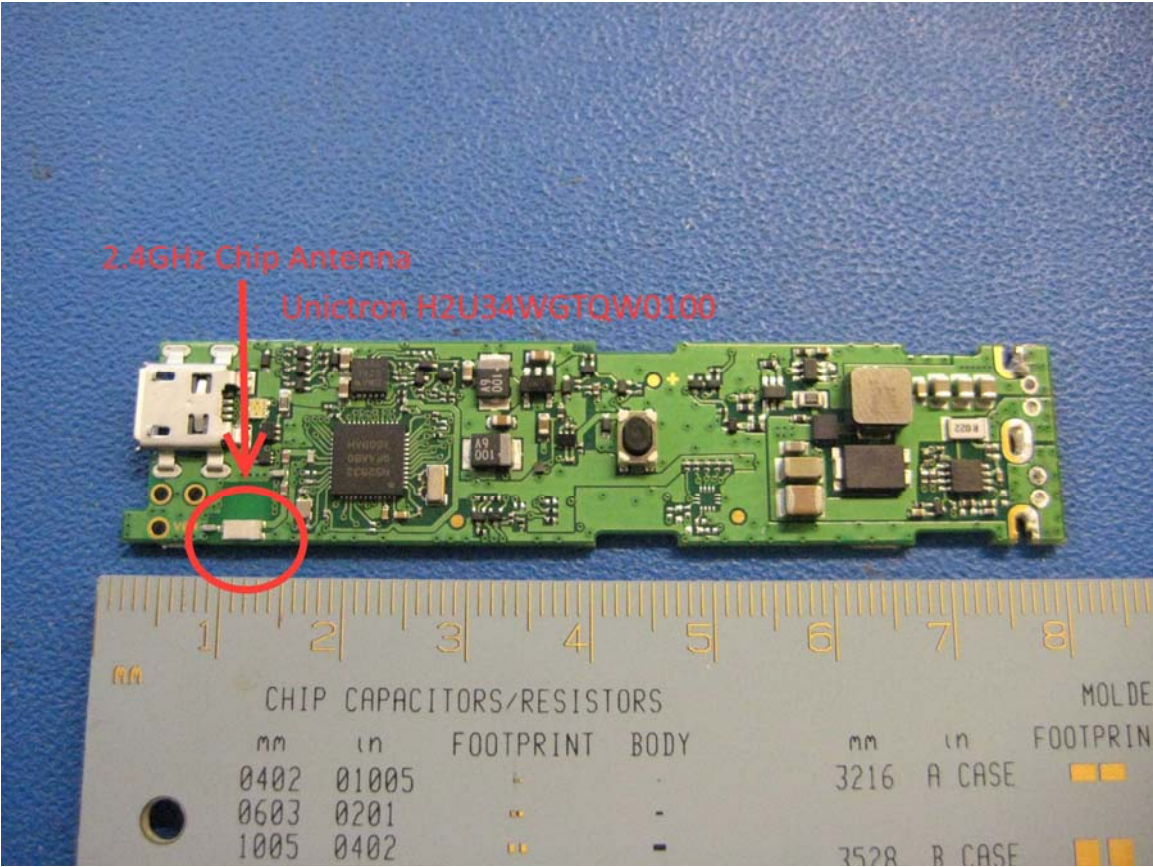
PCB Top
