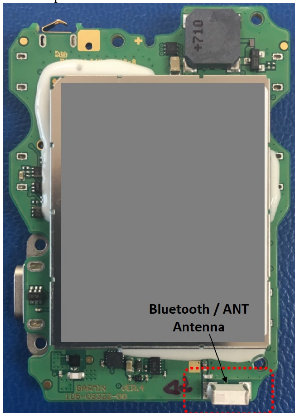
PCB bottom
