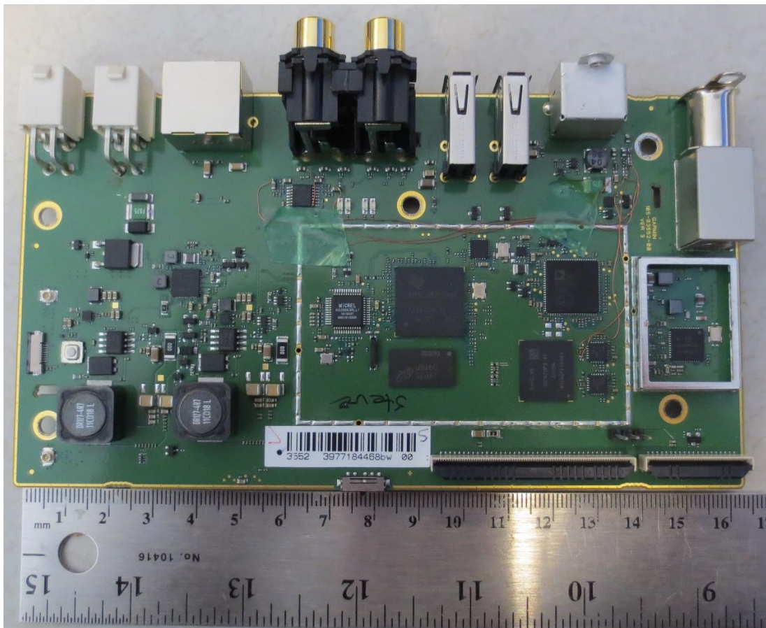
012-03552-00 L Board
