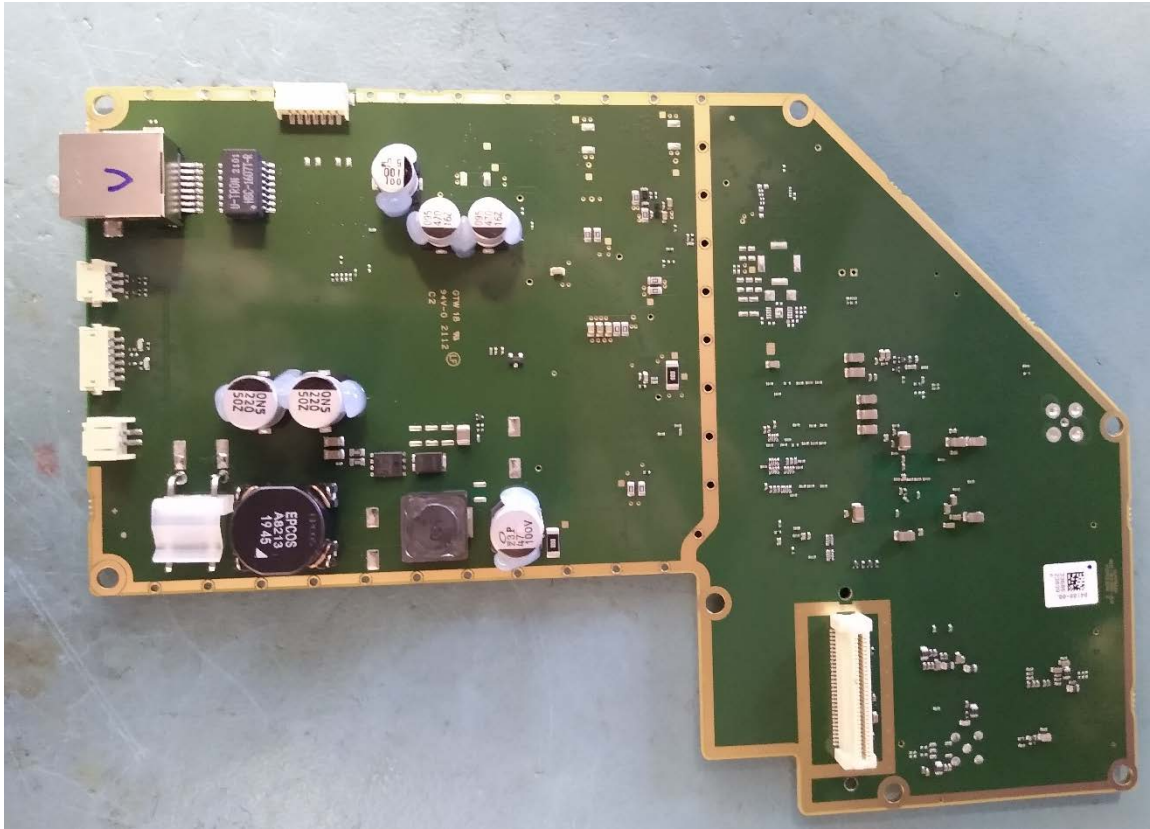
PCB1 – Side 1
