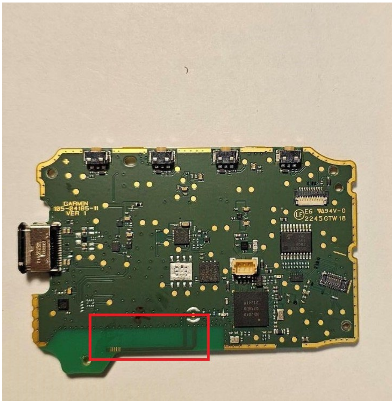
2.4 GHz Antenna
