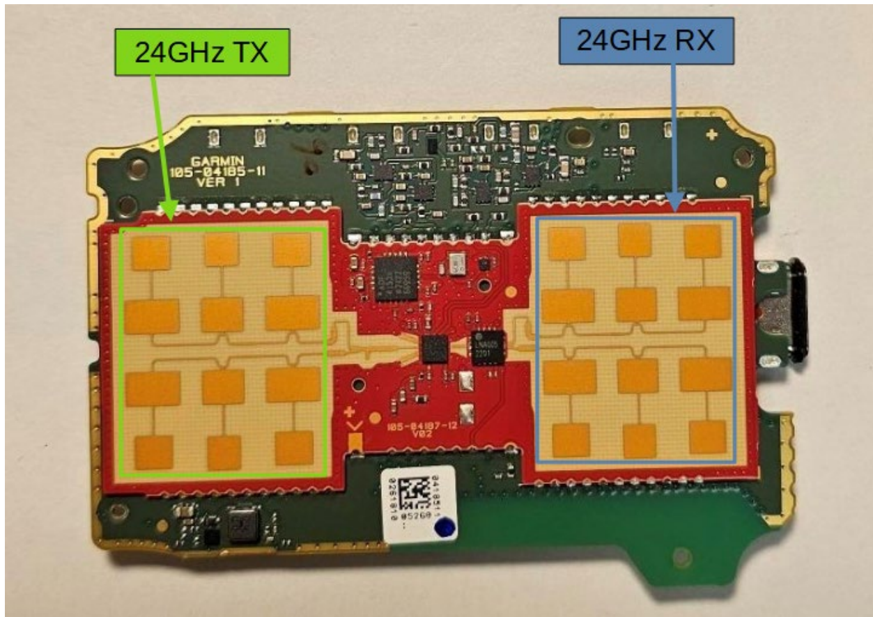
24 GHz Antenna
