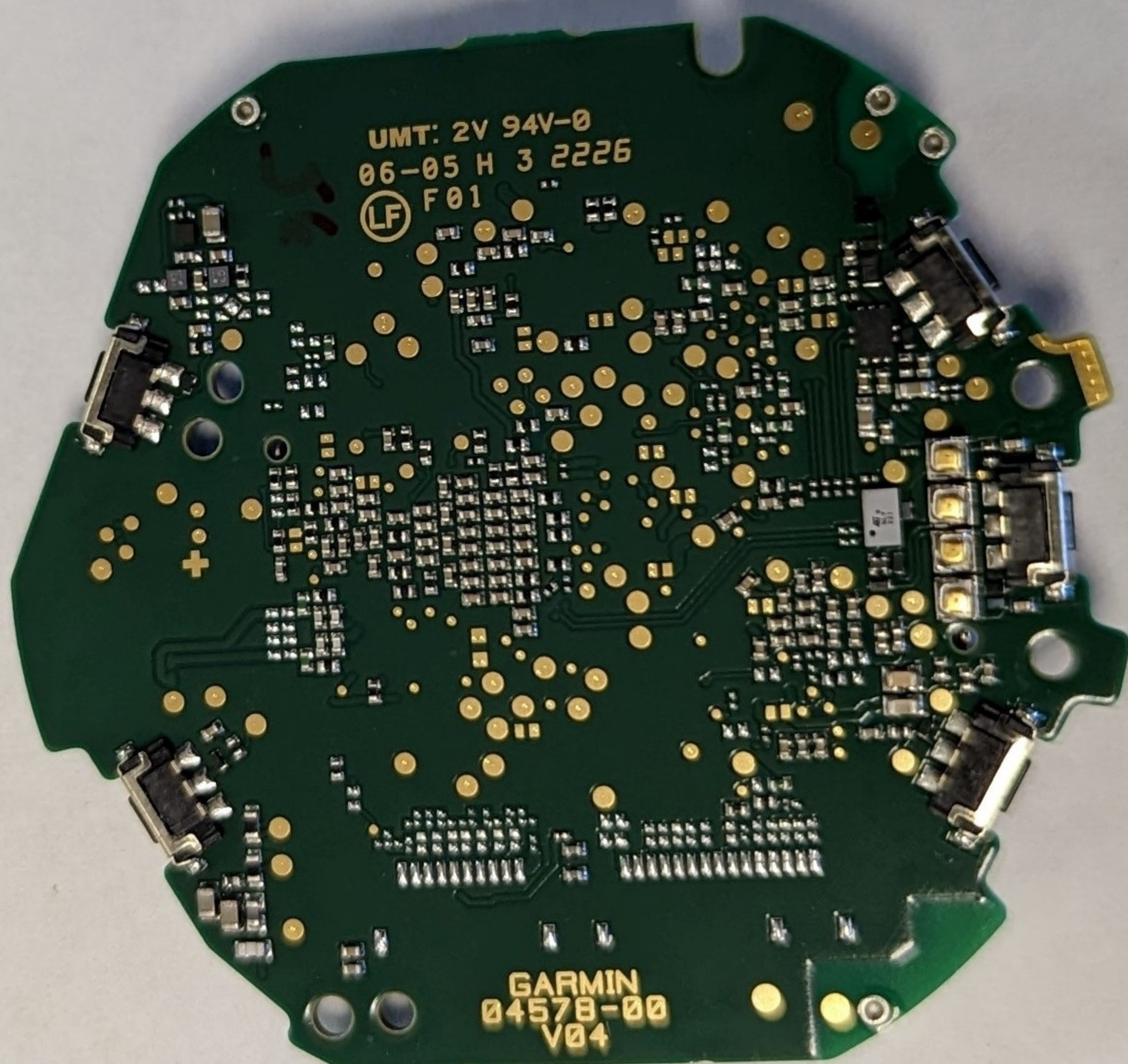
2.4GHz Antenna (Metal bezel)
