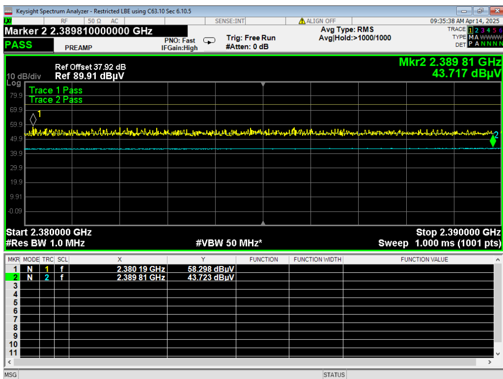
12 LBE Restricted, BLE 1MB, 2402MHz
