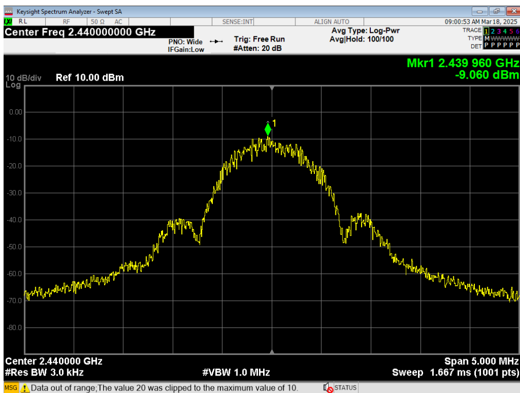
08 PSD, BLE 1MB, 2440MHz
