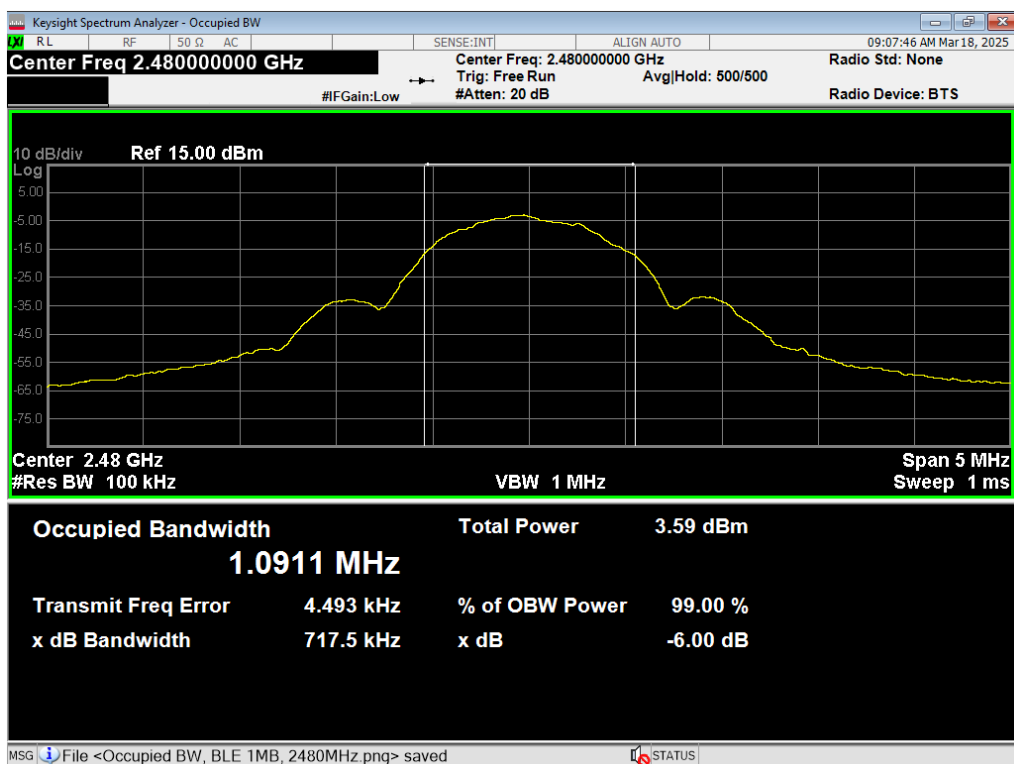
06 6dB BW, BLE 1MB, 2480MHz
