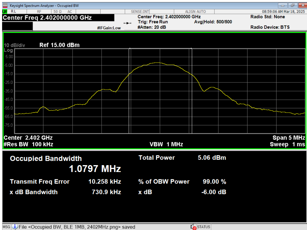
04 6dB BW, BLE 1MB, 2402MHz
