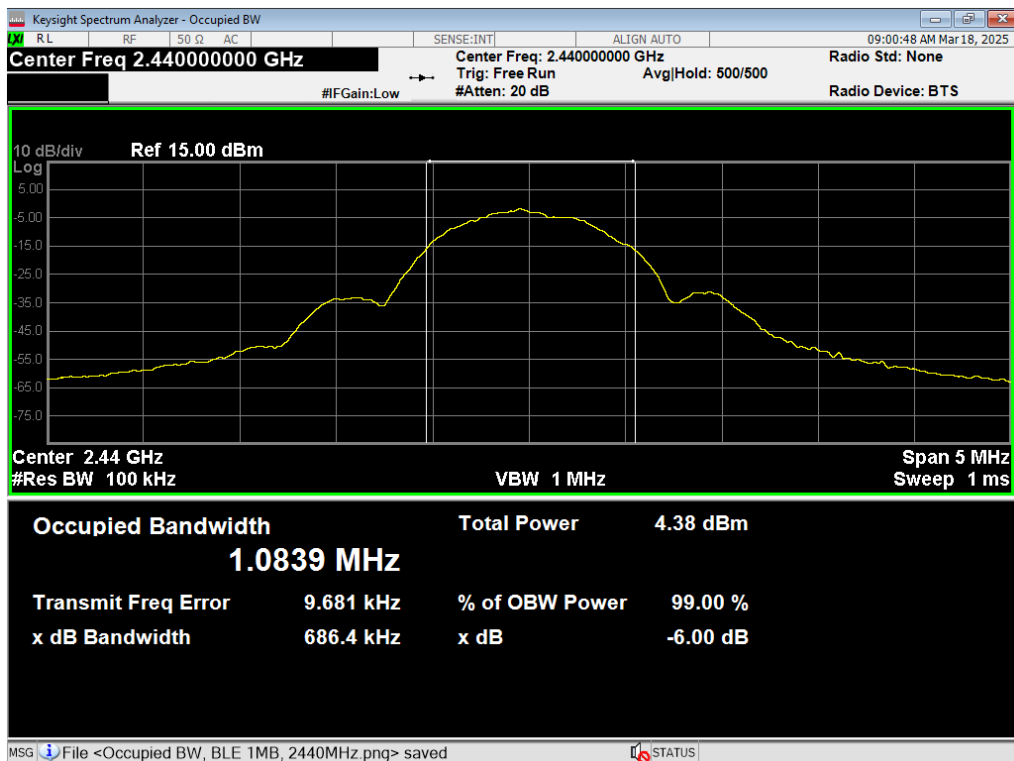
05 6dB BW, BLE 1MB, 2440MHz
