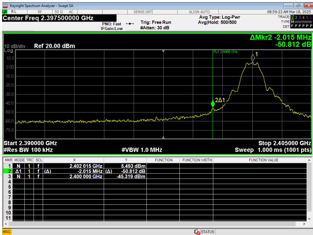
10 LBE Unrestricted, BLE 1MB
