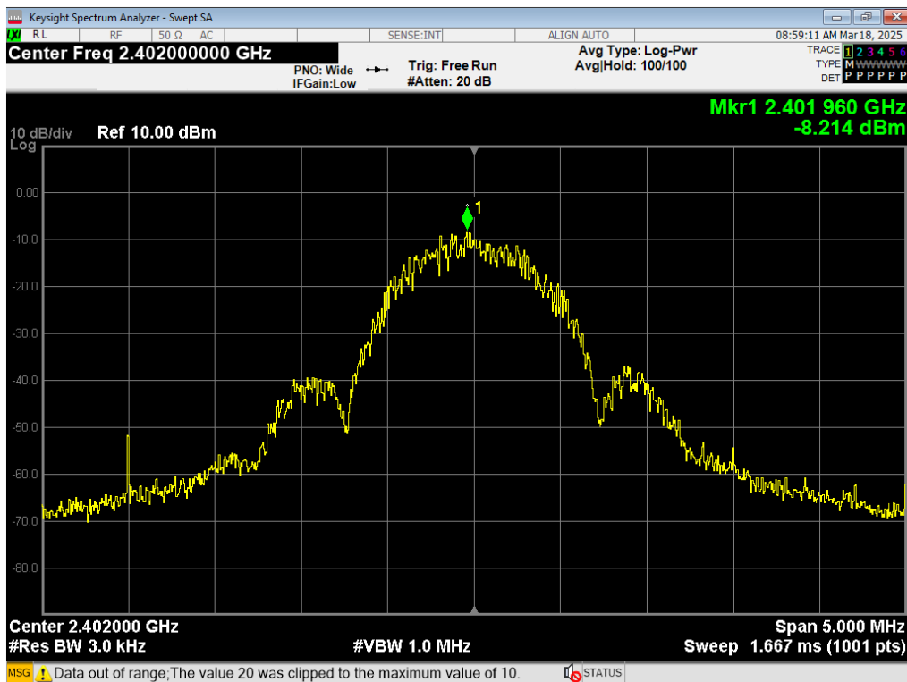
07 PSD, BLE 1MB, 2402MHz
