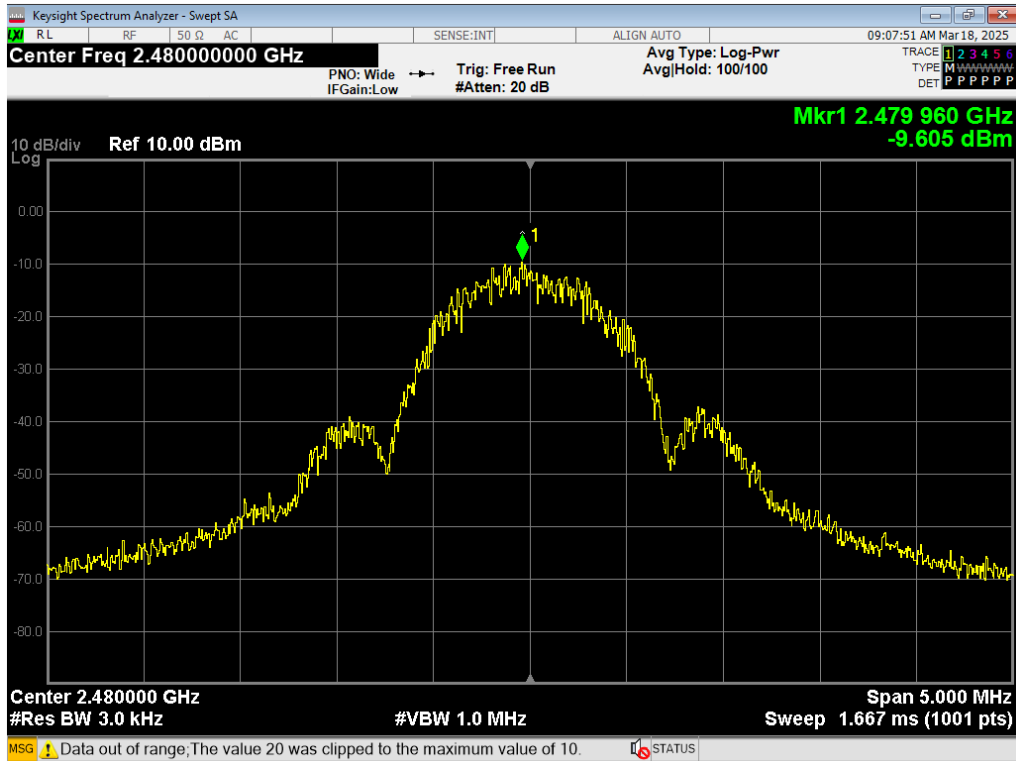
09 PSD, BLE 1MB, 2480MHz
