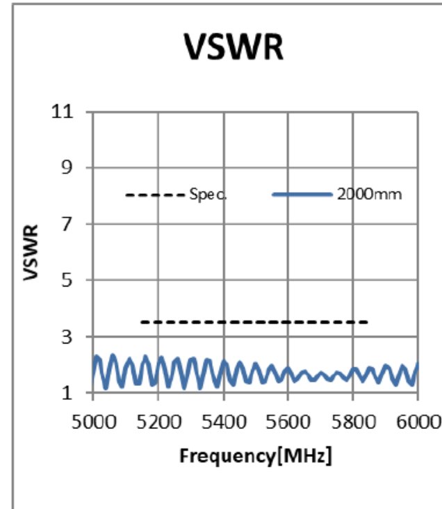
5GHz (5150~5850MHz)
