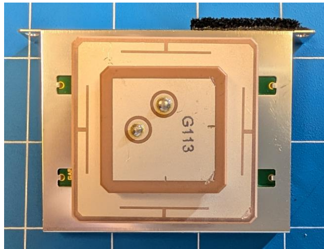
x04946 GPS/GNSS Module Front
