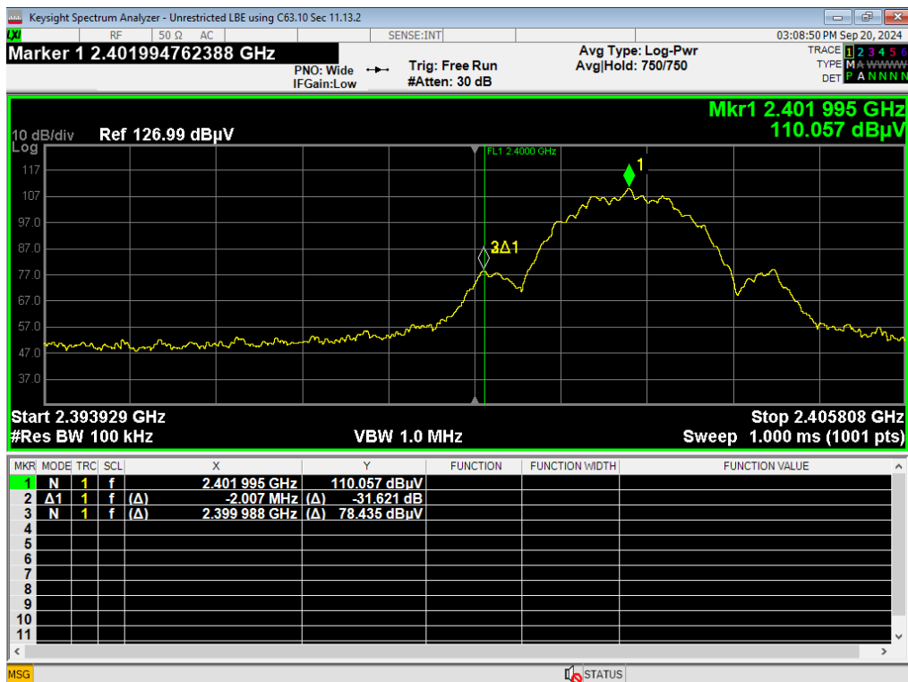
29 LBE Unrestricted, BLE 2MB
