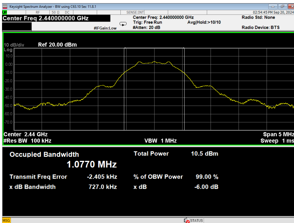
08 6dB BW, BLE 1MB, Mid
