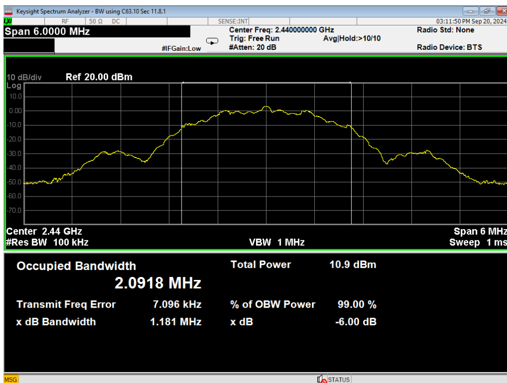
24 6dB BW, BLE 2MB, Mid
