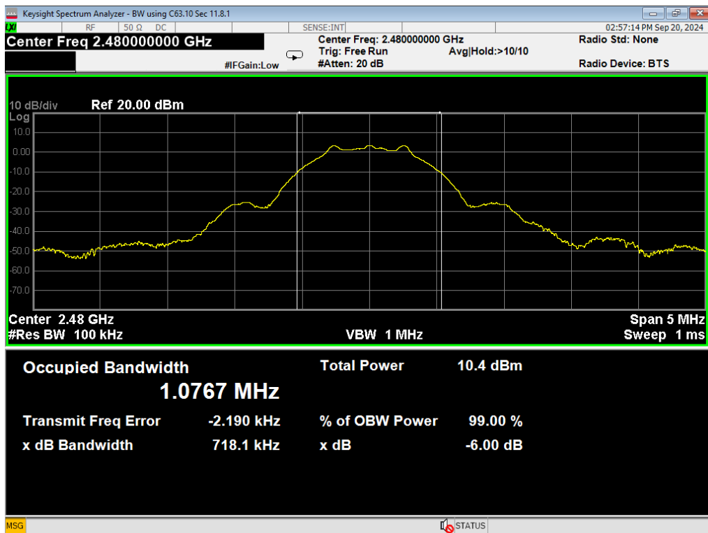
09 6dB BW, BLE 1MB, High
