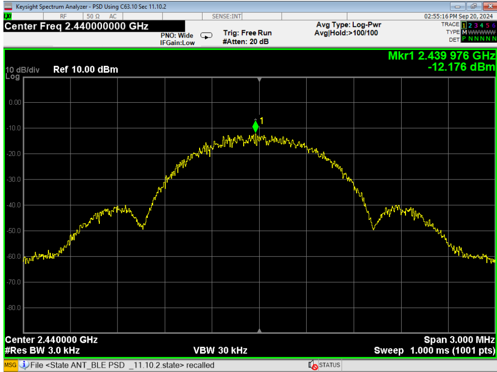
11 PSD, BLE 1MB, Mid
