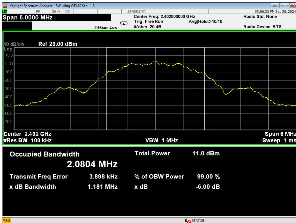
23 6dB BW, BLE 2MB, Low
