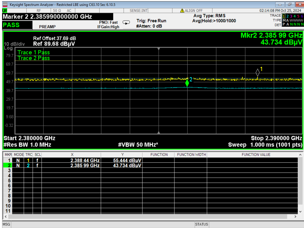
15 LBE Restricted, BLE 1MB
