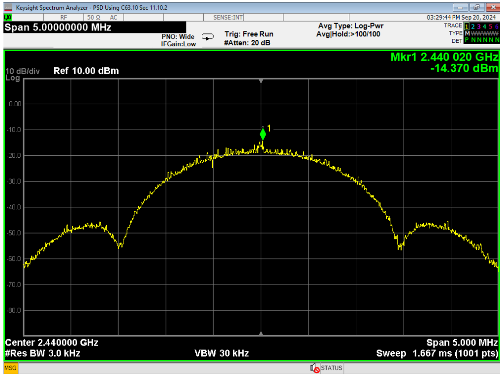
27 PSD, BLE 2MB, Mid
