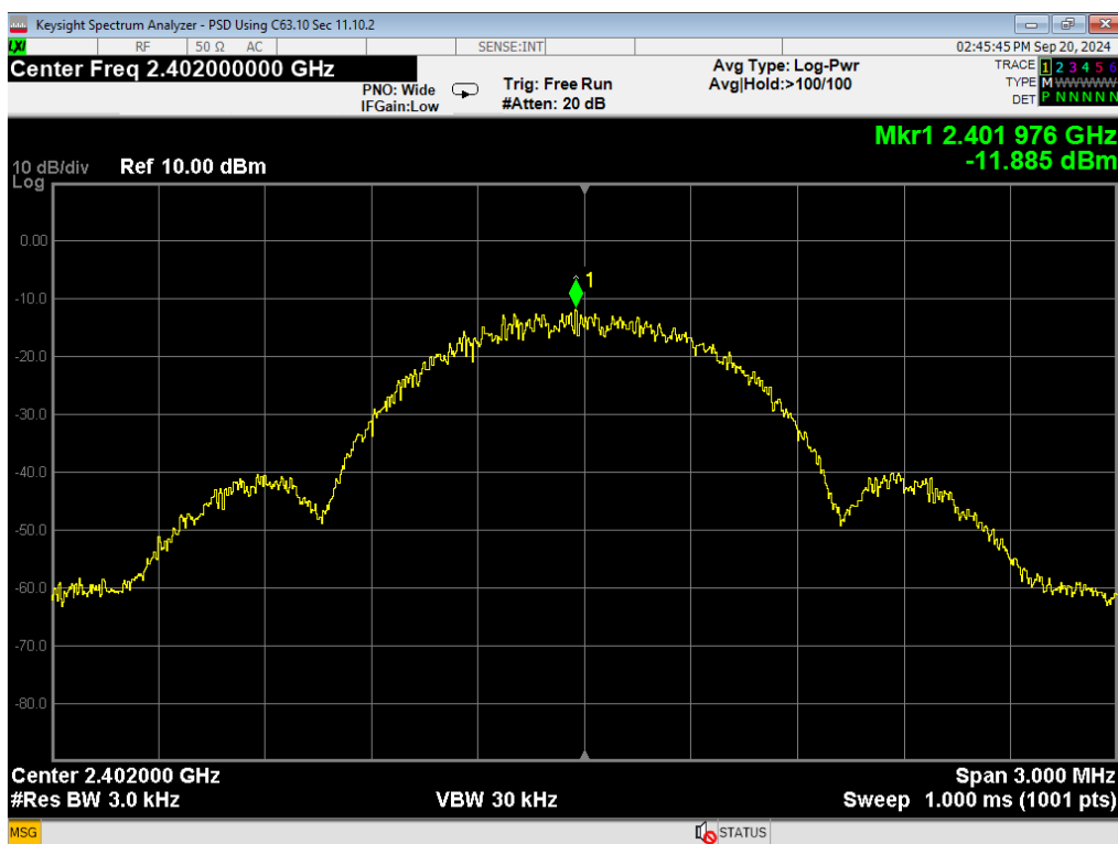
10 PSD, BLE 1MB, Low
