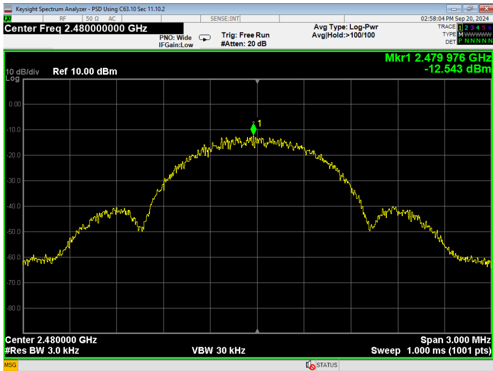
12 PSD, BLE 1MB, High
