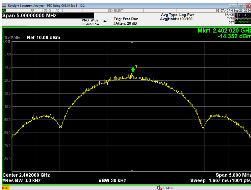
26 PSD, BLE 2MB, Low
