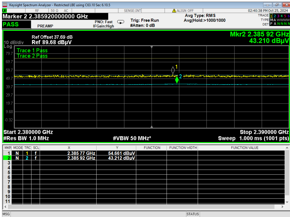
31 LBE Restricted, BLE 2MB
