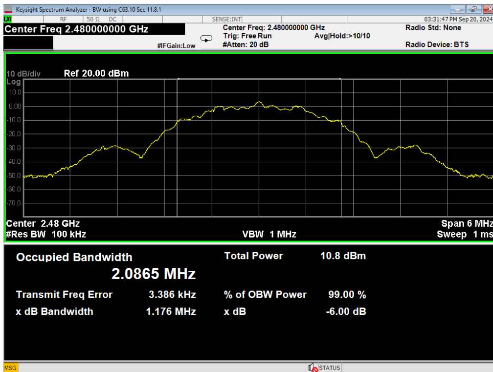
25 6dB BW, BLE 2MB, High
