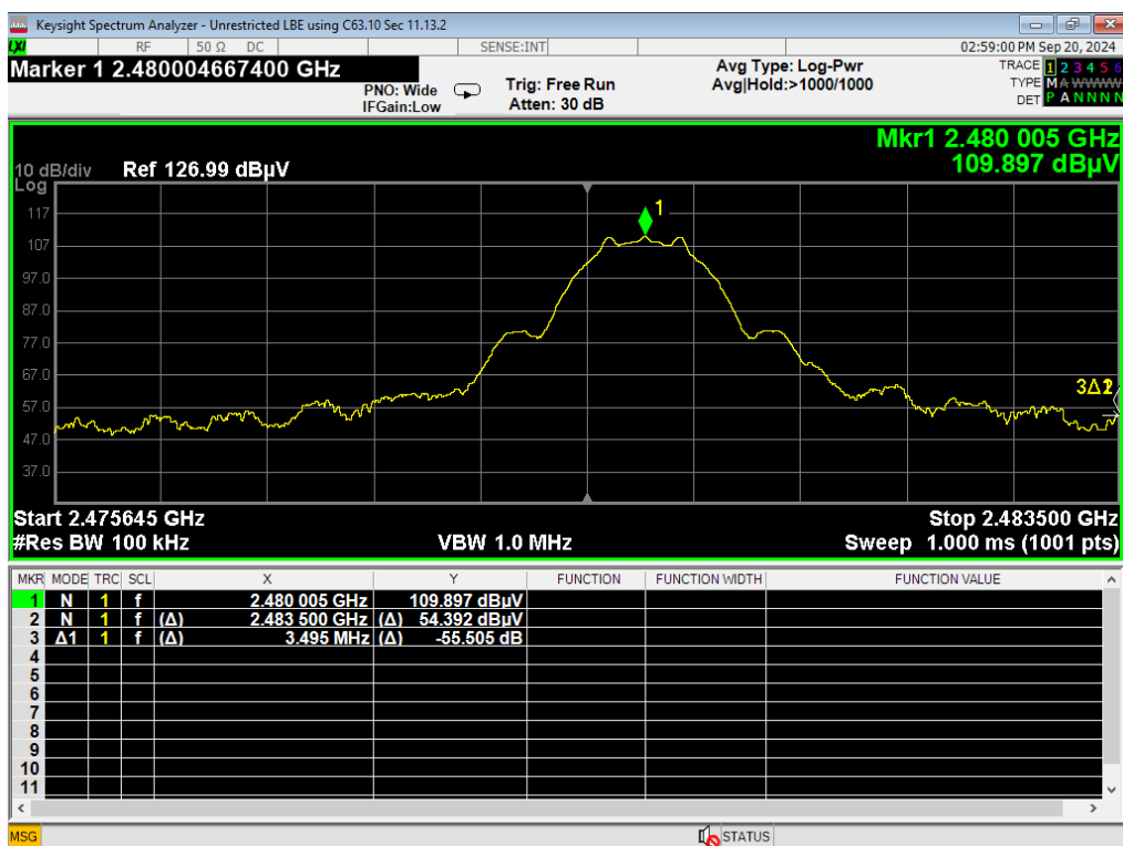
14 HBE Unrestricted, BLE 1MB
