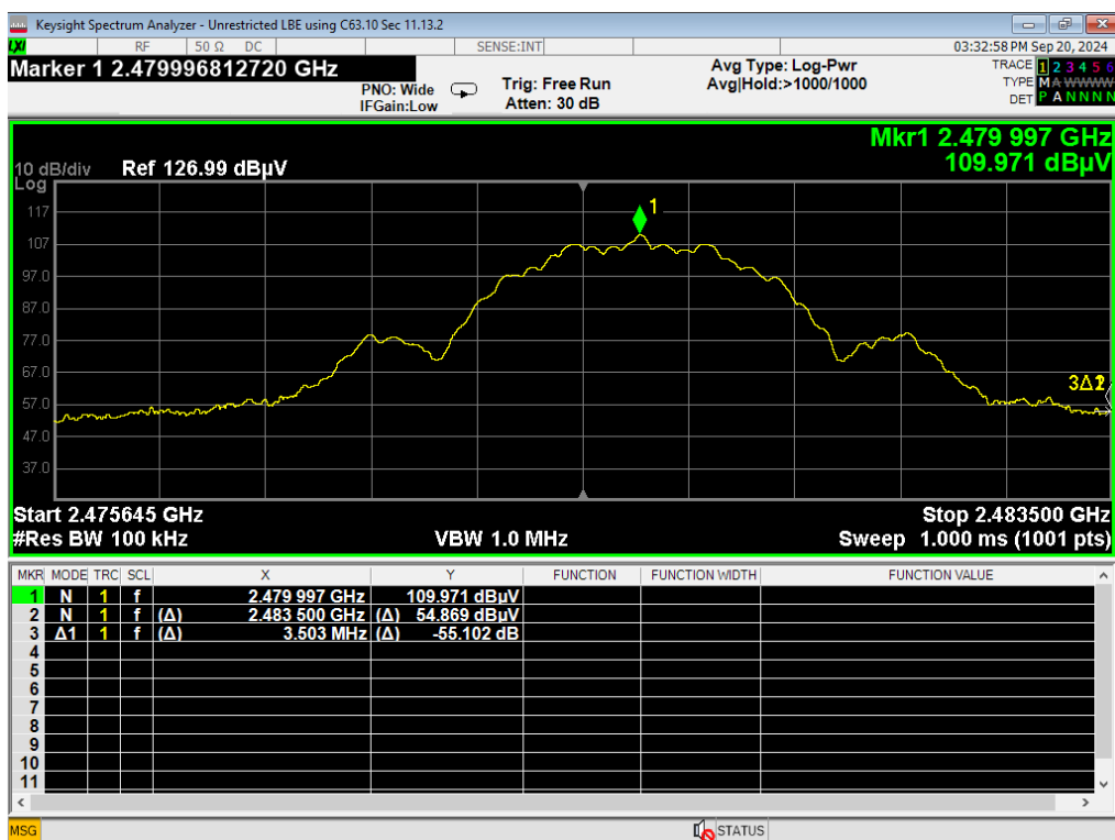
30 HBE Unrestricted, BLE 2MB
