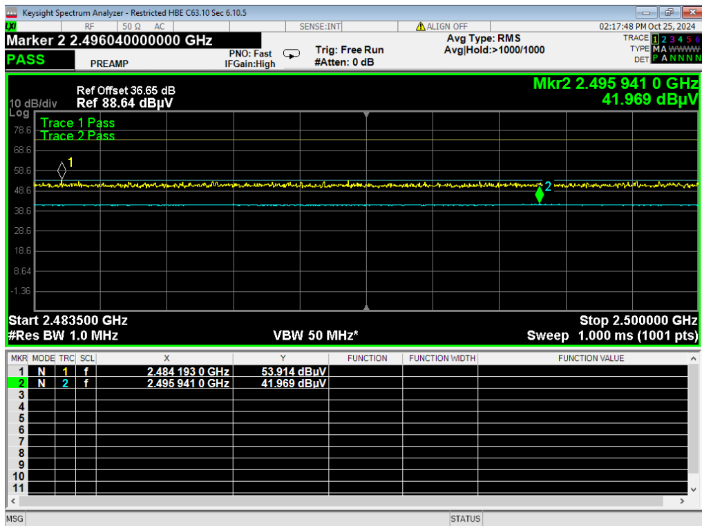
16 HBE Restricted, BLE 1MB
