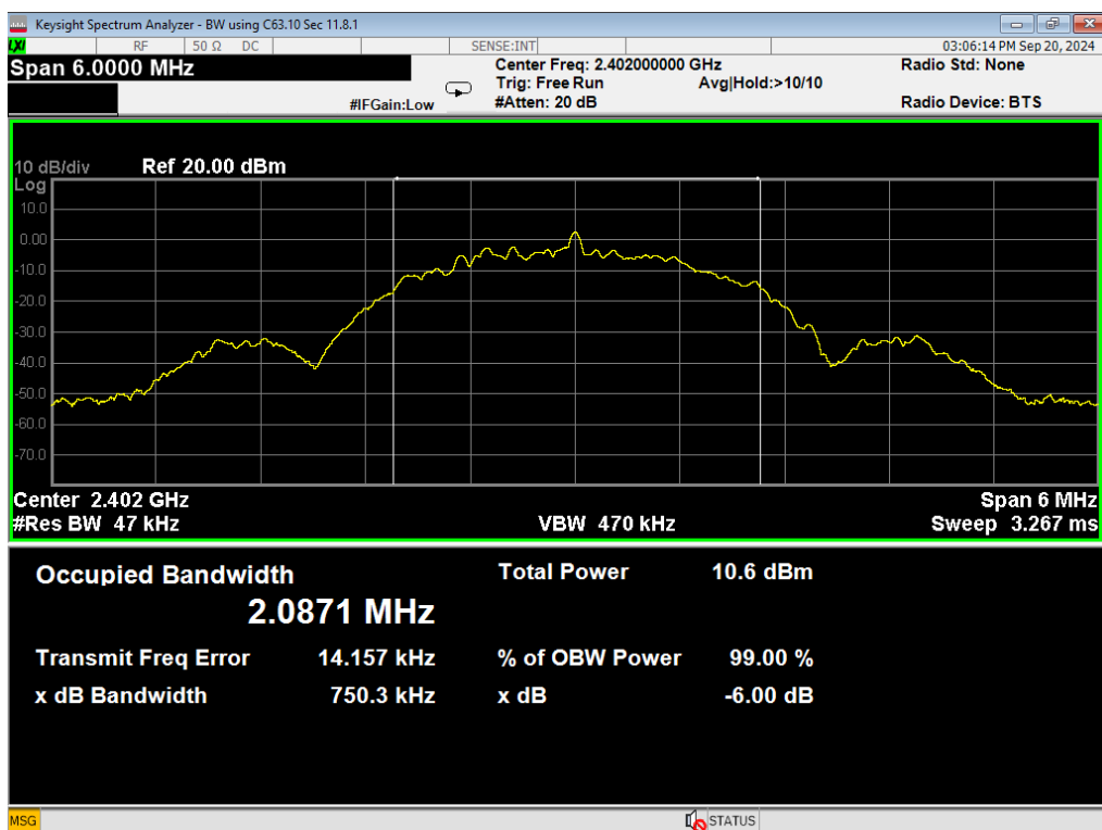
20 Occupied BW, BLE 2MB, Low
