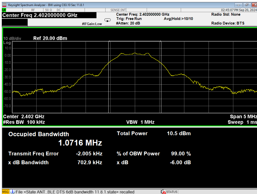
07 6dB BW, BLE 1MB, Low
