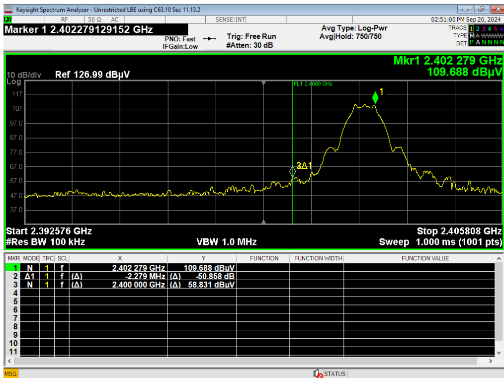
13 LBE Unrestricted, BLE 1MB
