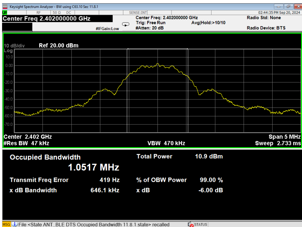
04 Occupied BW, BLE 1MB, Low
