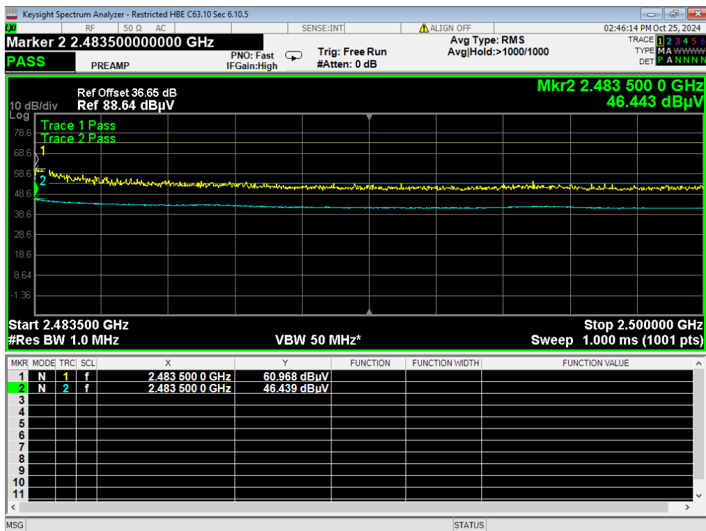
32 HBE Restricted, BLE 2MB
