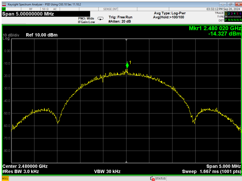
28 PSD, BLE 2MB, High
