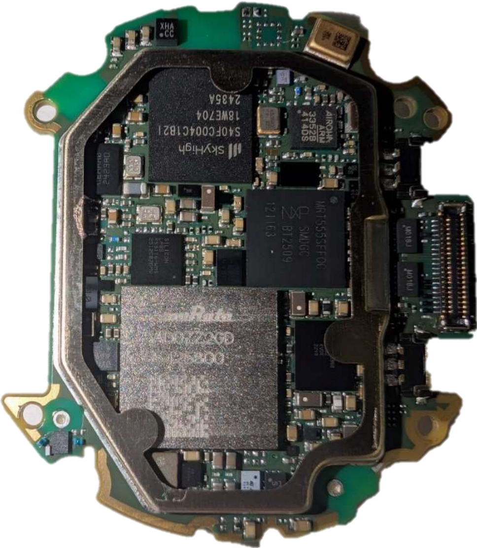
Front: PCB
