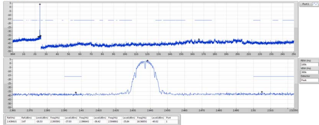
802.11b_Nss1,(1Mbps)_1TX
