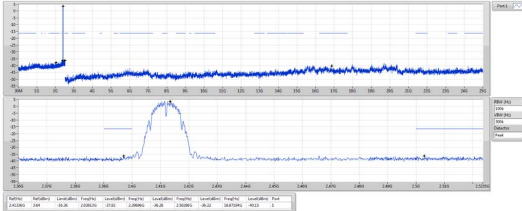
802.11b_Nss1,(1Mbps)_1TX
