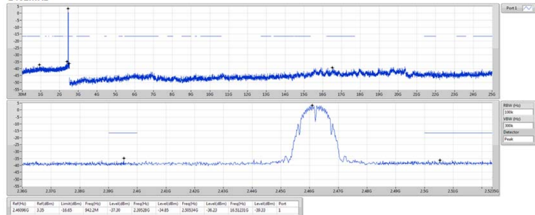
802.11b_Nss1,(1Mbps)_1TX
