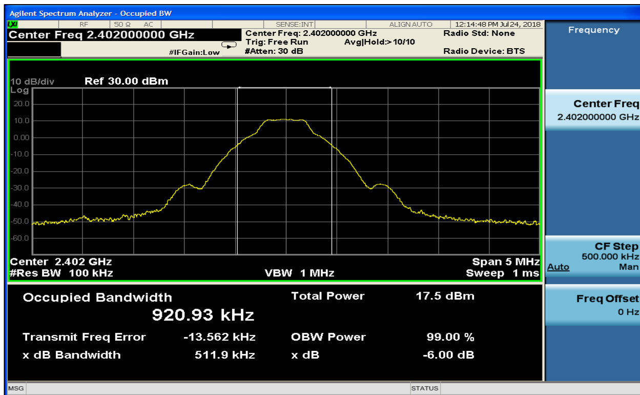
Plot 5-4: 6 dB BW – BLE – 2402 MHz
