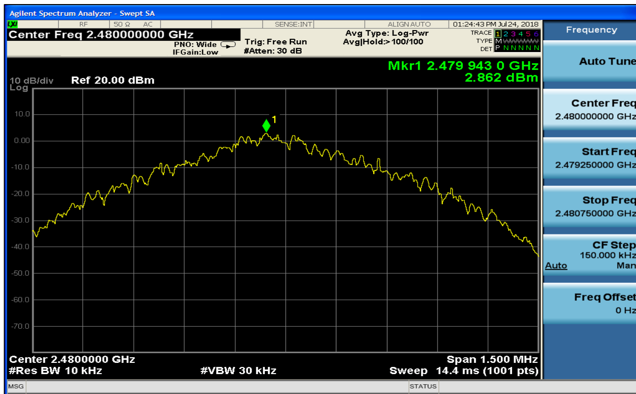
Plot 9-6: PSD – BLE – 2480 MHz
