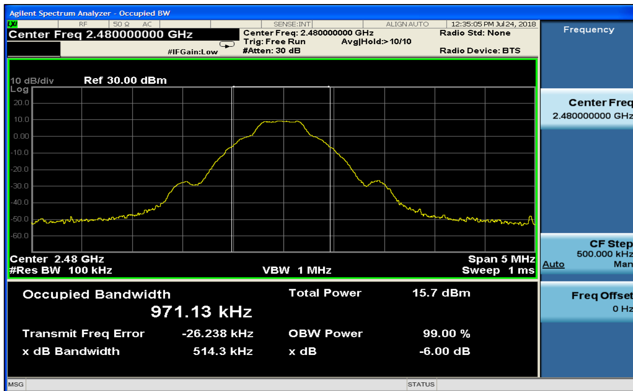
Plot 5-6: 6 dB BW – BLE – 2480 MHz
