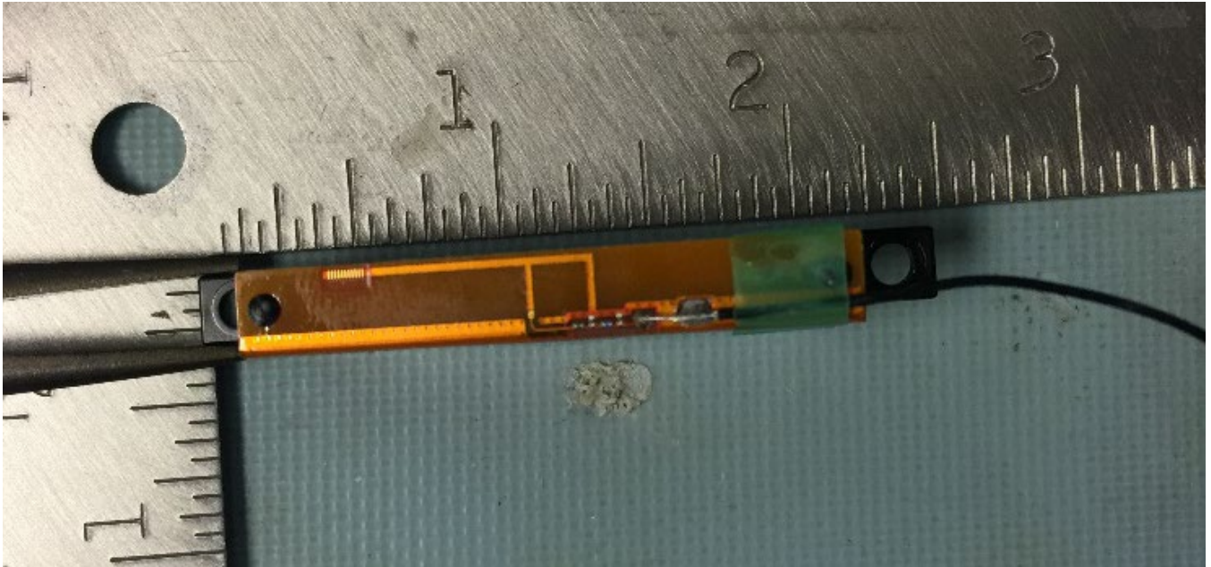
BLE / ANT antenna and WiFi antenna – Back
