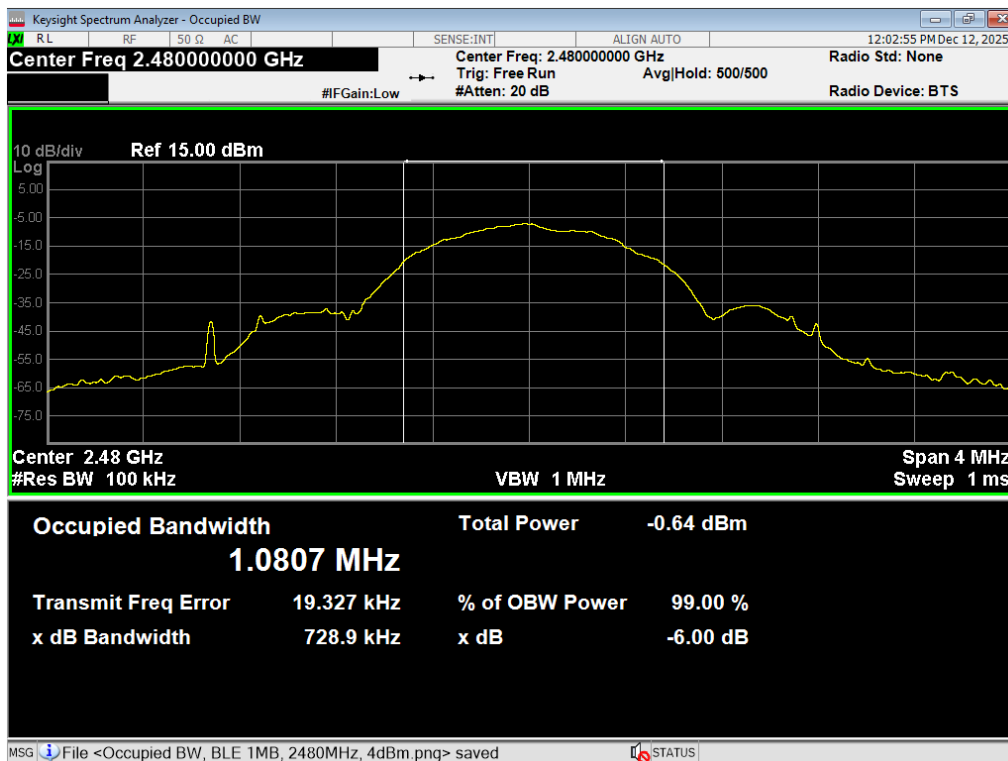
03 6dB BW, BLE 1MB, 2480MHz, 4dBm
