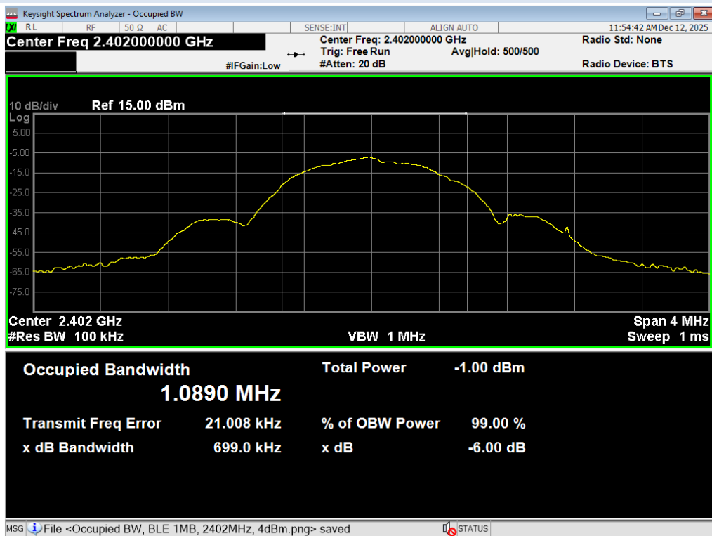
01 6dB BW, BLE 1MB, 2402MHz, 4dBm
