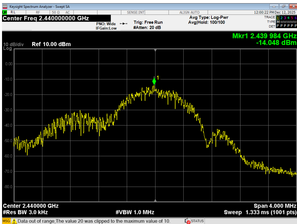
12 PSD, BLE 1MB, 2440MHz, 4dBm
