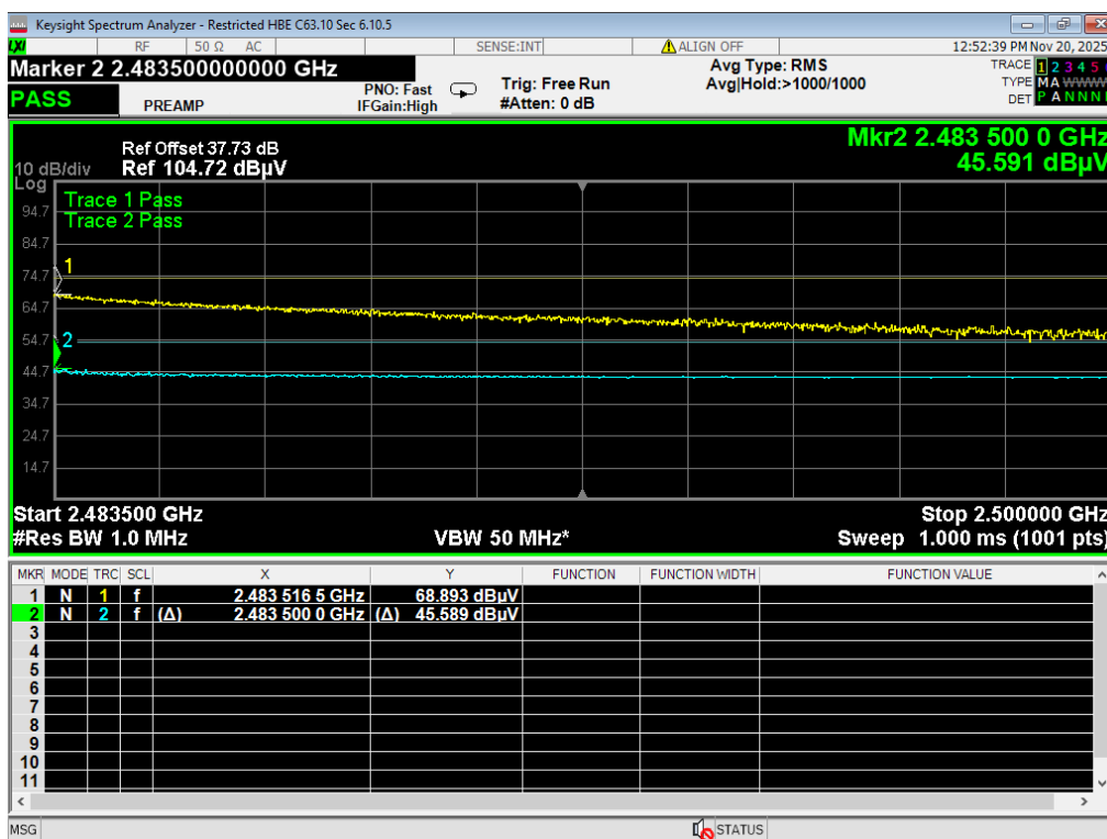
04 HBE Restricted, BLE 1MB, 2480M
