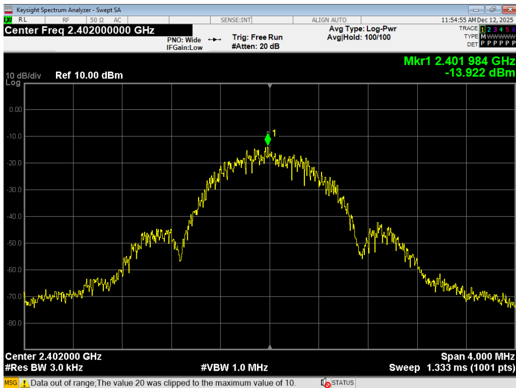
11 PSD, BLE 1MB, 2402MHz, 4dBm
