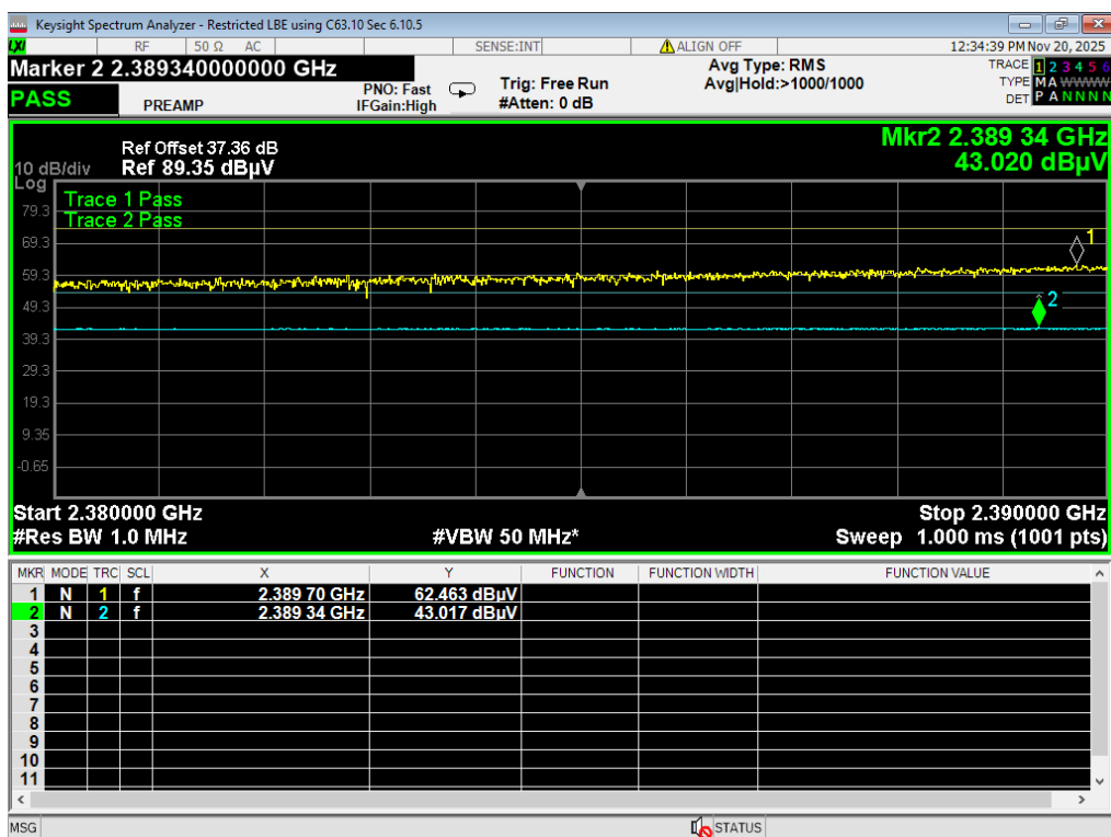
06 LBE Restricted, BLE 1MB, 2402M
