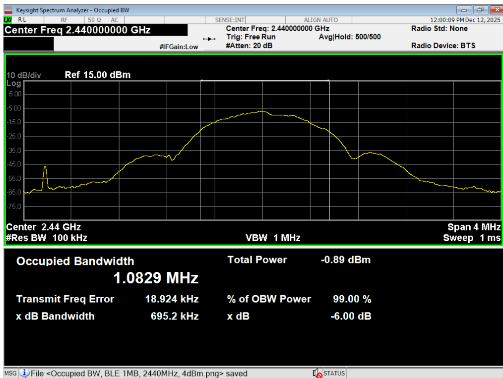
02 6dB BW, BLE 1MB, 2440MHz, 4dBm
