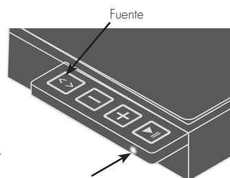
Figura 1 El indicador LED de Wi-Fi parpadea lentamente
