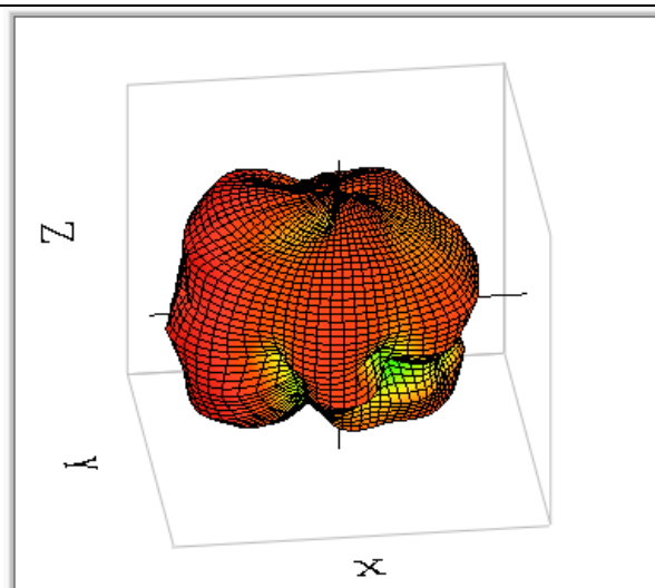
GNSS 1596MHz
