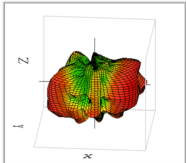
WLAN 2450MHz
