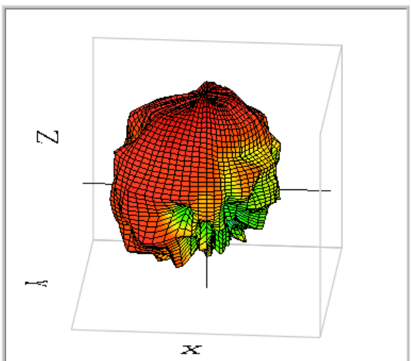
WLAN 5350MHz
