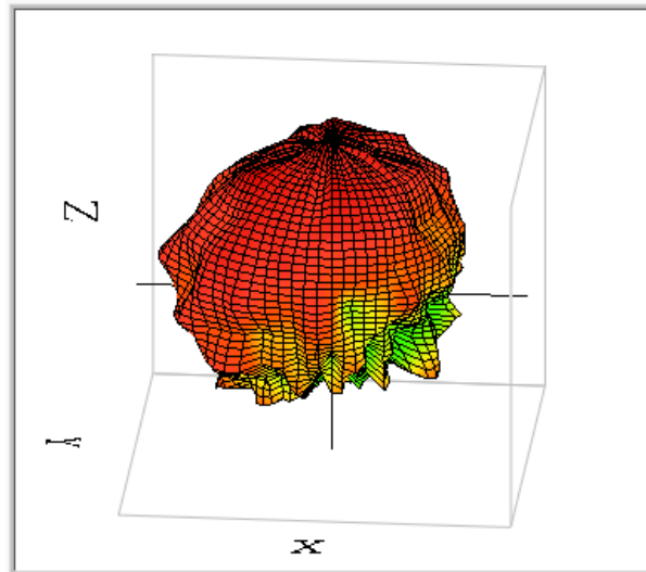
WLAN 5725MHz
