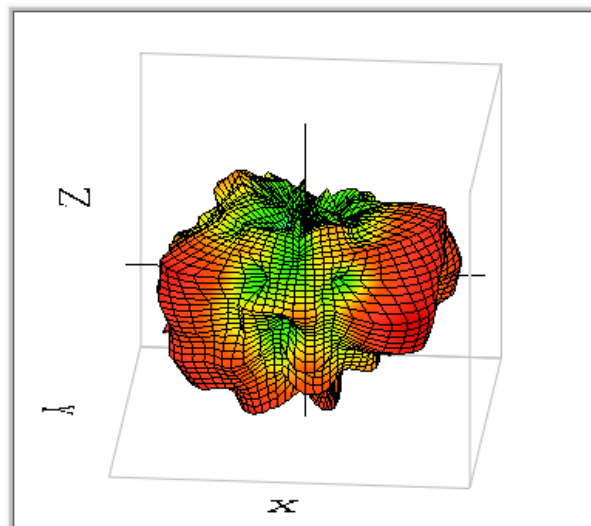
WLAN 2500MHz
