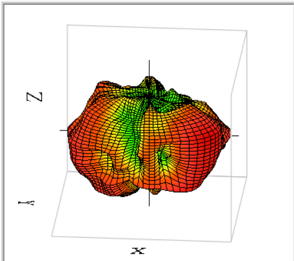
WLAN 2400MHz
