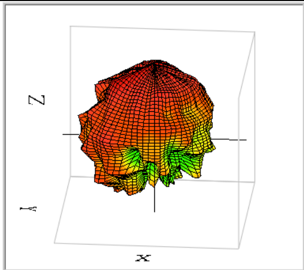
WLAN 5500MHz
