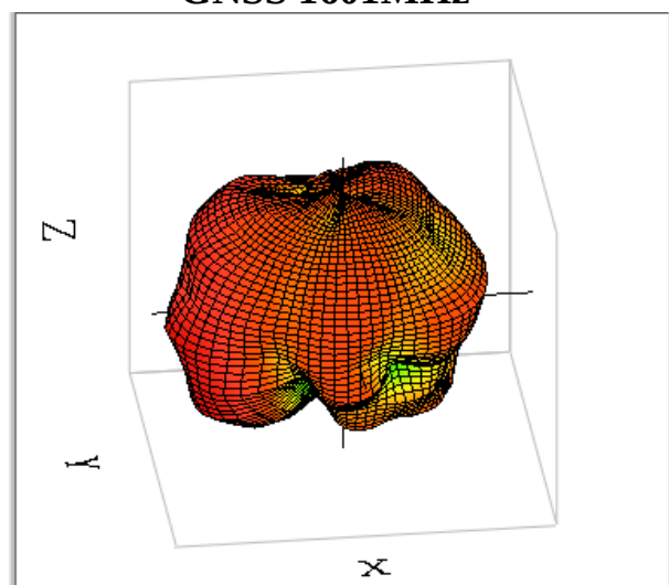
GNSS 1615MHz
