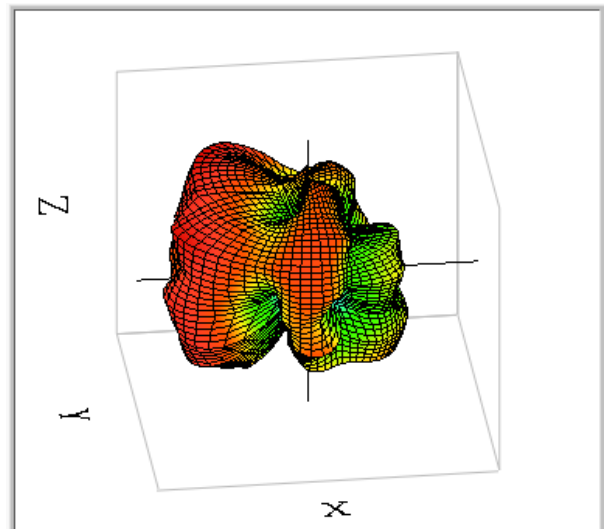
GNSS 1564MHz
