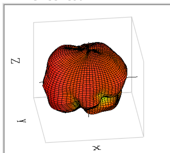
GNSS 1606MHz
