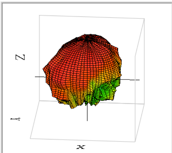
WLAN 5750MHz
