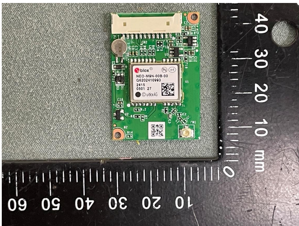
GPS Module
