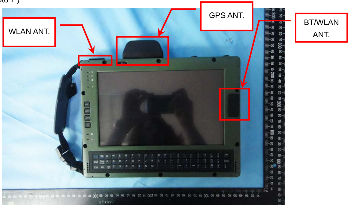
EUT Photo 1 )
