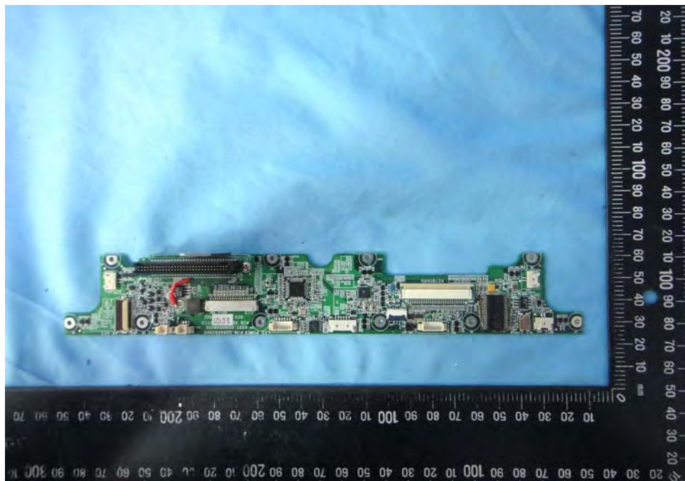
EUT Photo 46 )
