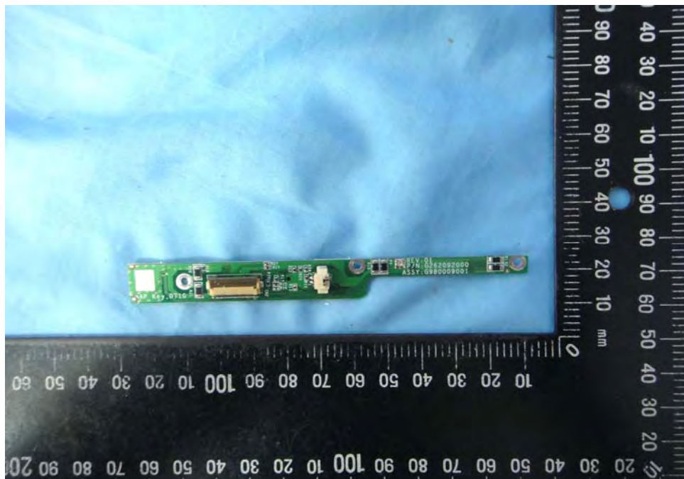
EUT Photo 50 )
