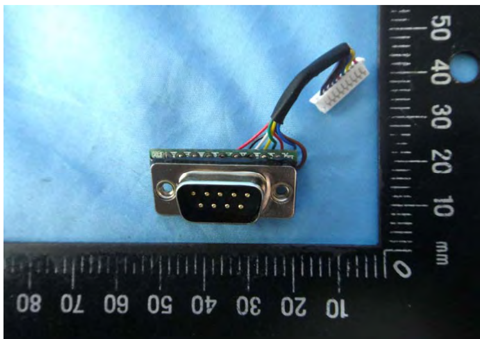
EUT Photo 40 )
