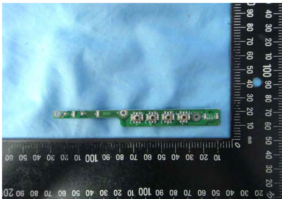
EUT Photo 52 )
