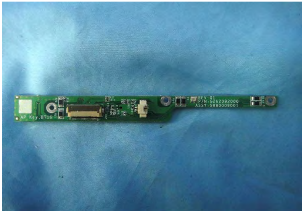
EUT Photo 52 )
