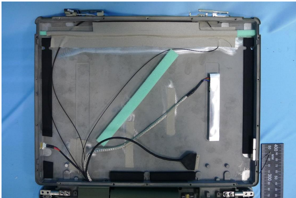
(67) EUT Photo
