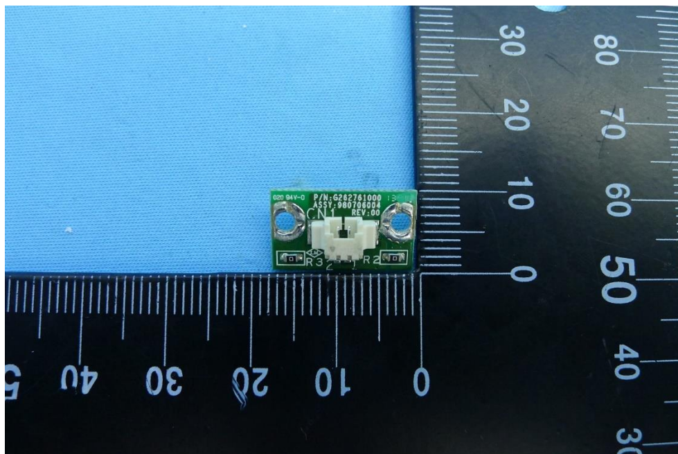
(63) EUT Photo
