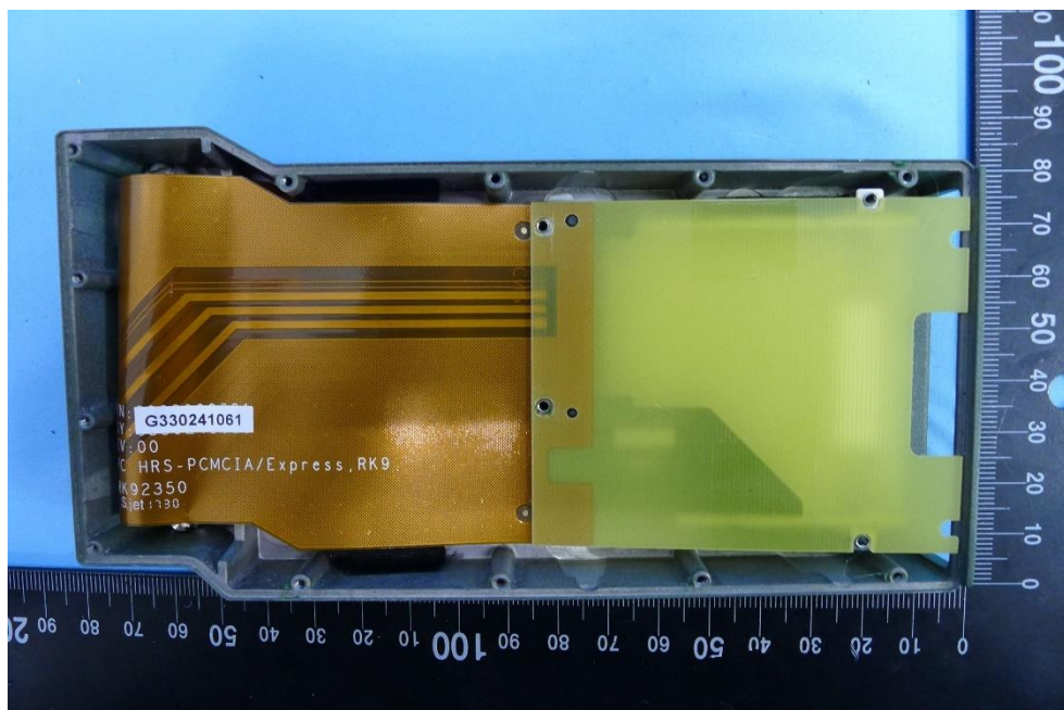
(47) EUT Photo
