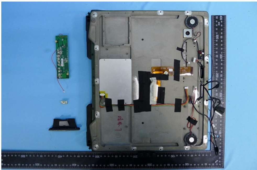
(59) EUT Photo
