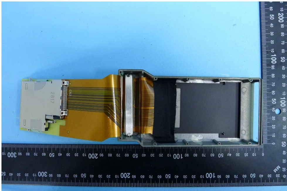
(49) EUT Photo
