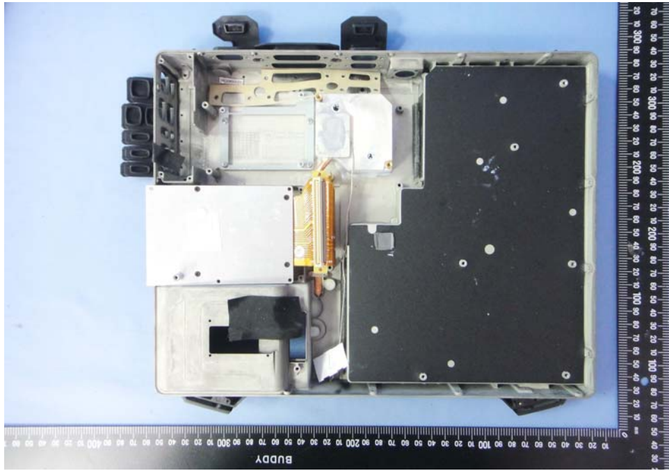
EUT Photo 93 )
