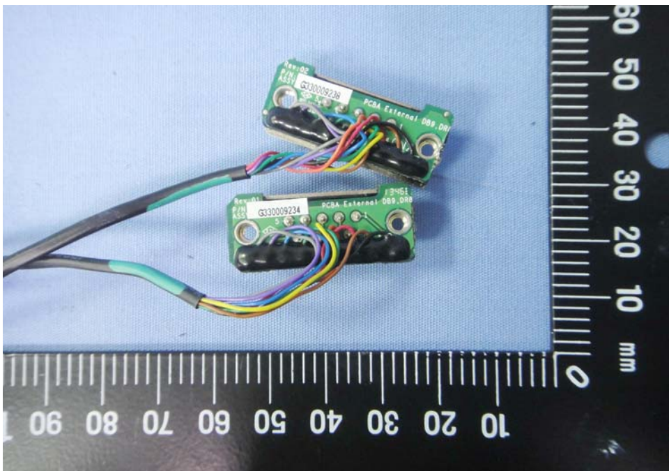
EUT Photo 90 )
