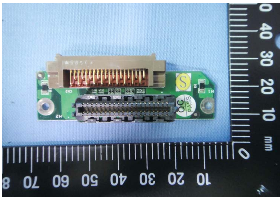
EUT Photo 72 )
