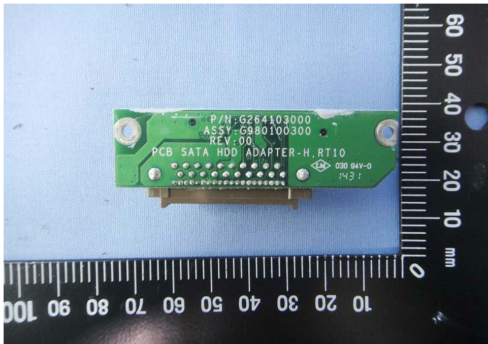
EUT Photo 74 )
