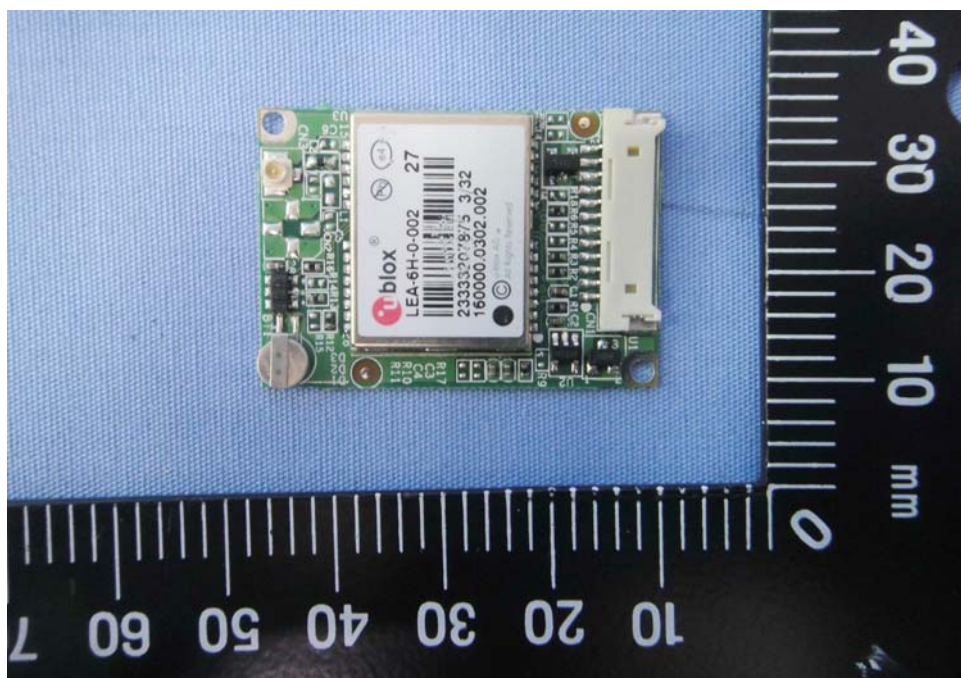
EUT Photo 74 )
