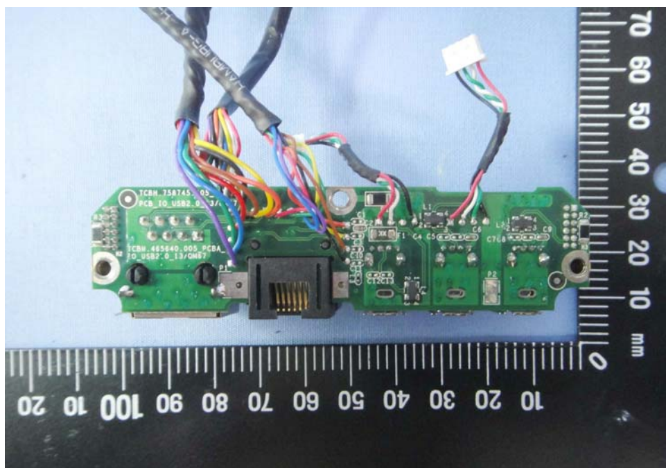
EUT Photo 88 )
