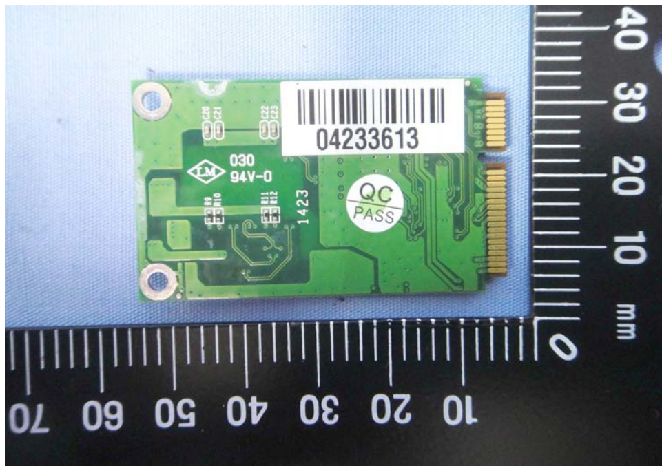
EUT Photo 56 )
