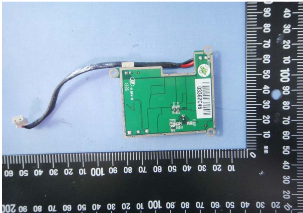
EUT Photo 78 )
