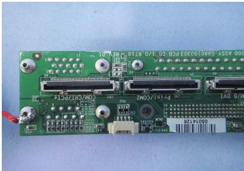
EUT Photo 82 )
