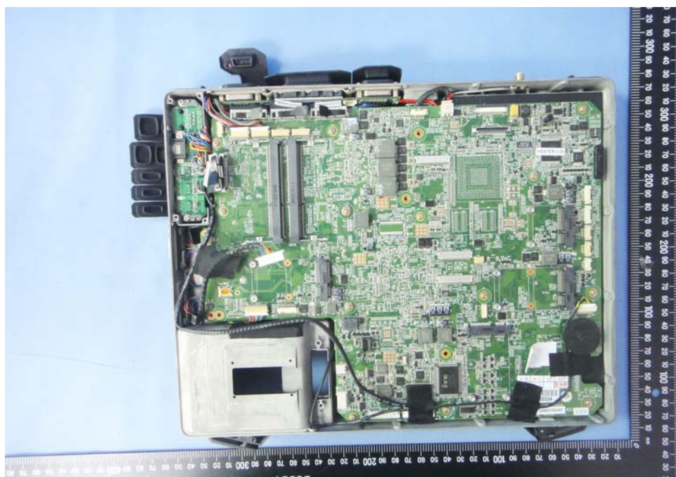
EUT Photo 58 )
