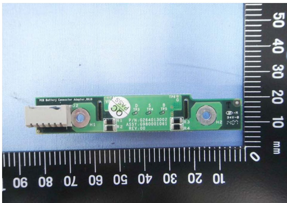
EUT Photo 56 )
