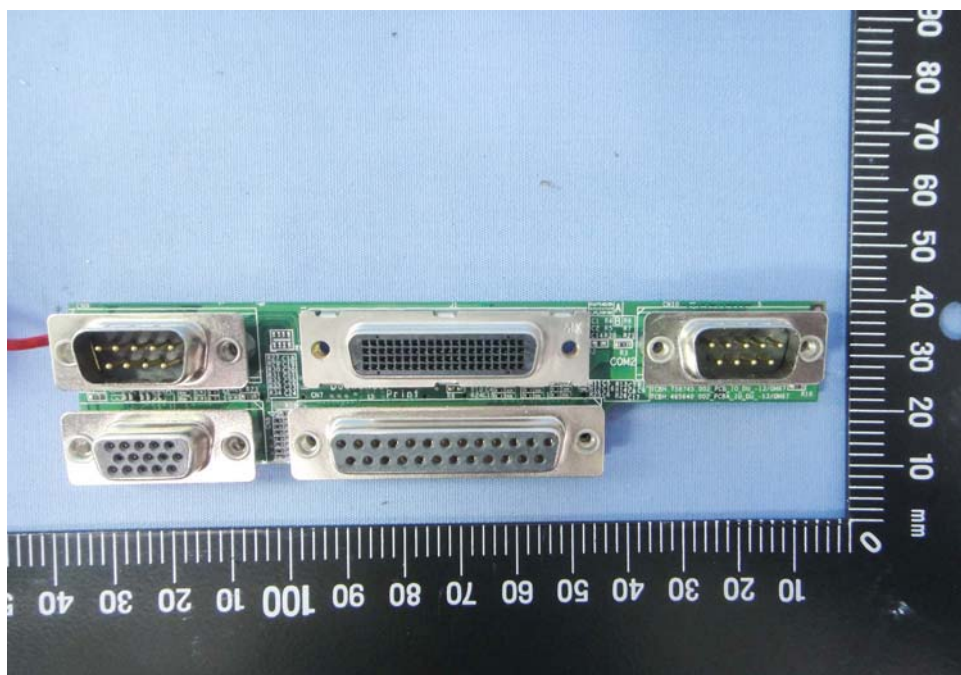
EUT Photo 84 )
