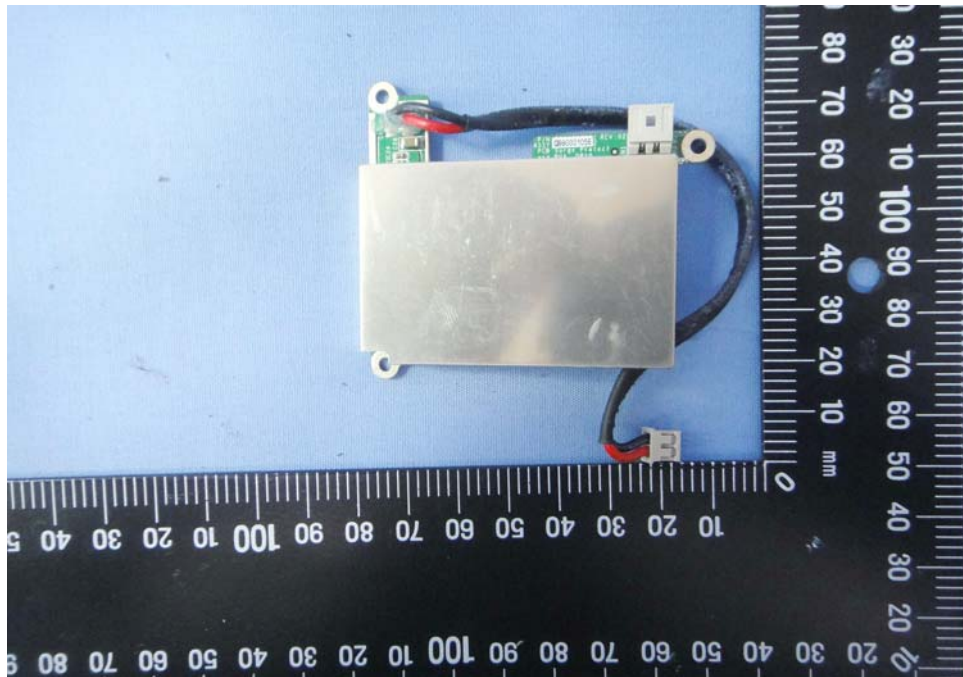
EUT Photo 80 )
