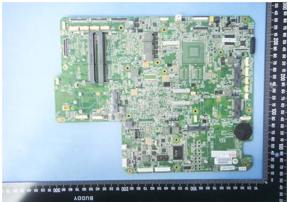
EUT Photo 60 )
