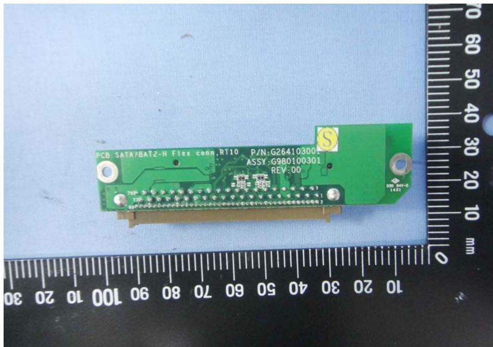
EUT Photo 72 )
