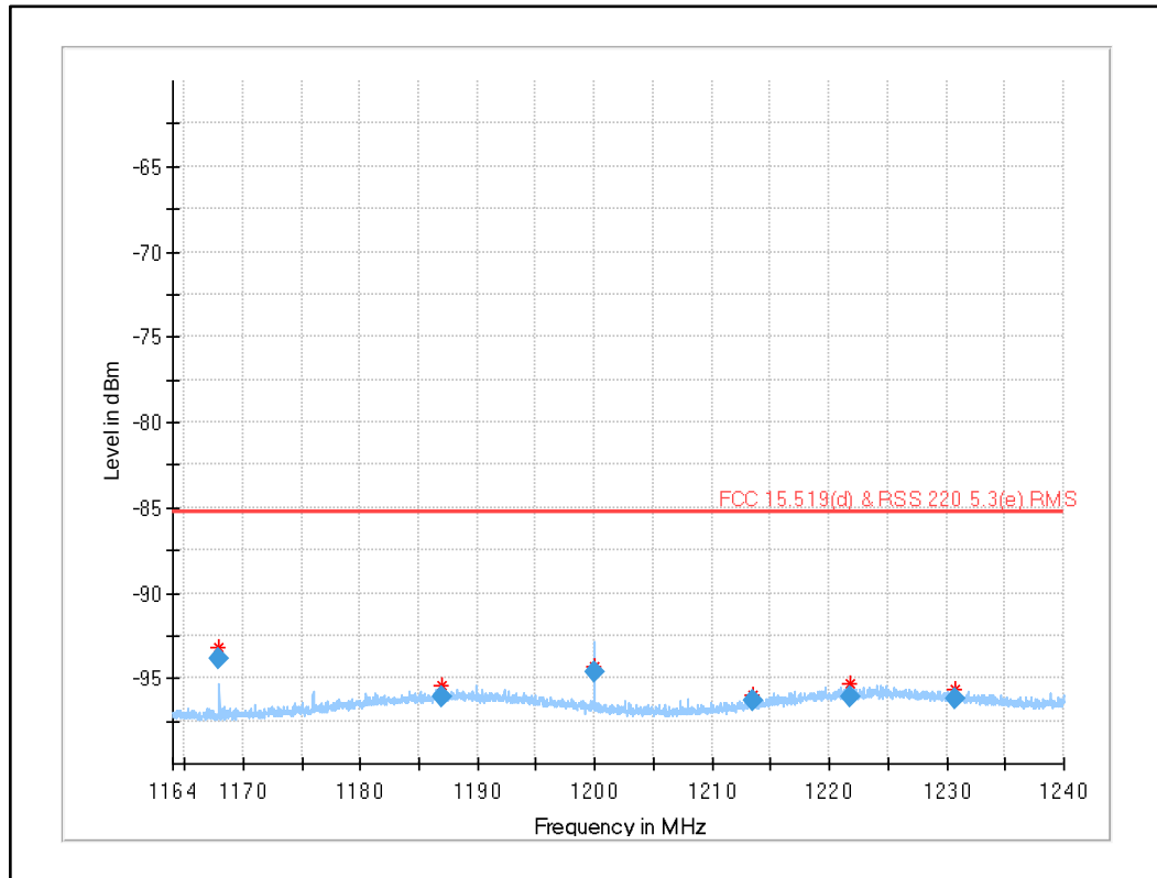
Plot 55: 1164 MHz to 1240 MHz (§15.519 (d), UWB test mode)
