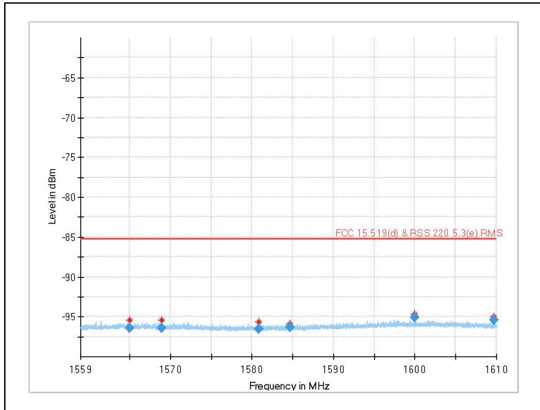
Plot 56: 1559 MHz to 1610 MHz (§15.519 (d), UWB test mode)
