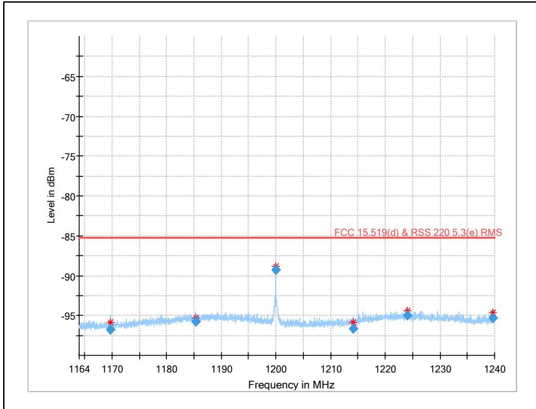
Plot 29: 1164 MHz to 1240 MHz (§15.519 (d), UWB test mode)
