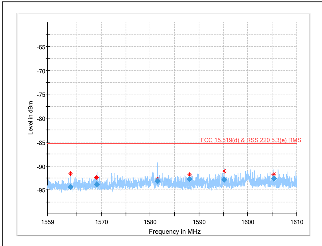
Plot 56: 1559 MHz to 1610 MHz §15.519 (d), UWB test mode
