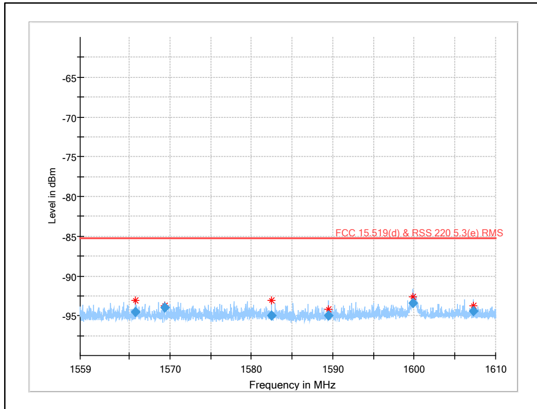
Plot 43: 1559 MHz to 1610 MHz (§15.519 (d), UWB test mode)
