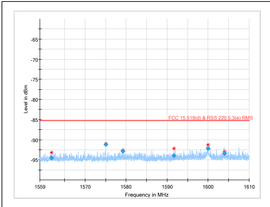
Plot 30: 1559 MHz to 1610 MHz (§15.519 (d), UWB test mode)
