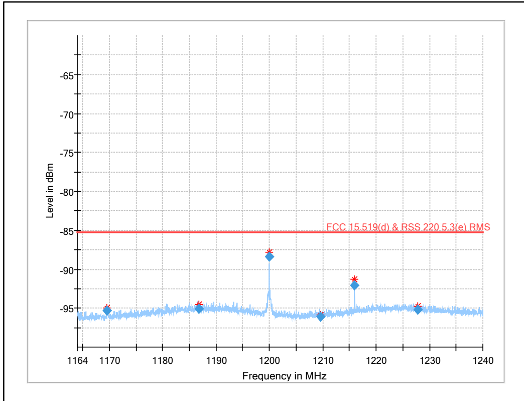
Plot 55: 1164 MHz to 1240 MHz §15.519 (d), UWB test mode
