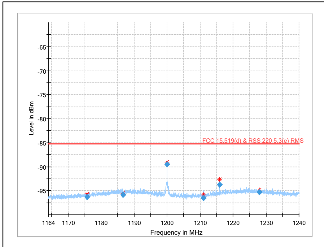
Plot 42: 1164 MHz to 1240 MHz (§15.519 (d), UWB test mode)
