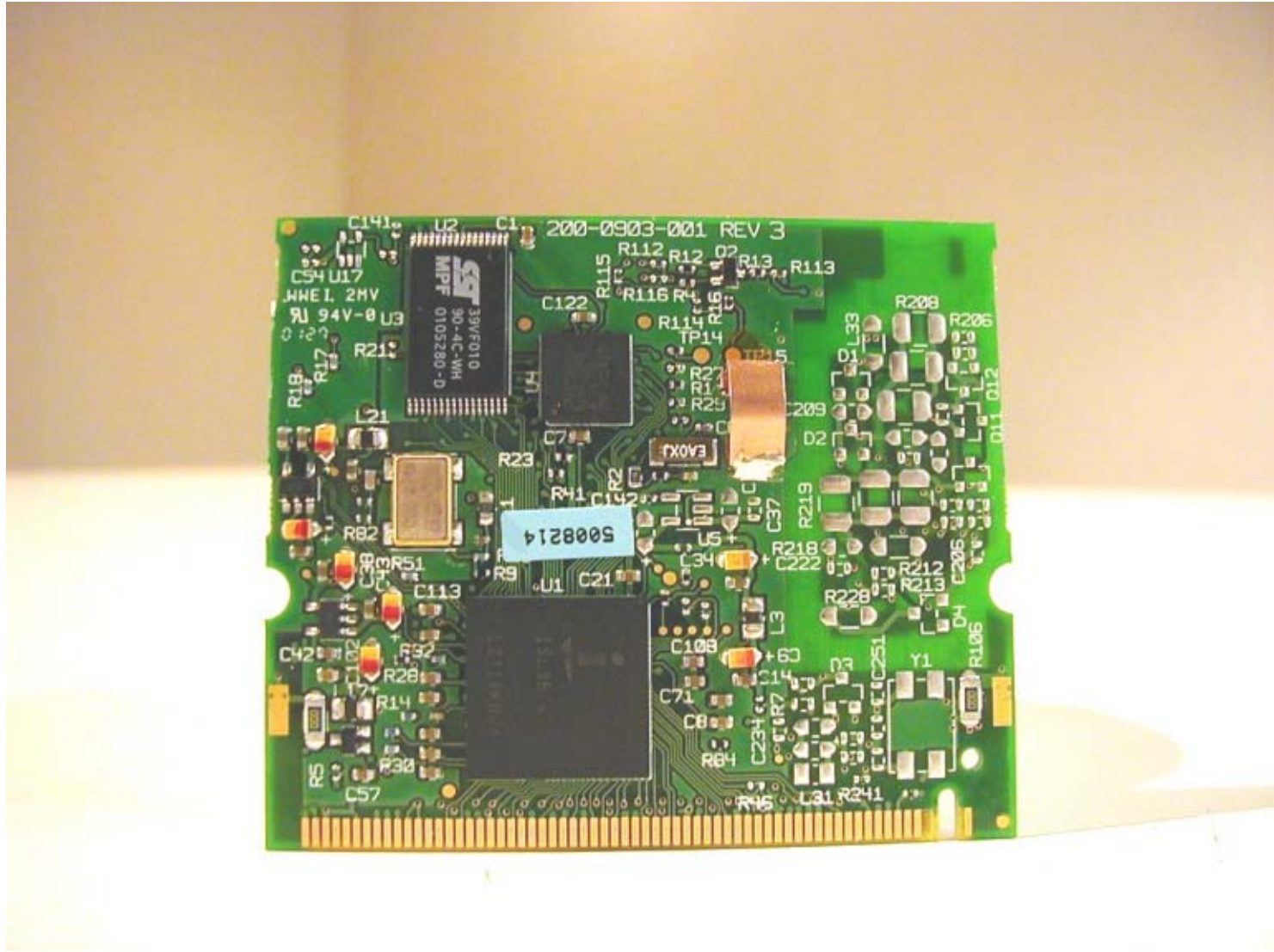
2.4 GHz Mini PCI card back side
