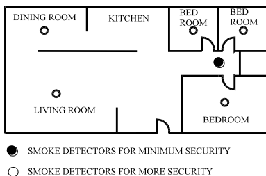
Figuur 1: Installatie van rook & hitte detectoren in een appartement of woning met 1 enkele slaapkamer
