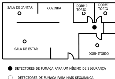
Figura 1: Locais de instalação para detectores de fumaça e calor em apartamentos ou casas para uma família com apenas uma área de dormitório
