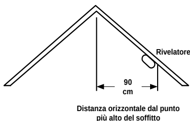
Figura 4: Posizione consigliata di installazione dei rivelatori di fumo e di calore nei locali con soffitti particolarmente inclinati ( >20^\circ ).
