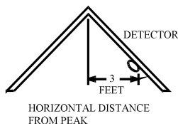
Figuur 4: Aanbevolen locatie om een rook & hitte detector te installeren in ruimtes met hellende plafonds of gevels. (helling >20 graden).
