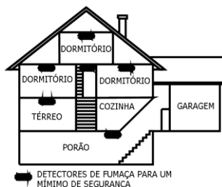
Figura 2: Locais de instalação para detectores de fumaça e calor em apartamentos ou casas com mais de um andar
