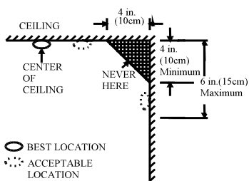
Figuur 3: Aanbevelingen om de rook & hitte detectoren op de best mogelijk locatie te installeren.
