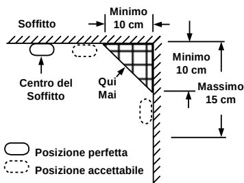
Figura 3: Posizioni perfetta e accettabile di installazione dei rivelatori di fumo e di calore.
