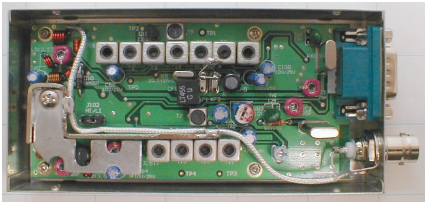
PCB Top
