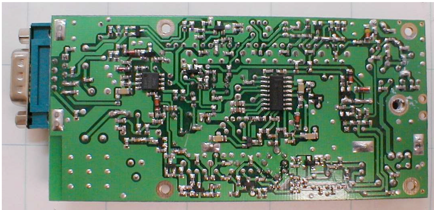
PCB Bottom
