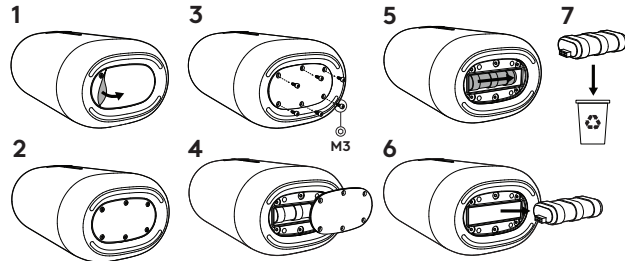
Battery removal for recycling / Retrait de la batterie pour le recyclage
