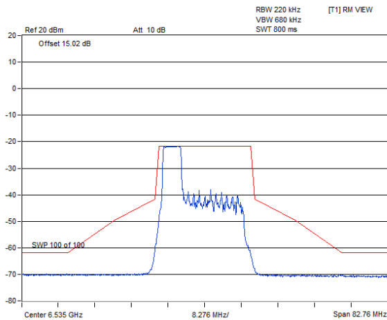
802.11ax (HE20) 52-tone RU 1Tx / Chain 0 : CH 117@37
