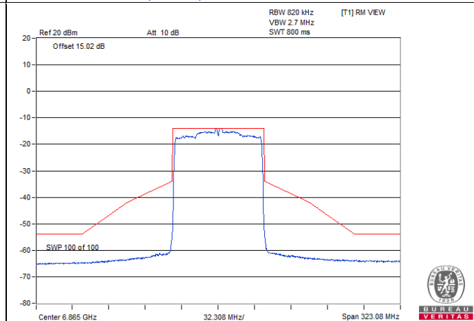
802.11ax (HE80) CDD-2Tx / Chain 1 : CH 183
