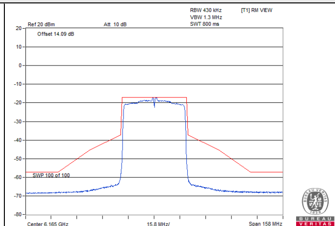
802.11ax (HE40) CDD-2Tx / Chain 1 : CH 43
