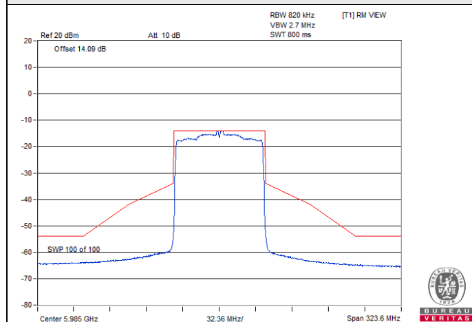
802.11ax (HE80) CDD-2Tx / Chain 0 : CH 7
