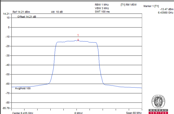
802.11ax (HE20) CDD-2Tx / Chain 1 : CH 97
