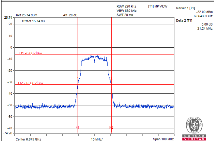
802.11a 1Tx : CH 185
