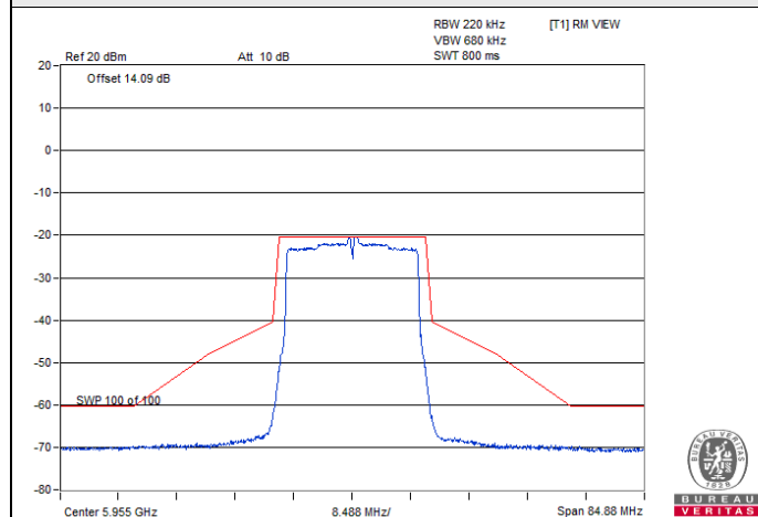
802.11ax (HE20) CDD-2Tx / Chain 0 : CH 1
