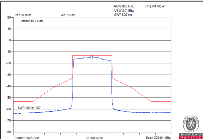
802.11ax (HE80) CDD-2Tx / Chain 0 : CH 199
