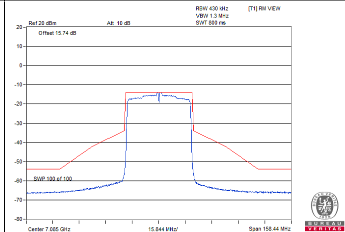
802.11ax (HE40) 1Tx / Chain 0 : CH 227
