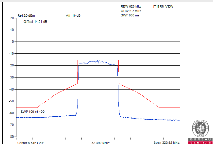
802.11ax (HE80) CDD-2Tx / Chain 1 : CH 119
