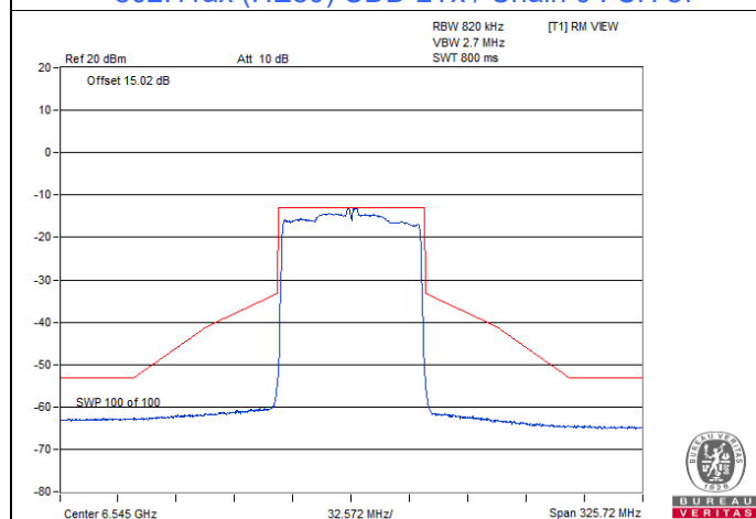
802.11ax (HE80) CDD-2Tx / Chain 0 : CH 119
