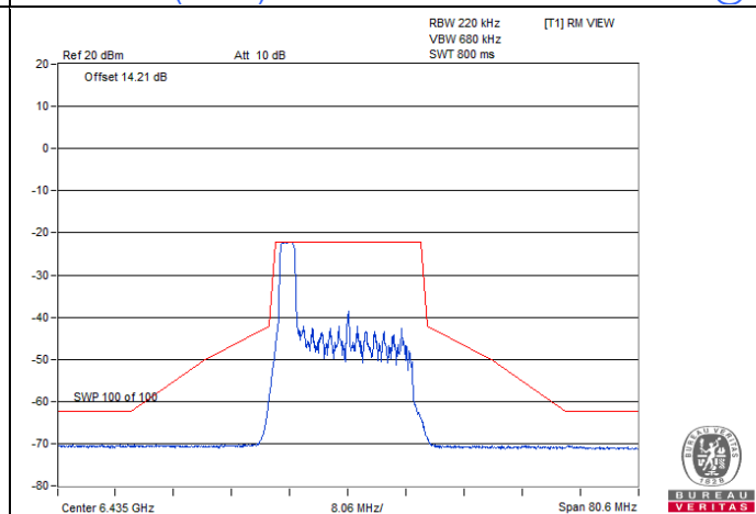
802.11ax (HE20) 26-tone RU 1Tx / Chain 0 : CH 97@0
