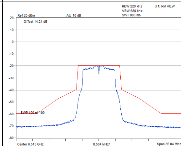
802.11a CDD-2Tx / Chain 0 : CH 113
