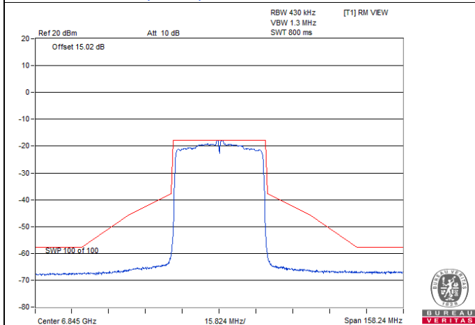
802.11ax (HE40) CDD-2Tx / Chain 0 : CH 179
