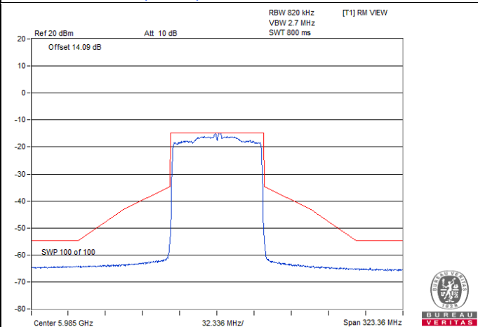
802.11ax (HE80) CDD-2Tx / Chain 1 : CH 7
