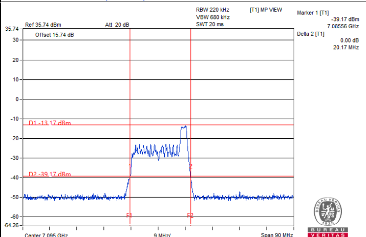
802.11ax (HE20) 26-tone RU CDD-2Tx / Chain 0 : CH 229@8
