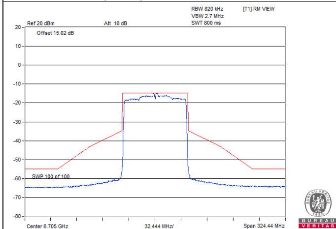
802.11ax (HE80) CDD-2Tx / Chain 1 : CH 151
