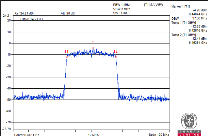
802.11ax (HE40) CDD-2Tx / Chain 0 : CH 99
