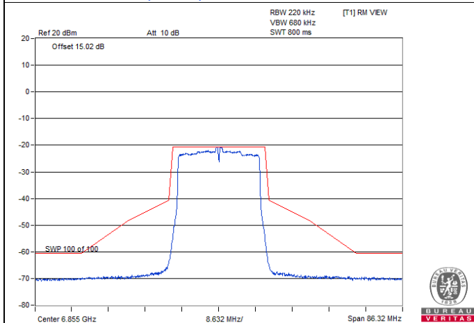
802.11ax (HE20) CDD-2Tx / Chain 0 : CH 181
