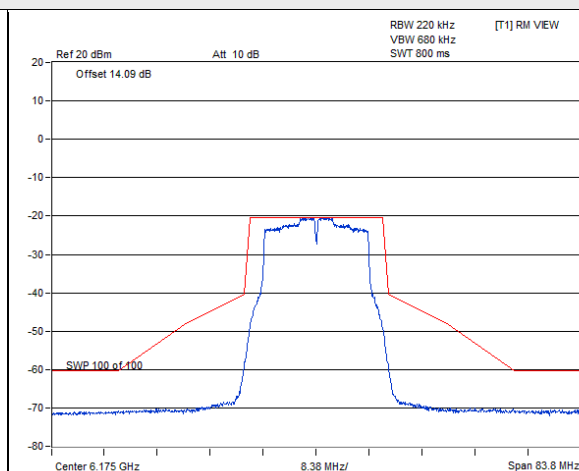
802.11a CDD-2Tx / Chain 0 : CH 45
