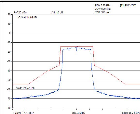
802.11ax (HE20) 1Tx / Chain 0 : CH 45
