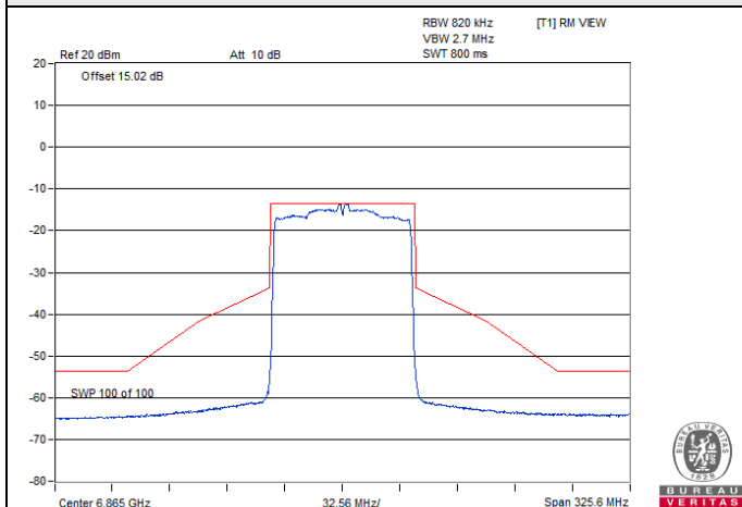
802.11ax (HE80) CDD-2Tx / Chain 0 : CH 183
