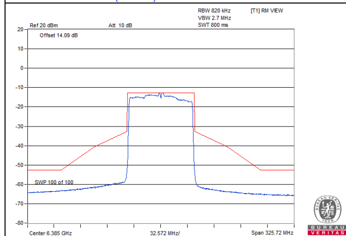
802.11ax (HE80) CDD-2Tx / Chain 0 : CH 87
