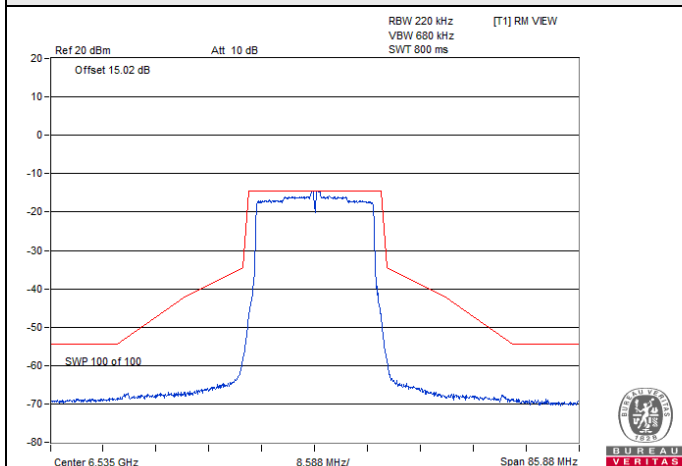
802.11ax (HE20) 1Tx / Chain 0 : CH 117
