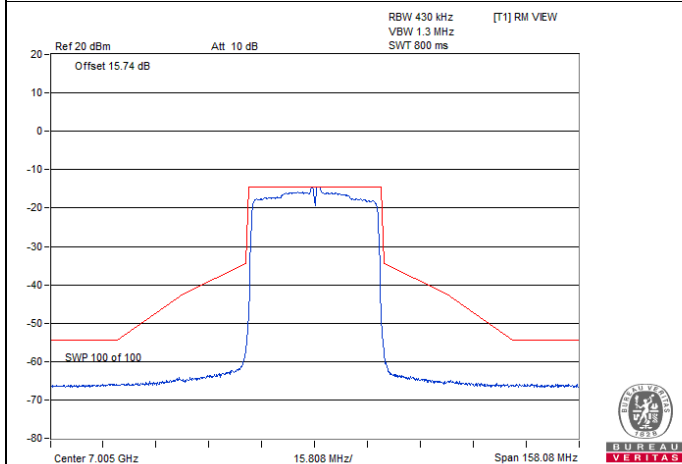
802.11ax (HE40) 1Tx / Chain 0 : CH 211
