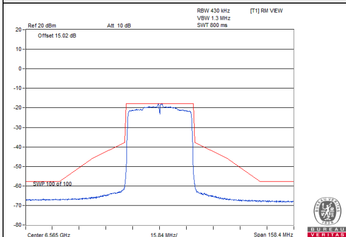
802.11ax (HE40) CDD-2Tx / Chain 1 : CH 123
