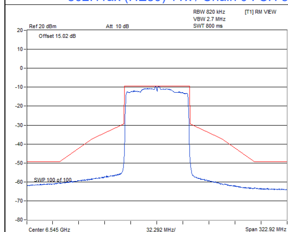
802.11ax (HE80) 1Tx / Chain 0 : CH 119
