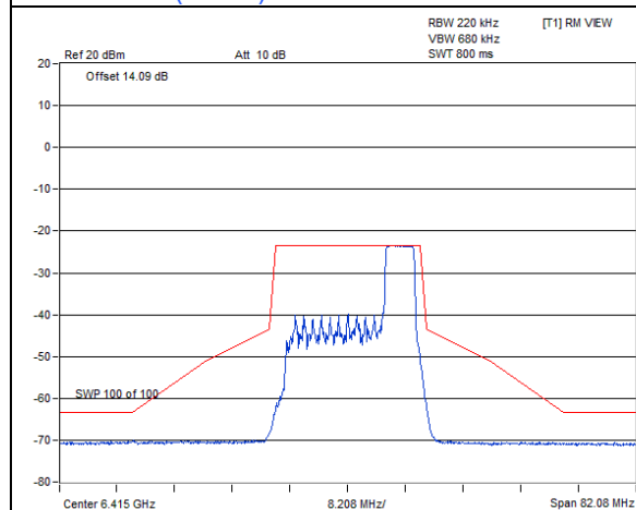
802.11ax (HE20) 52-tone RU 1Tx / Chain 0 : CH 93@40
