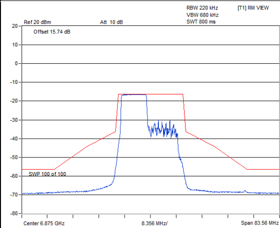
802.11ax (HE20) 106-tone RU 1Tx / Chain 0 : CH 185@53
