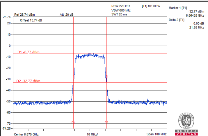
802.11ax (HE20) 1Tx : CH 185
