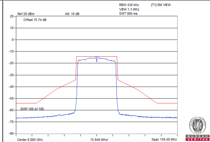
802.11ax (HE40) 1Tx / Chain 0 : CH 187
