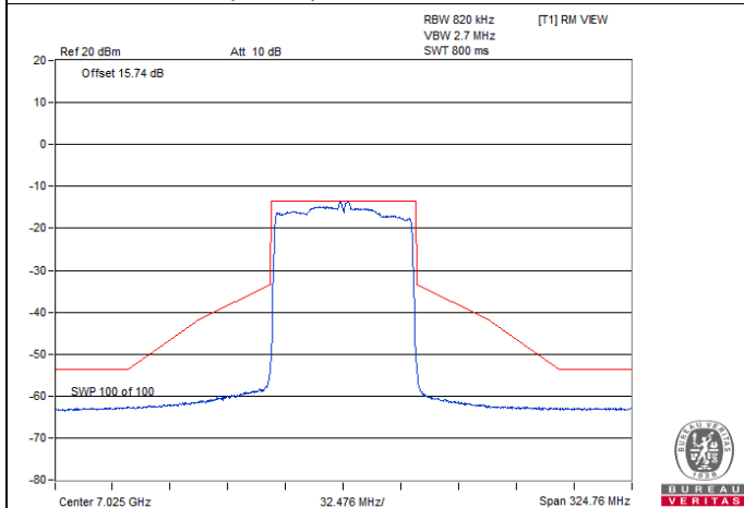
802.11ax (HE80) CDD-2Tx / Chain 0 : CH 215
