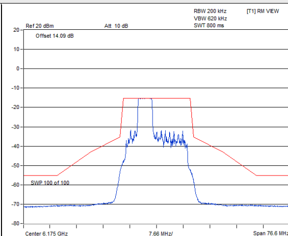
802.11ax (HE20) 52-tone RU 1Tx / Chain 0 : CH 45@38
