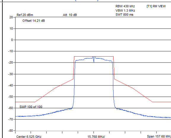
802.11ax (HE40) 1Tx / Chain 0 : CH 115
