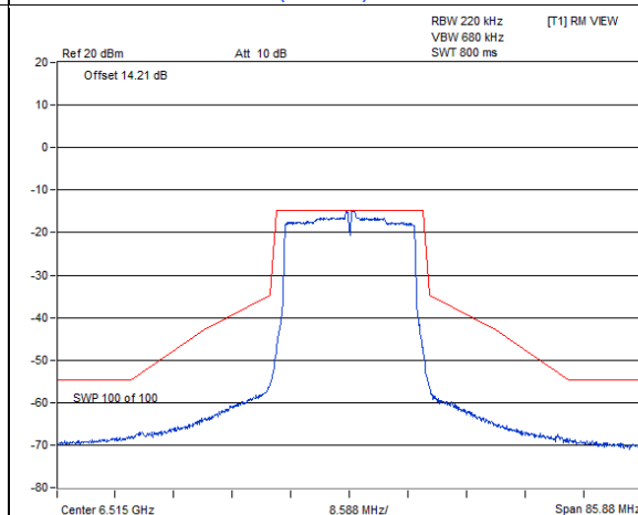
802.11ax (HE20) 1Tx / Chain 0 : CH 113
