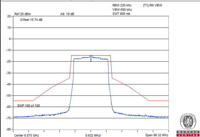
802.11ax (HE20) 1Tx / Chain 0 : CH 185
