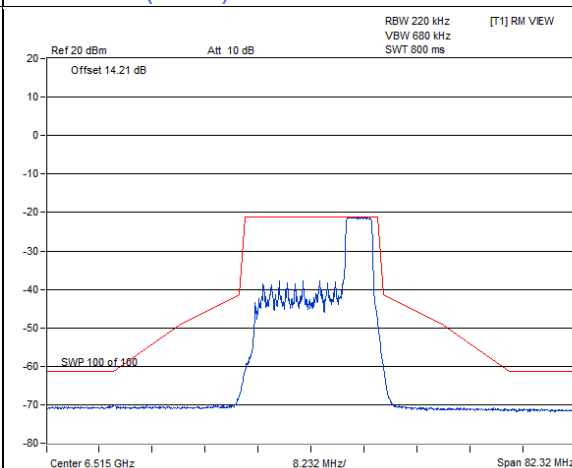
802.11ax (HE20) 52-tone RU 1Tx / Chain 0 : CH 113@40
