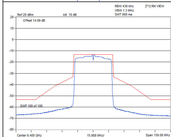
802.11ax (HE40) 1Tx / Chain 0 : CH 91
