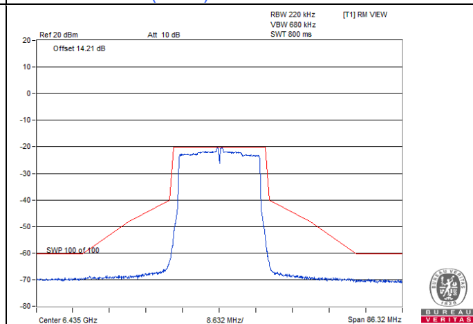
802.11ax (HE20) CDD-2Tx / Chain 0 : CH 97
