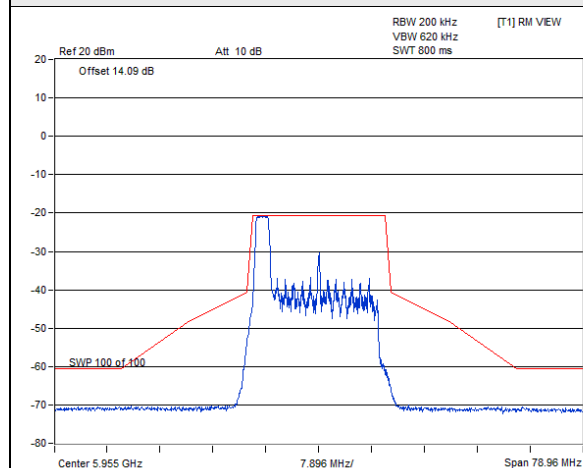
802.11ax (HE20) 26-tone RU CDD-2Tx / Chain 0 : CH 1@0
