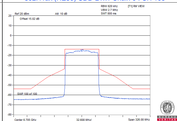
802.11ax (HE80) CDD-2Tx / Chain 0 : CH 151
