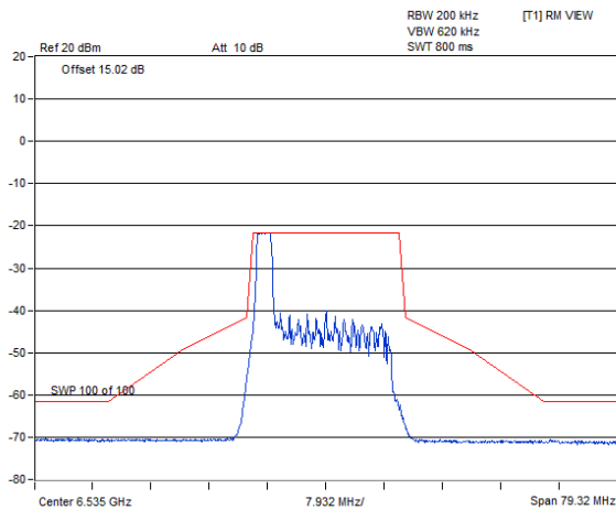
802.11ax (HE20) 26-tone RU 1Tx / Chain 0 : CH 117@0
