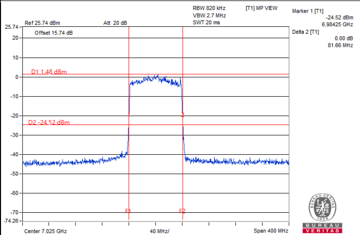
802.11ax (HE80) 1Tx : CH 215
