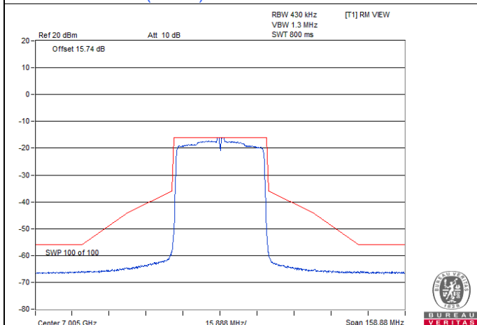
802.11ax (HE40) CDD-2Tx / Chain 1 : CH 211
