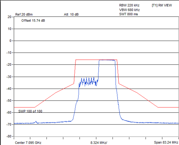
802.11ax (HE20) 106-tone RU 1Tx / Chain 0 : CH 229@54
