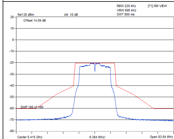
802.11a CDD-2Tx / Chain 0 : CH 93
