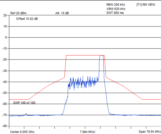
802.11ax (HE20) 26-tone RU 1Tx / Chain 0 : CH 181@8
