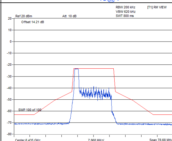
802.11ax (HE20) 26-tone RU CDD-2Tx / Chain 0 : CH 97@0
