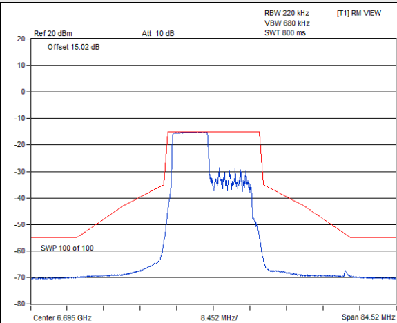
802.11ax (HE20) 106-tone RU 1Tx / Chain 0 : CH 149@53
