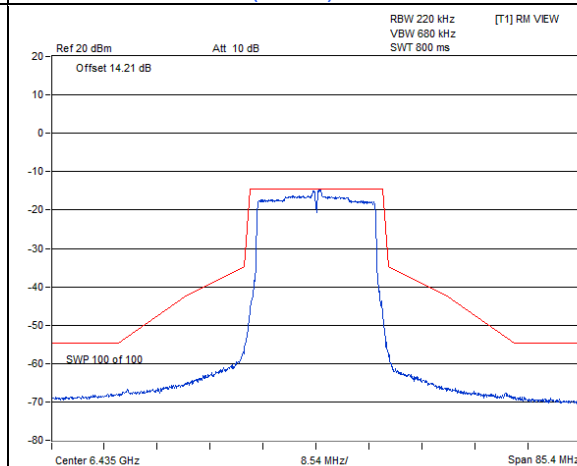
802.11ax (HE20) 1Tx / Chain 0 : CH 97
