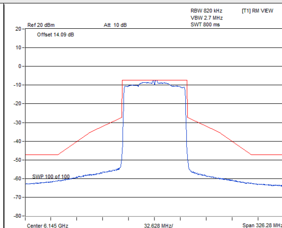
802.11ax (HE80) 1Tx / Chain 0 : CH 39
