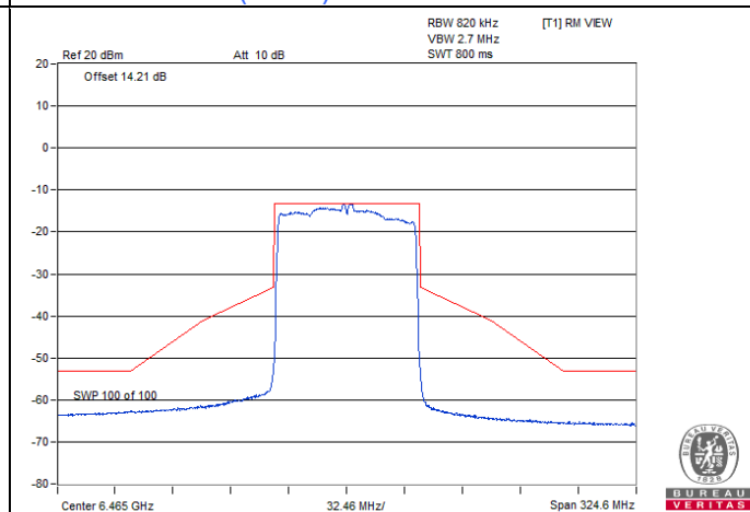
802.11ax (HE80) CDD-2Tx / Chain 0 : CH 103
