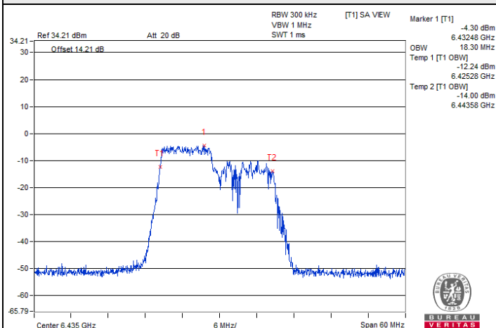
802.11ax (HE20) 106-tone RU 1Tx / Chain 0 : CH 97@53
