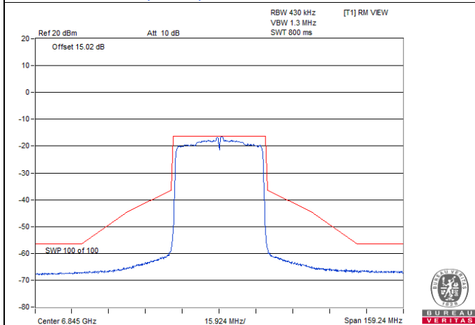
802.11ax (HE40) CDD-2Tx / Chain 1 : CH 179
