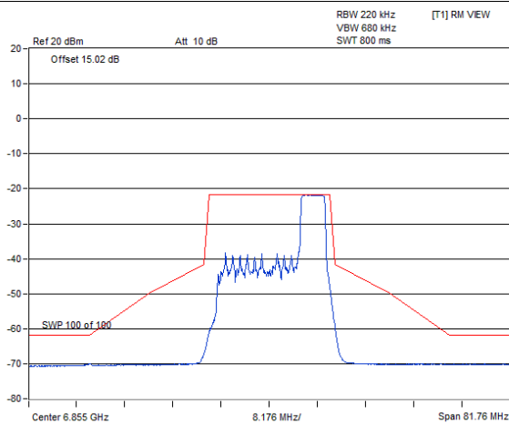
802.11ax (HE20) 52-tone RU 1Tx / Chain 0 : CH 181@40
