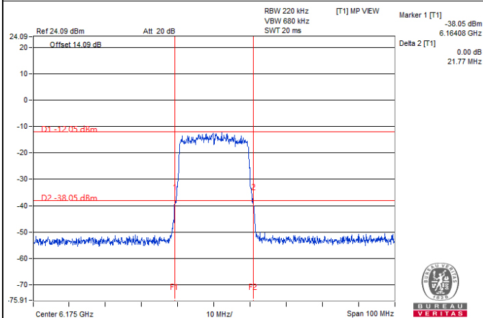
802.11ax (HE20) CDD-2Tx / Chain 0 : CH 45
