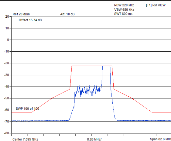
802.11ax (HE20) 52-tone RU 1Tx / Chain 0 : CH 229@40
