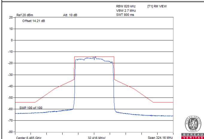
802.11ax (HE80) CDD-2Tx / Chain 1 : CH 103
