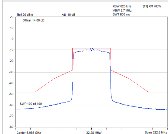
802.11ax (HE80) 1Tx / Chain 0 : CH 7
