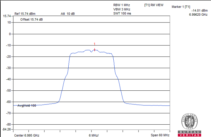
802.11a CDD-2Tx / Chain 1 : CH 209
