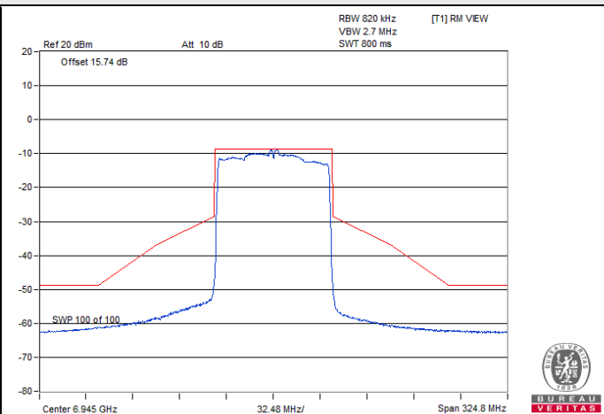
802.11ax (HE80) 1Tx / Chain 0 : CH 199
