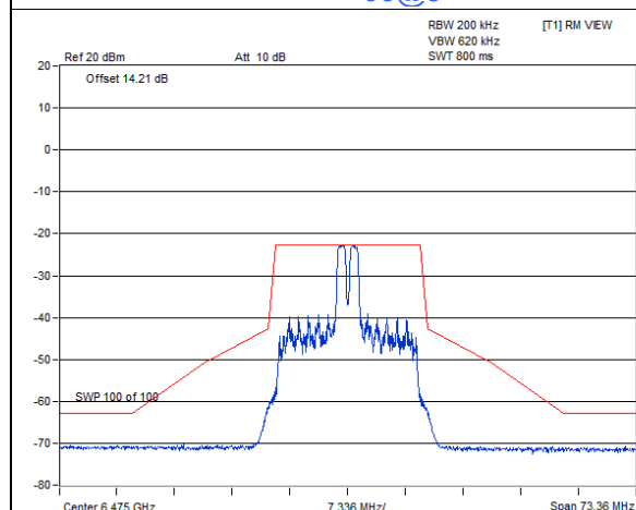
802.11ax (HE20) 26-tone RU CDD-2Tx / Chain 0 : CH 105@4
