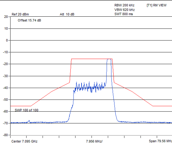
802.11ax (HE20) 26-tone RU 1Tx / Chain 0 : CH 229@8
