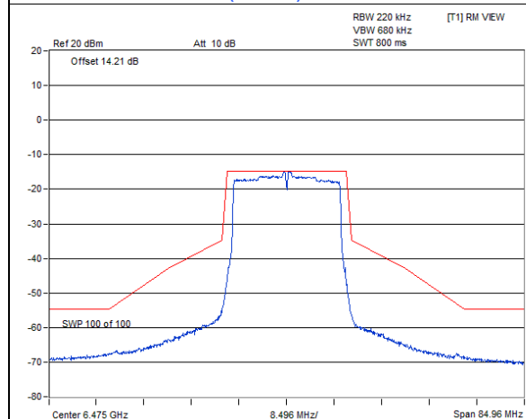
802.11ax (HE20) 1Tx / Chain 0 : CH 105
