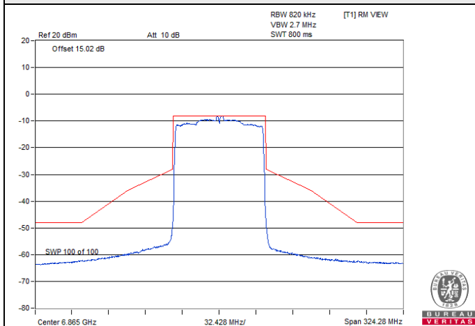
802.11ax (HE80) 1Tx / Chain 0 : CH 183
