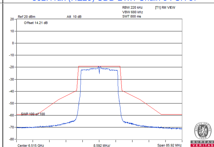
802.11ax (HE20) CDD-2Tx / Chain 0 : CH 113
