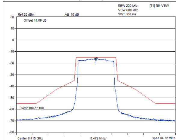
802.11ax (HE20) 1Tx / Chain 0 : CH 93
