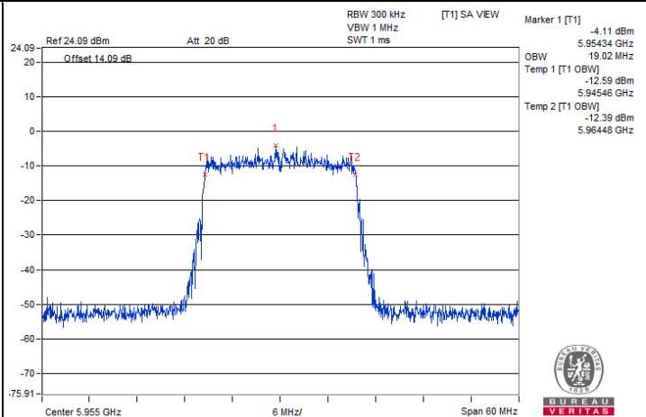
802.11ax (HE20) 1Tx / Chain 0 : CH 1
