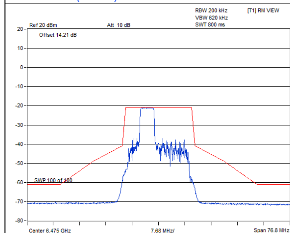
802.11ax (HE20) 52-tone RU 1Tx / Chain 0 : CH 105@38
