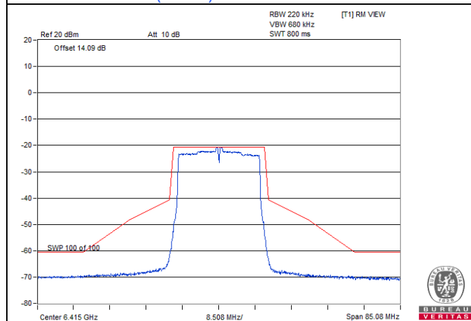
802.11ax (HE20) CDD-2Tx / Chain 0 : CH 93
