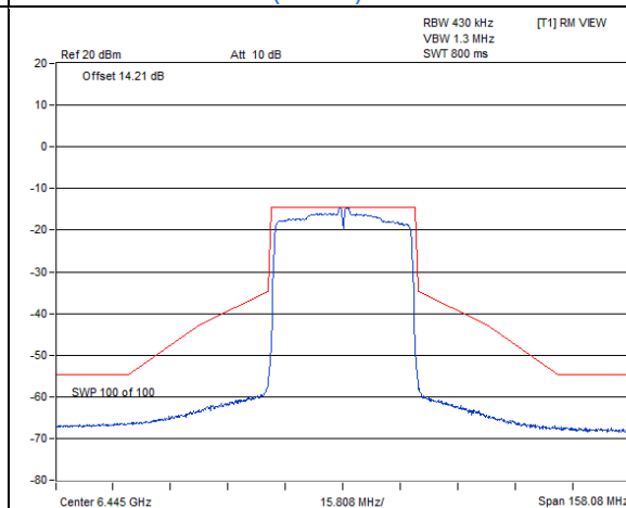
802.11ax (HE40) 1Tx / Chain 0 : CH 99
