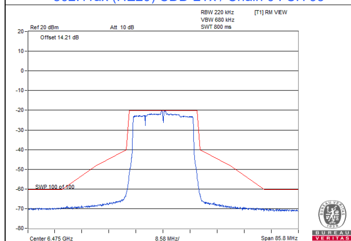
802.11ax (HE20) CDD-2Tx / Chain 0 : CH 105
