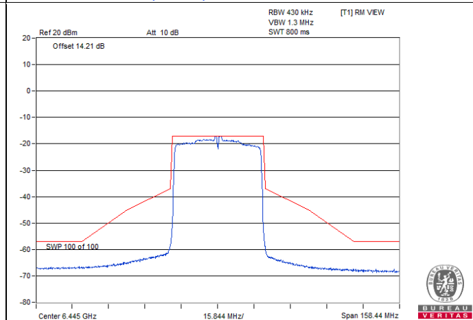
802.11ax (HE40) CDD-2Tx / Chain 1 : CH 99
