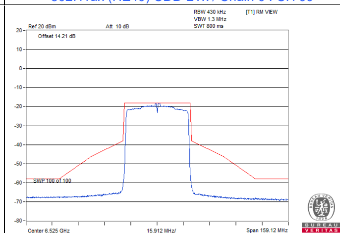
802.11ax (HE40) CDD-2Tx / Chain 0 : CH 115
