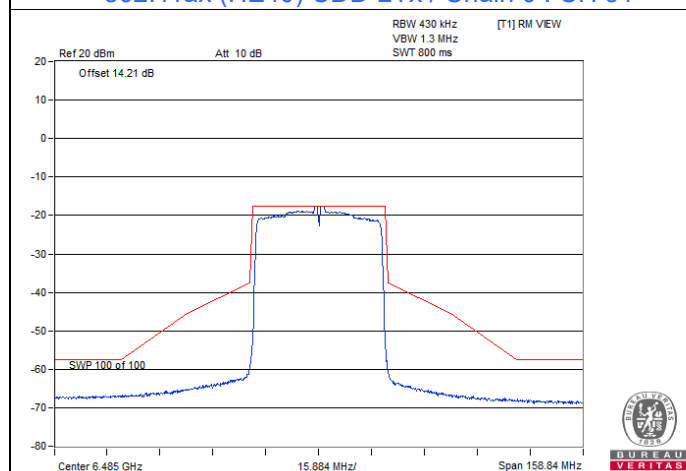
802.11ax (HE40) CDD-2Tx / Chain 0 : CH 107
