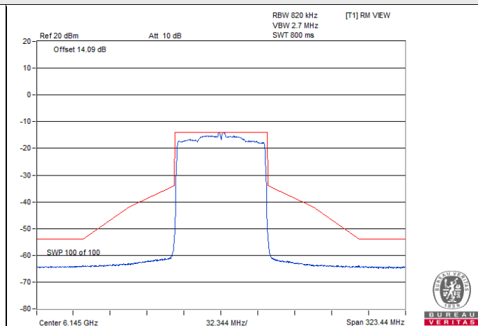
802.11ax (HE80) CDD-2Tx / Chain 0 : CH 39
