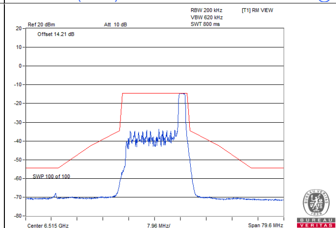
802.11ax (HE20) 26-tone RU 1Tx / Chain 0 : CH 113@8
