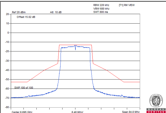
802.11ax (HE20) 1Tx / Chain 0 : CH 149
