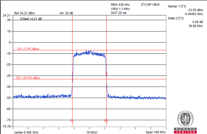
802.11ax (HE40) CDD-2Tx / Chain 1 : CH 107
