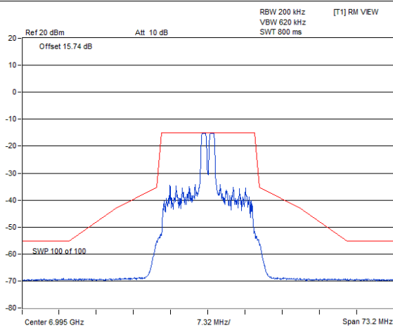
802.11ax (HE20) 26-tone RU 1Tx / Chain 0 : CH 209@4
