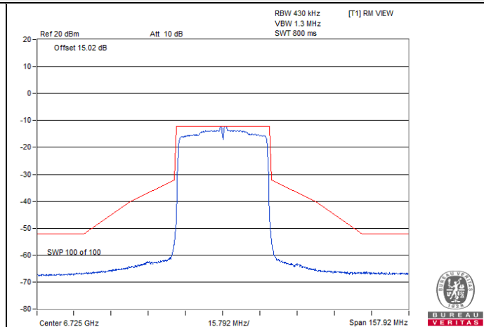
802.11ax (HE40) 1Tx / Chain 0 : CH 155
