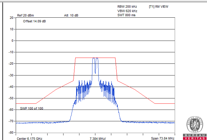
802.11ax (HE20) 26-tone RU 1Tx / Chain 0 : CH 45@4
