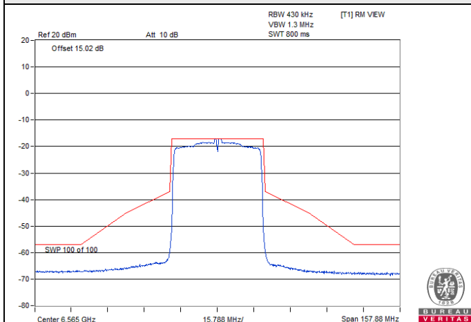
802.11ax (HE40) CDD-2Tx / Chain 0 : CH 123
