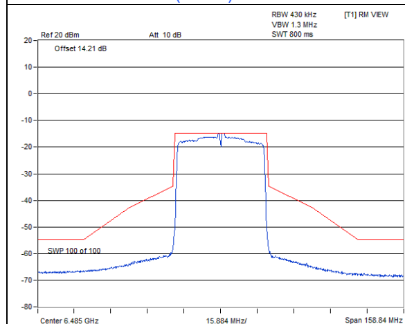
802.11ax (HE40) 1Tx / Chain 0 : CH 107
