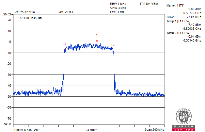
802.11ax (HE80) 1Tx / Chain 0 : CH 119
