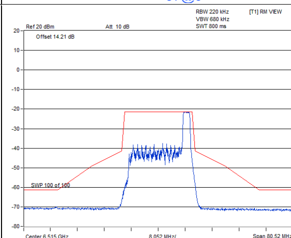
802.11ax (HE20) 26-tone RU CDD-2Tx / Chain 0 : CH 113@8
