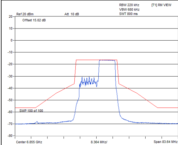
802.11ax (HE20) 106-tone RU 1Tx / Chain 0 : CH 181@54
