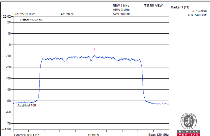
802.11ax (HE80) 1Tx / Chain 0 : CH 183
