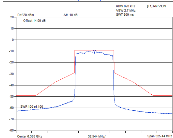
802.11ax (HE80) 1Tx / Chain 0 : CH 87
