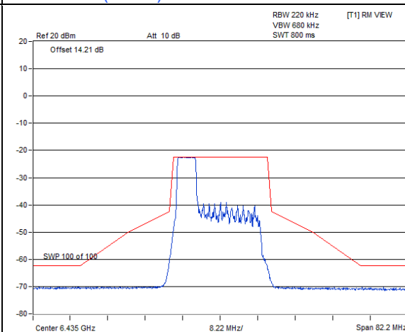
802.11ax (HE20) 52-tone RU 1Tx / Chain 0 : CH 97@37
