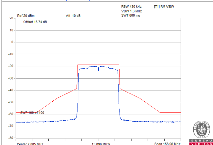
802.11ax (HE40) CDD-2Tx / Chain 0 : CH 211
