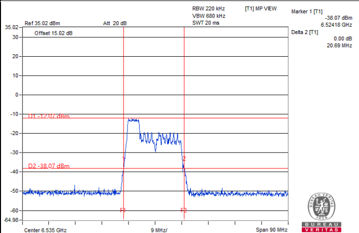
802.11ax (HE20) 52-tone RU 1Tx : CH 117@37
