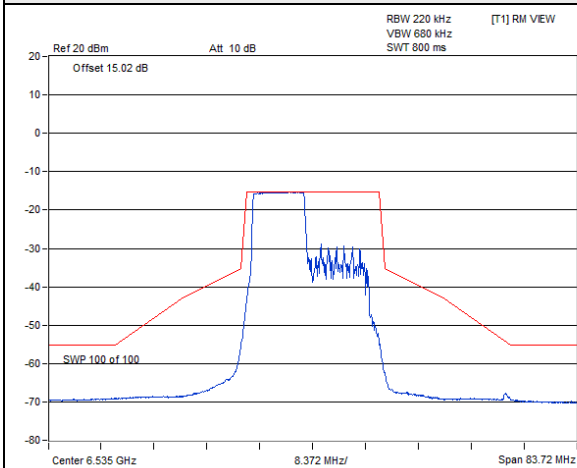
802.11ax (HE20) 106-tone RU 1Tx / Chain 0 : CH 117@53
