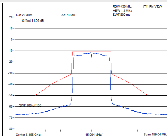
802.11ax (HE40) 1Tx / Chain 0 : CH 43
