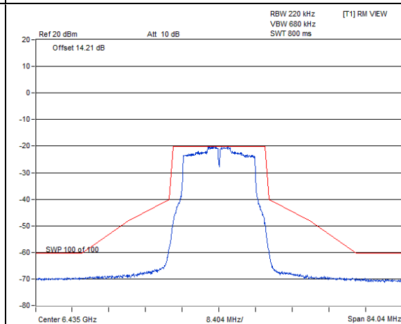
802.11a CDD-2Tx / Chain 0 : CH 97
