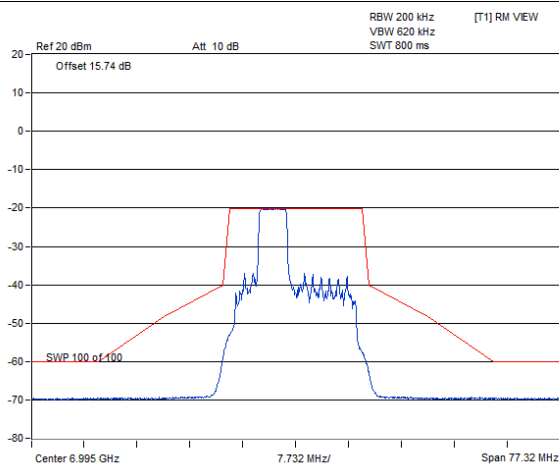
802.11ax (HE20) 52-tone RU 1Tx / Chain 0 : CH 209@38
