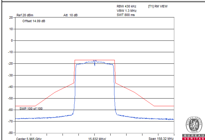
802.11ax (HE40) CDD-2Tx / Chain 1 : CH 3
