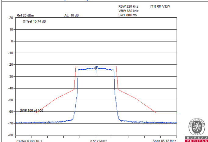
802.11ax (HE20) CDD-2Tx / Chain 0 : CH 209
