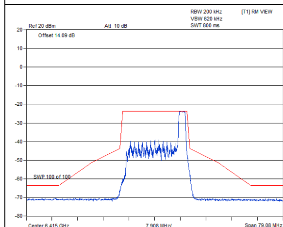
802.11ax (HE20) 26-tone RU CDD-2Tx / Chain 0 : CH 93@8
