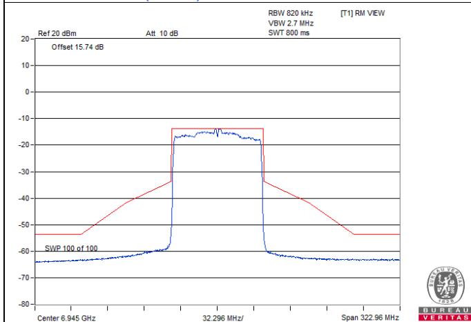
802.11ax (HE80) CDD-2Tx / Chain 1 : CH 199
