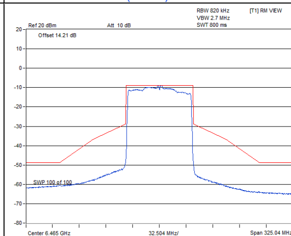
802.11ax (HE80) 1Tx / Chain 0 : CH 103
