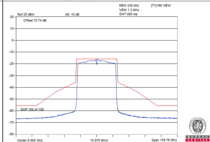
802.11ax (HE40) CDD-2Tx / Chain 1 : CH 187
