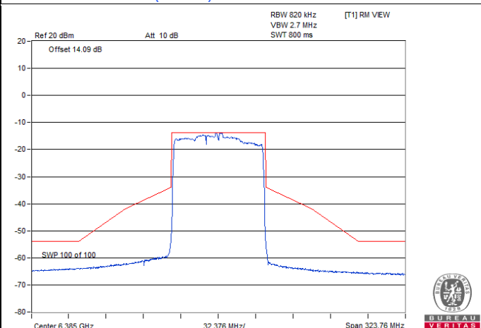
802.11ax (HE80) CDD-2Tx / Chain 1 : CH 87
