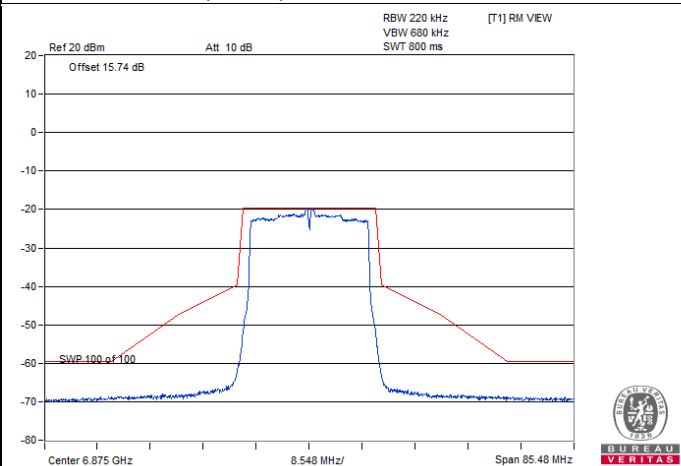
802.11ax (HE20) CDD-2Tx / Chain 0 : CH 185
