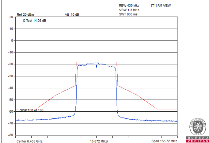
802.11ax (HE40) CDD-2Tx / Chain 1 : CH 91
