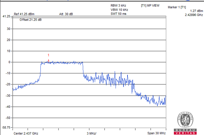
802.11ax (HE20) 106-tone RU 1Tx / Chain 0 : CH 6@53
