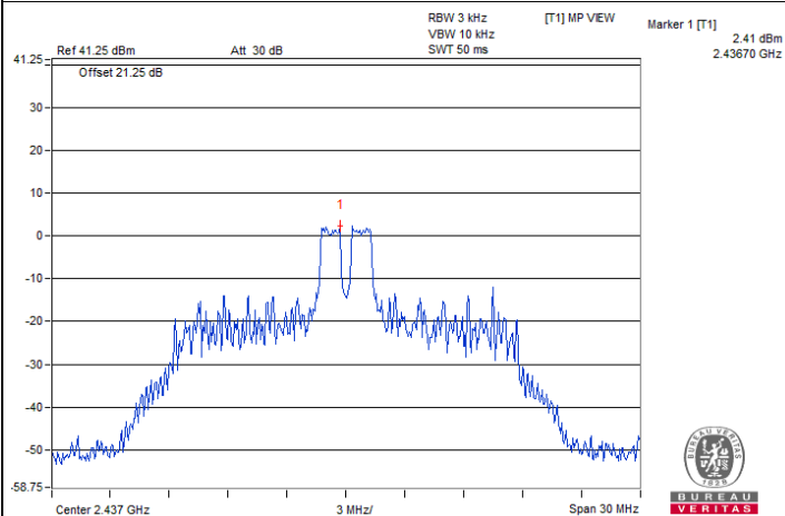
802.11ax (HE20) 26-tone RU CDD-2Tx / Chain 0 : CH 6@4
