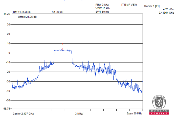
802.11ax (HE20) 52-tone RU 1Tx / Chain 0 : CH 6@38
