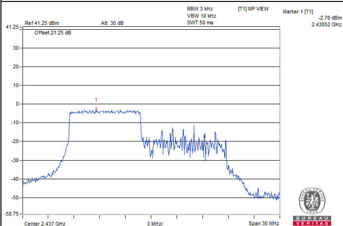
802.11ax (HE20) 106-tone RU CDD-2Tx / Chain 0 : CH 6@53
