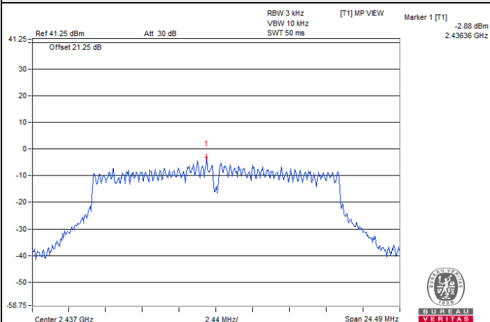
802.11g CDD-2Tx / Chain 1 : CH 6
