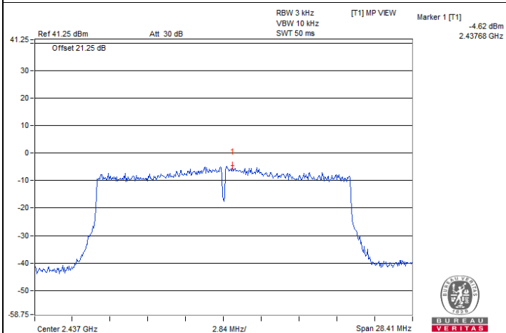
802.11ax (HE20) 1Tx / Chain 0 : CH 6
