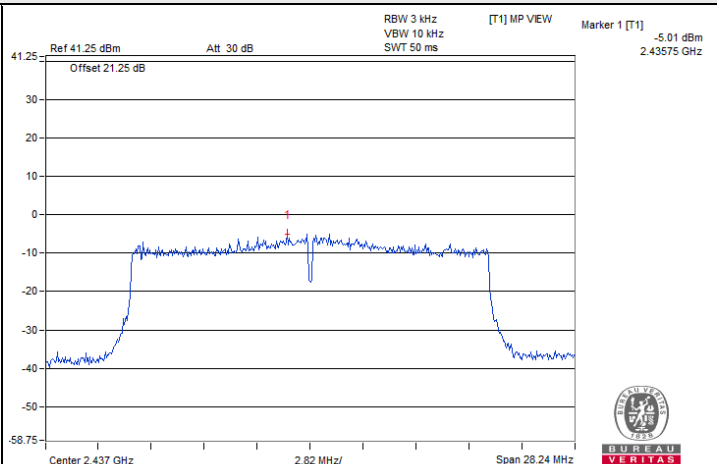
802.11ax (HE20) CDD-2Tx / Chain 1 : CH 6
