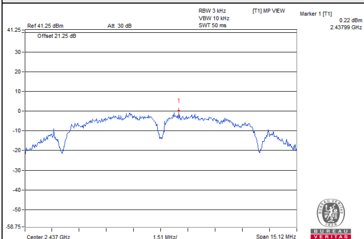
802.11b 1Tx / Chain 0 : CH 6
