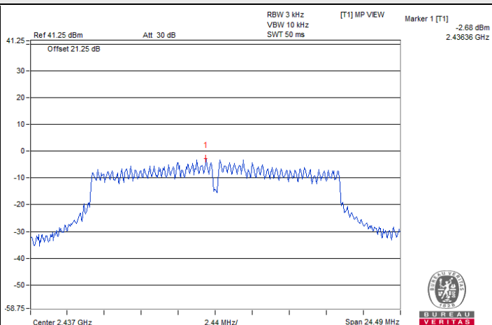
802.11g 1Tx / Chain 0 : CH 6
