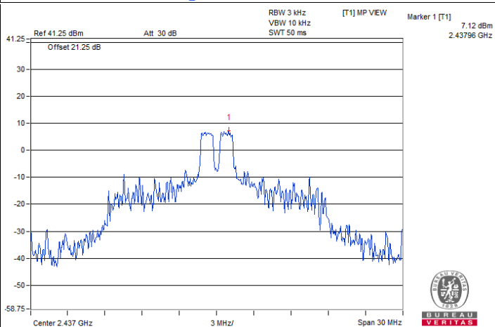
802.11ax (HE20) 26-tone RU 1Tx / Chain 0 : CH 6@4
