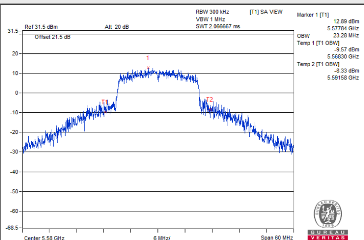
802.11ac (VHT20) : CH 116
