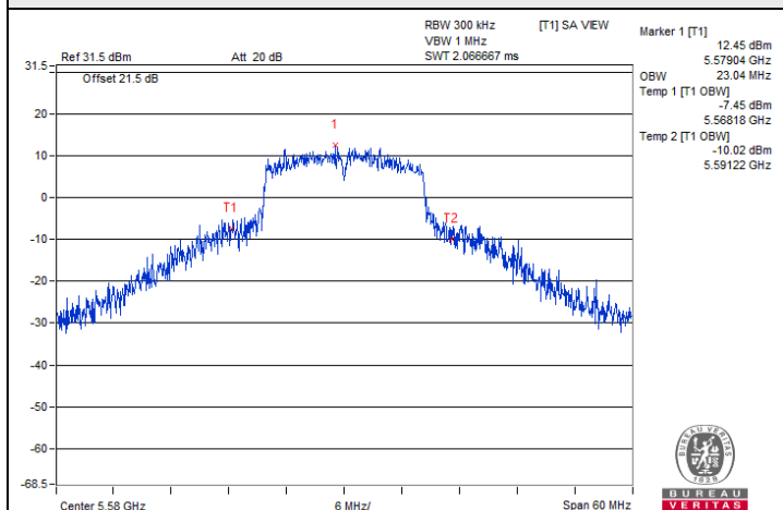
802.11a : CH 116
