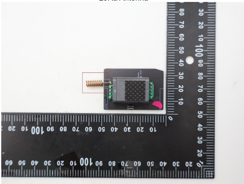
LoRa Antenna
