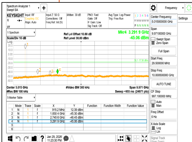
LoRa SF10 125kHz 915.2MHz
