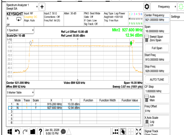
Lora_SF12_125kHz 915.2-927.6
