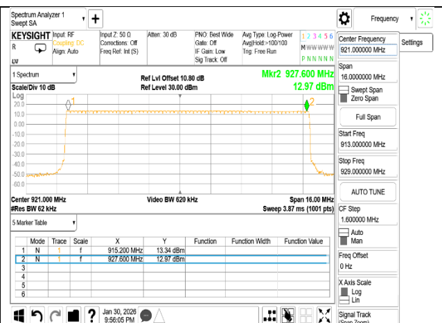
Lora_SF11_125kHz 915.2-927.6
