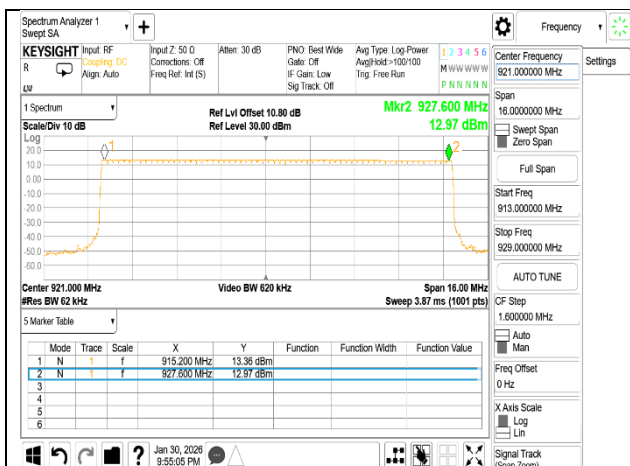
Lora_SF10_125kHz 915.2-927.6
