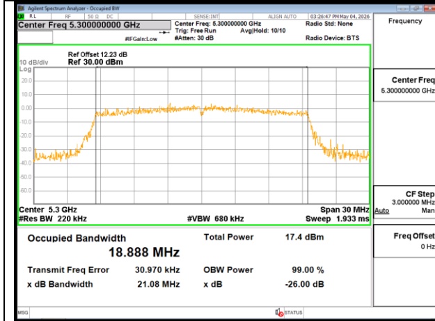
802.11ax 20MHz Chain0 5300MHz
