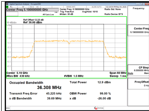
802.11n_40MHz_Chain0_5190MHz
