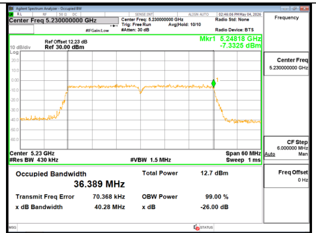
802.11n_40MHz_Chain0_5230MHz
