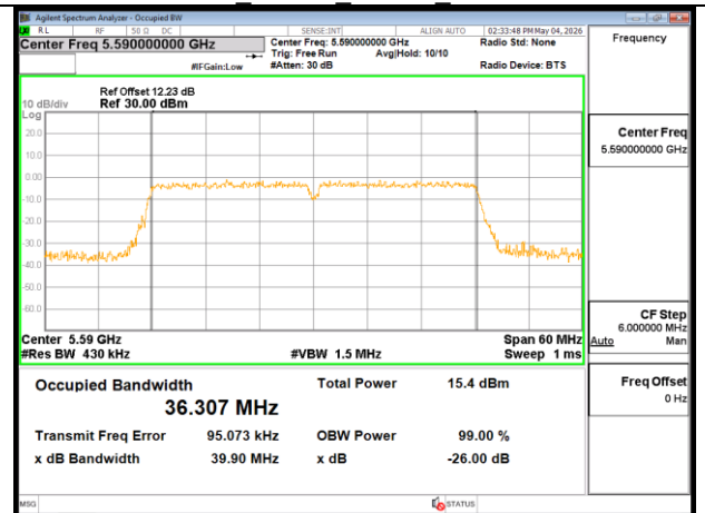
802.11n_40MHz_Chain0_5590MHz
