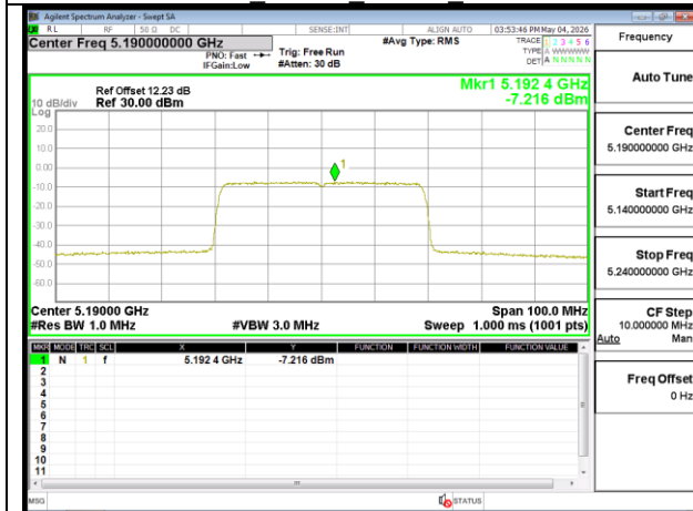
802.11ax 40MHz Chain0 5190MHz
