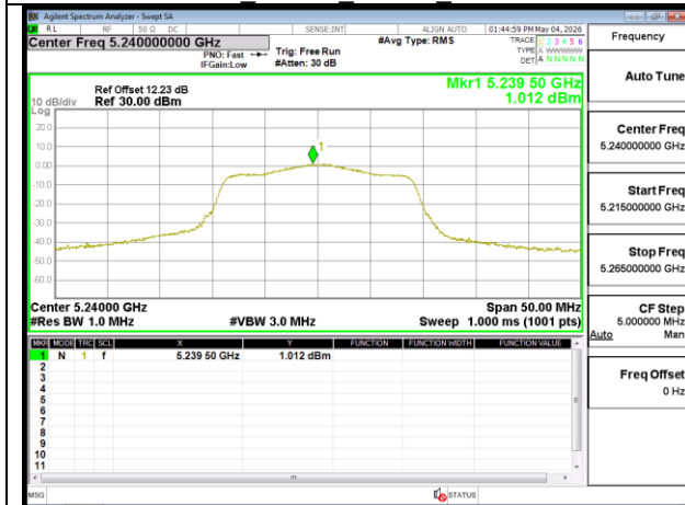
802.11n 20MHz Chain0 5240MHz
