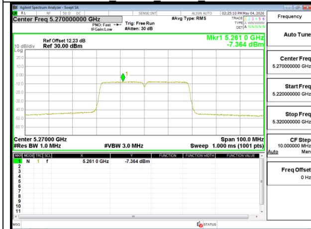
802.11n 40MHz Chain0 5270MHz
