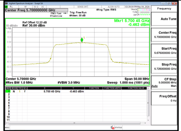
802.11ax 20MHz Chain1 5700MHz
