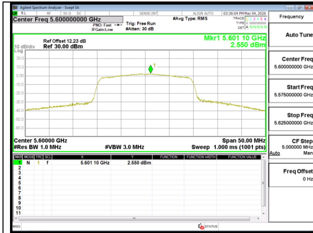
802.11ax 20MHz Chain0 5600MHz
