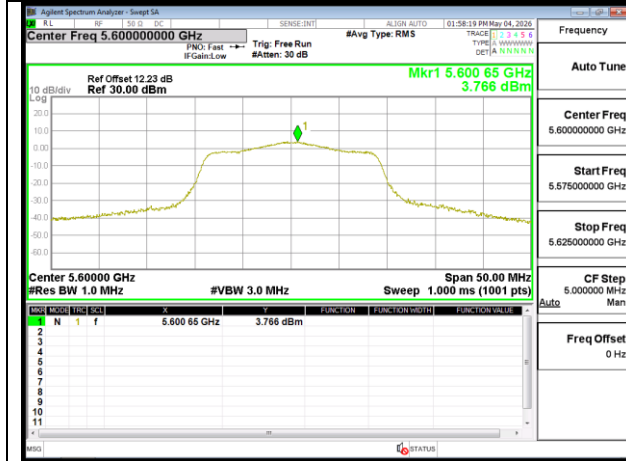
802.11n 20MHz Chain0 5600MHz
