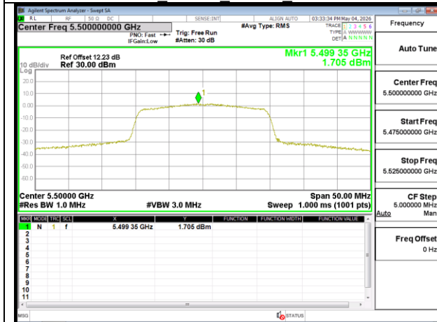
802.11ax 20MHz Chain0 5500MHz
