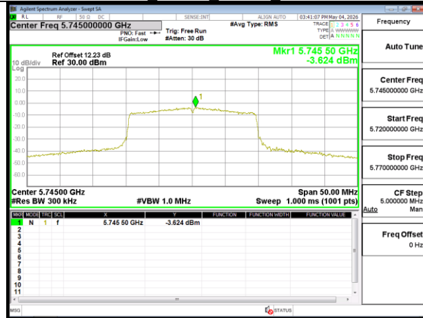
802.11ax 20MHz Chain0 5745MHz
