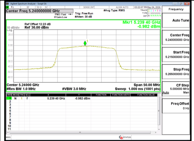
802.11ax 20MHz Chain1 5240MHz
