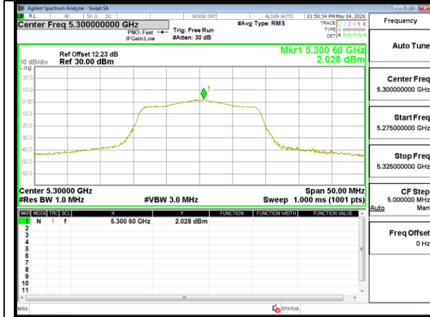
802.11n 20MHz Chain0 5300MHz
