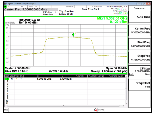
802.11ax 20MHz Chain1 5300MHz
