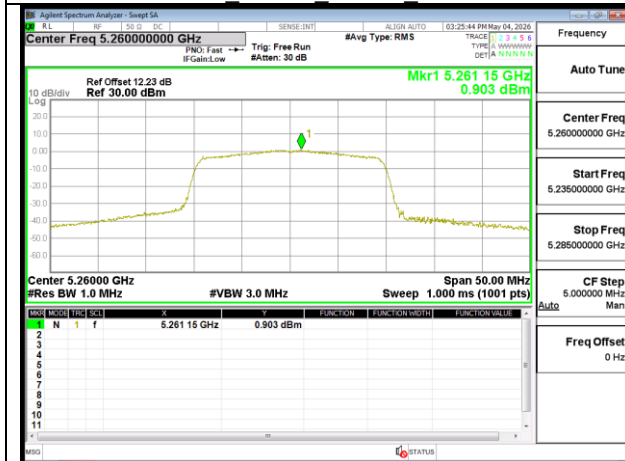
802.11ax 20MHz Chain0 5260MHz
