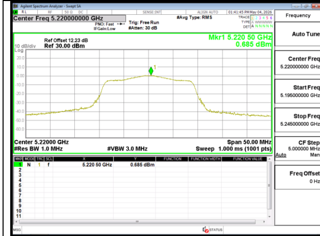
802.11n 20MHz Chain0 5220MHz
