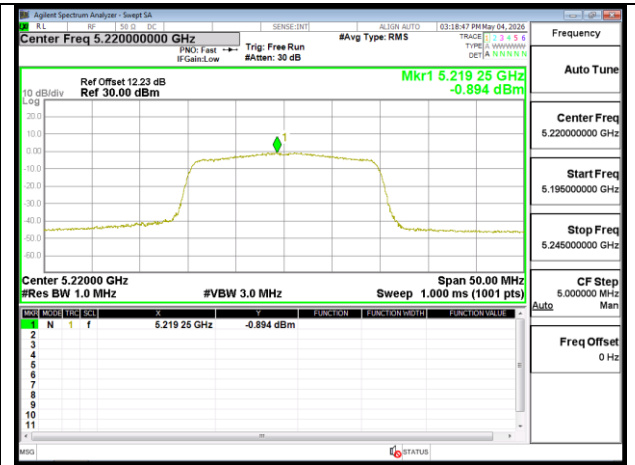
802.11ax 20MHz Chain1 5220MHz
