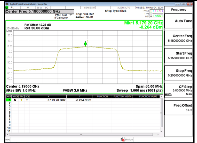
802.11ax 20MHz Chain1 5180MHz
