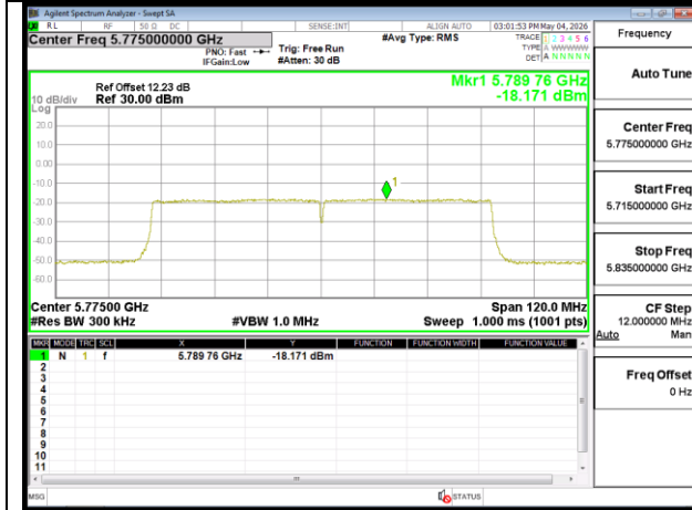
802.11ac 80MHz Chain0 5775MHz
