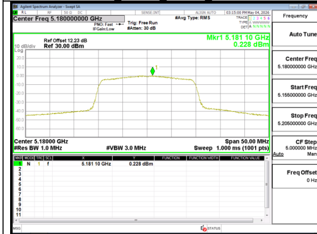
802.11ax 20MHz Chain0 5180MHz
