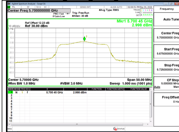
802.11n 20MHz Chain0 5700MHz
