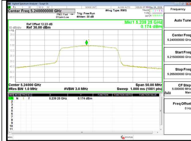
802.11ax 20MHz Chain0 5240MHz
