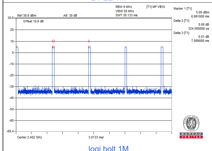
BT-LE 1M
