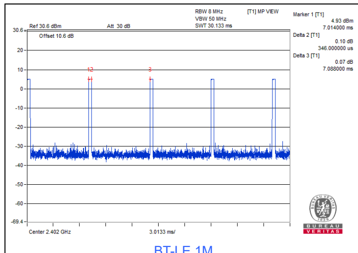
BT-LE 1M
