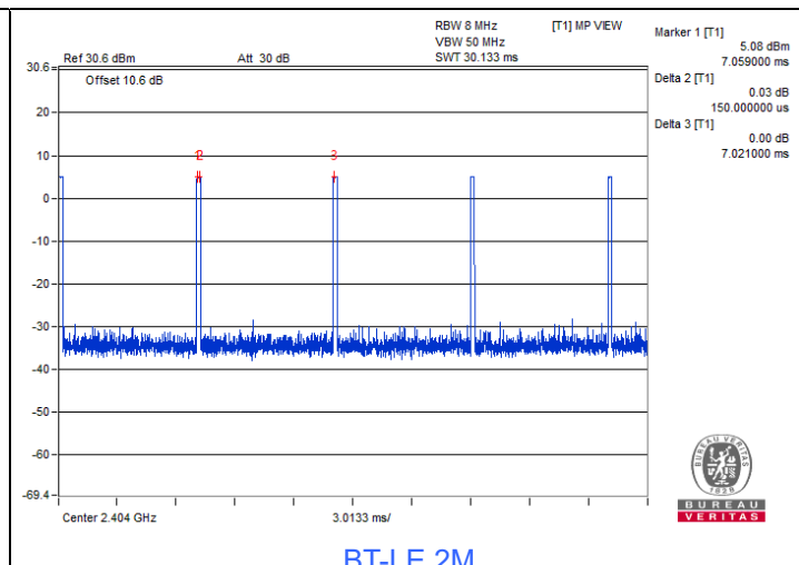
BT-LE 2M
