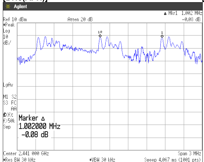
[DH5(AFH)]
