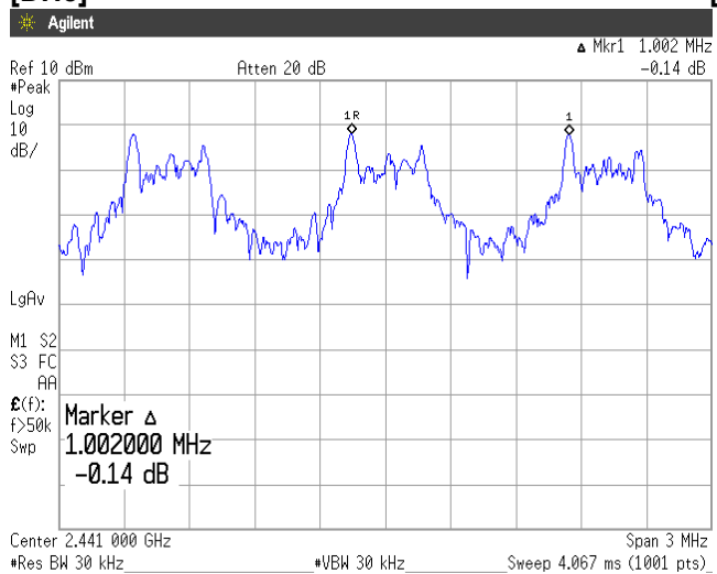
[DH5(AFH)]
