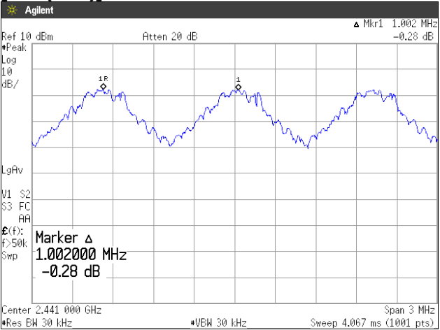
[DH5(AFH)]
