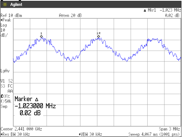
[DH5]
